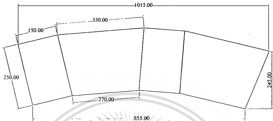
ภาพที่ 191 ภาพคลี่กระดาษ
