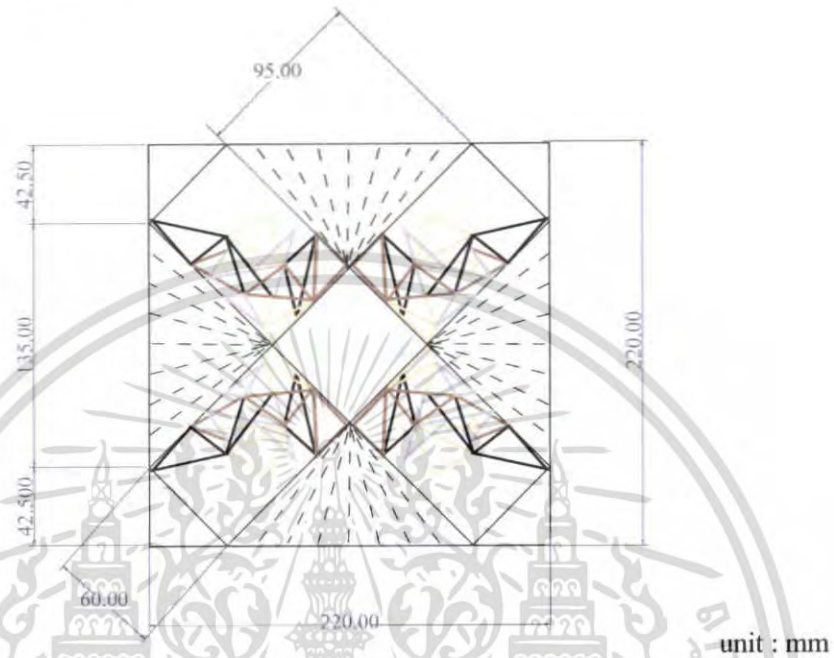
ภาพที่ 161 ขนาดตัดส่วนผลิตภัณฑ์ก่อนพับ
