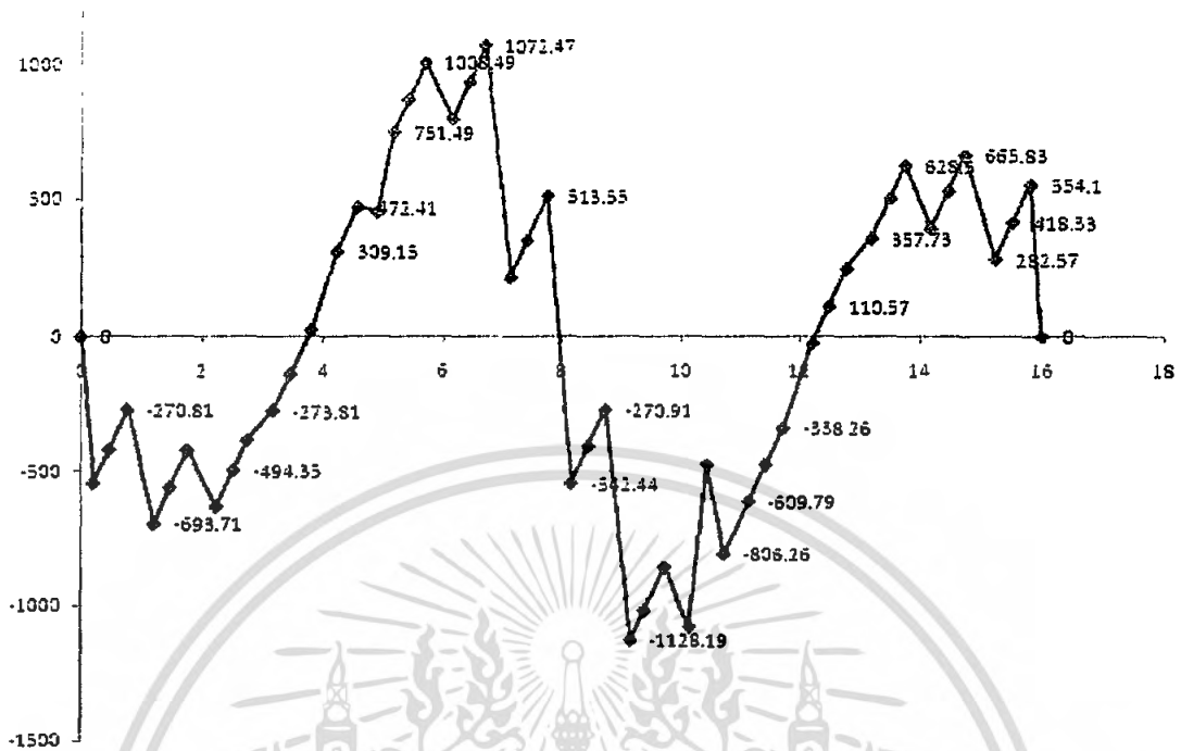
รูปที่ 4.35 ค่า Shear Force Diagram ที่หน้าตัด B-B ในโครงสร้าง Flat Slab
