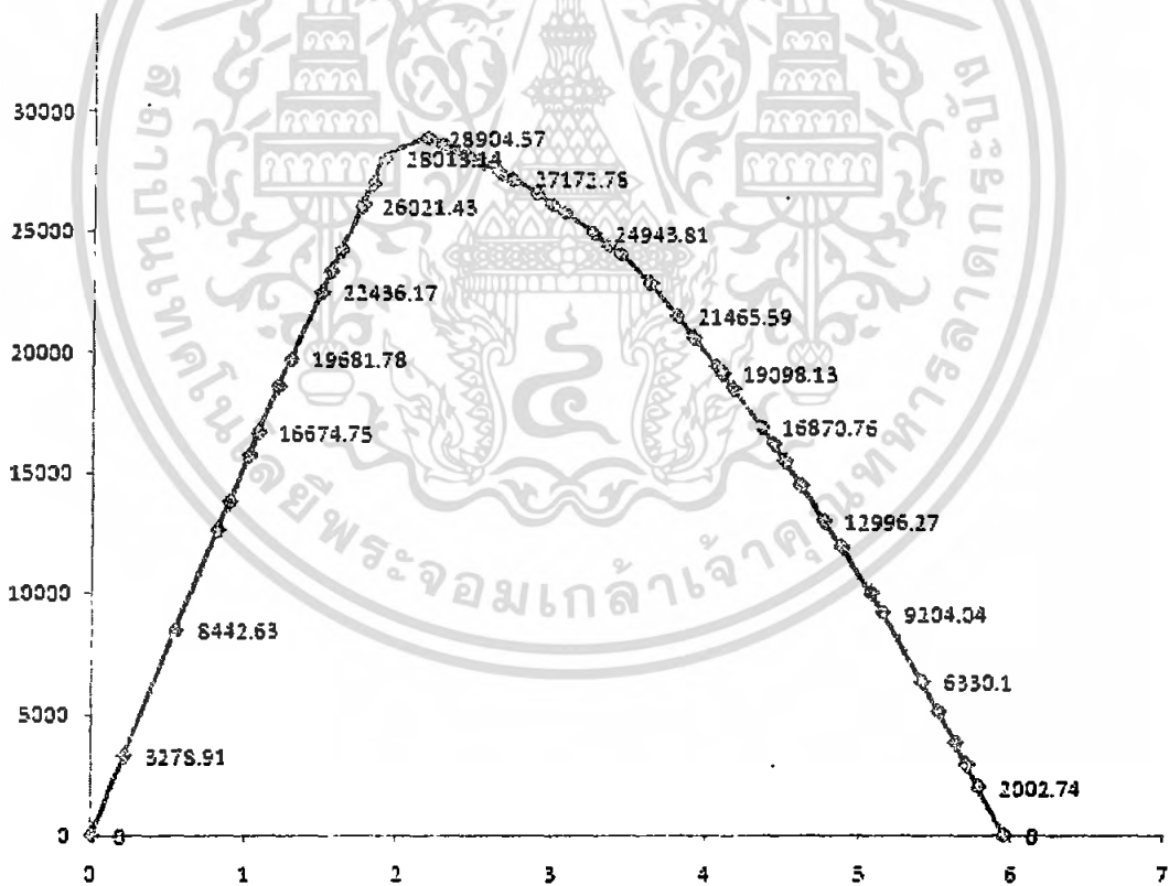
รูปที่ 4.96 Bending Moment Diagram เฉพาะคานที่ Critical ชั้นสอง (1)
