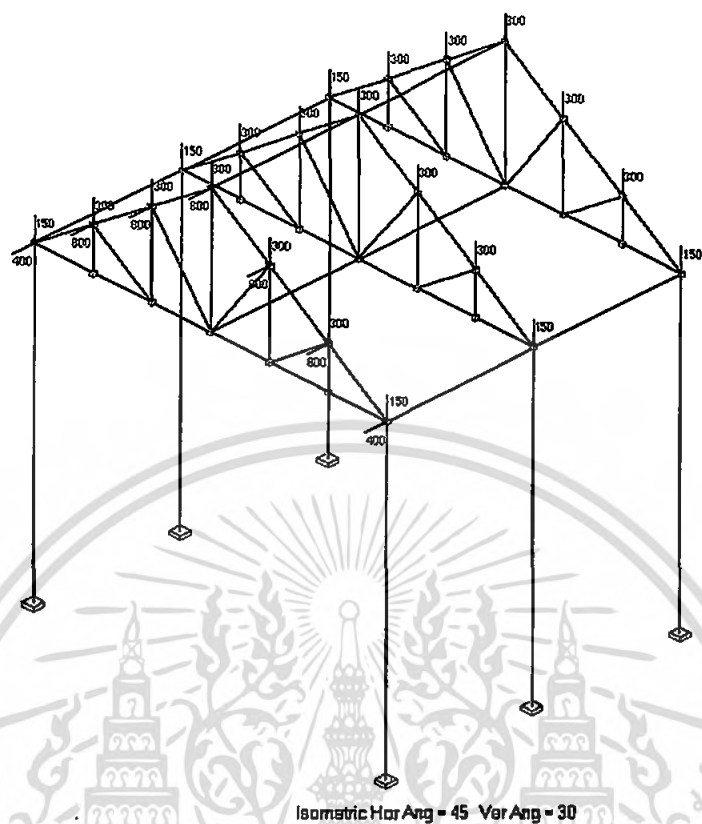
รูปที่ 4.17 โครงสร้าง Truss พร้อมแรงที่กระทำต่อโครงสร้าง
