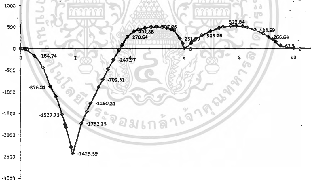
รูปที่ 4.5 ค่า Bending Moment Diagram ในคานของโครงสร้างช่วงเดียวและคานต่อเนื่อง
