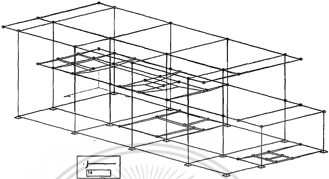
รูปที่ 4.91 การแอนเนนในโครงสร้าง บ้านพักอาศัยสองชั้นเมื่อใช้ Over Scale 14 เท่า
