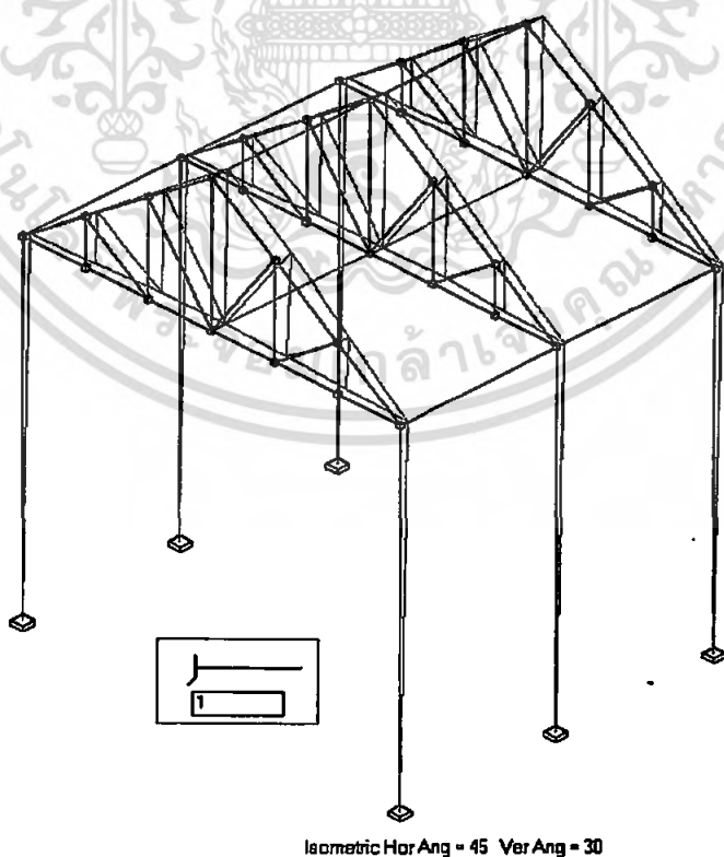
รูปที่ 4.18 การอ่อนเอนในโครงสร้าง Truss เมื่อใช้ Over Scale 1 เท่า
