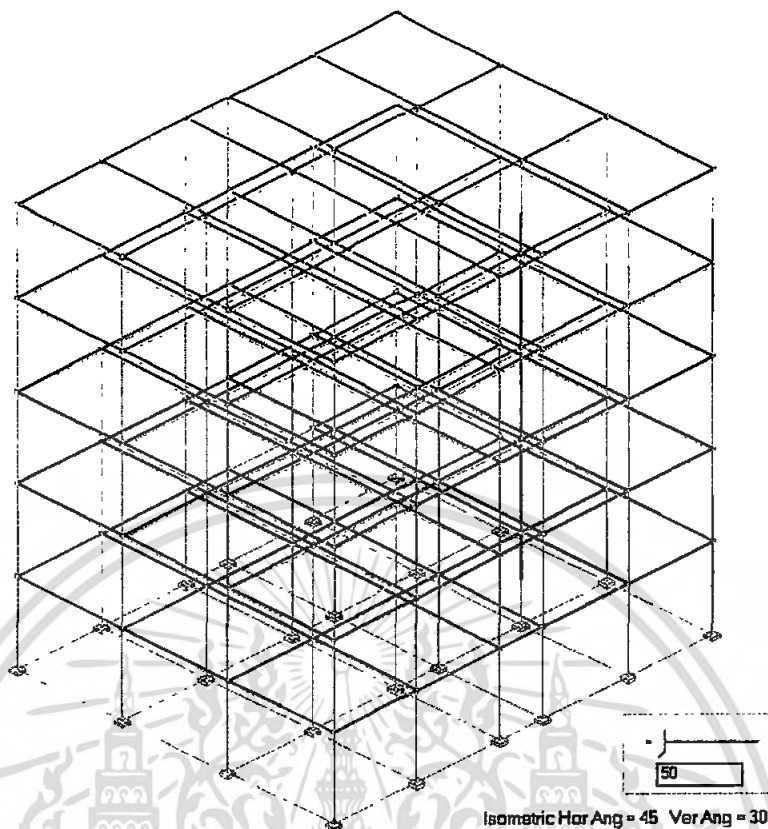
รูปที่ 4.114 การแอนไอโซเมตริกในโครงสร้างอาคารพักอาศัยหกชั้นเมื่อใช้ Over Scale 50 เท่า
