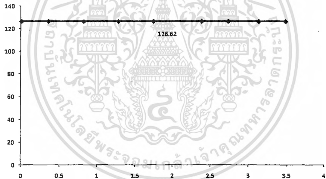
รูปที่ 4.11 ค่า Shear Force Diagram ในเสา (2) ของโครงสร้างช่วงเดียวและคานต่อเนื่อง
