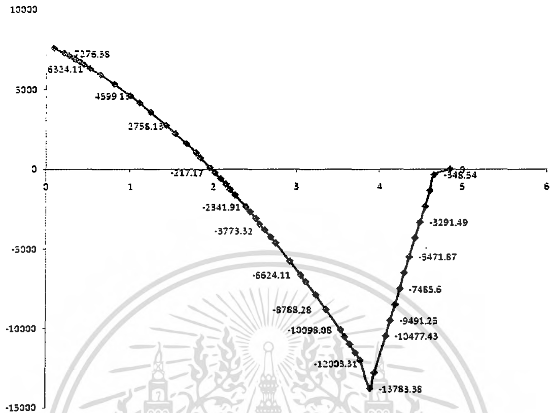
รูปที่ 4.97 Bending Moment Diagram เฉพาะคานที่ Critical ชั้นสอง (2)
