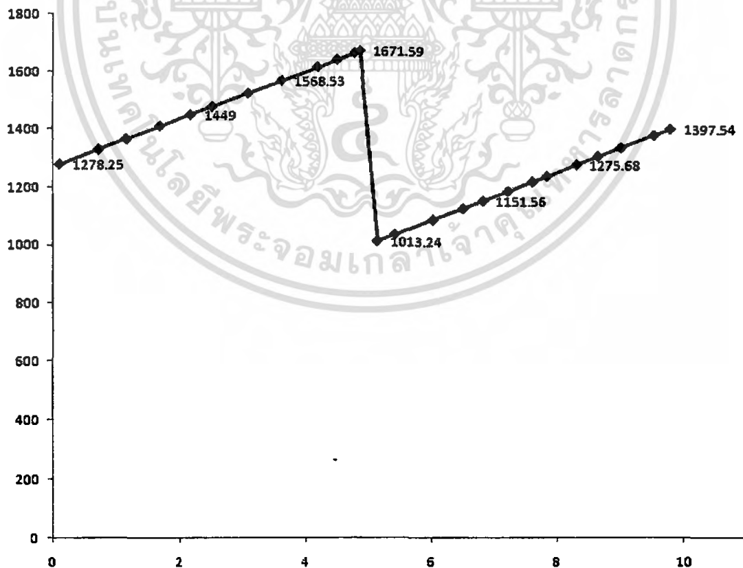
รูปที่ 4.22 ค่า Shear Force Diagram ในคานโครงสร้าง Truss
