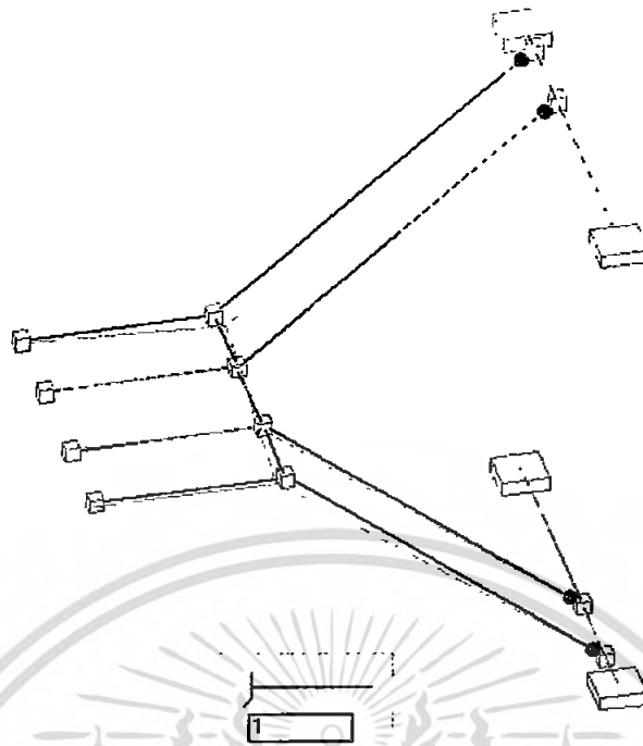
รูปที่ 4.61 การอ่านเอนในโครงสร้าง Dog Leg Stair เมื่อใช้ Over Scale 1 เท่า (ภาพสามมิติ) (3)
