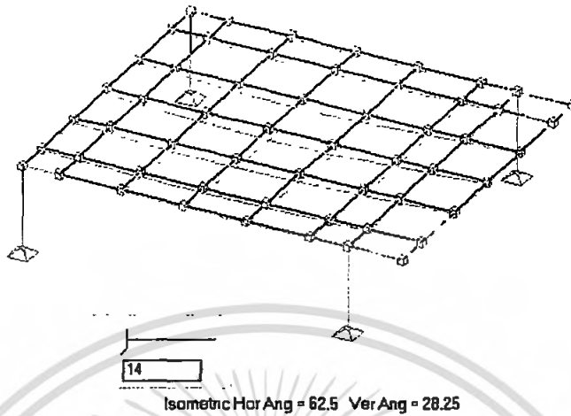
รูปที่ 4.82 การแอนเนนในโครงสร้างบ้านพักอาศัยสองชั้นส่วนที่จอดรถ เมื่อใช้ Over Scale 14 เท่า
