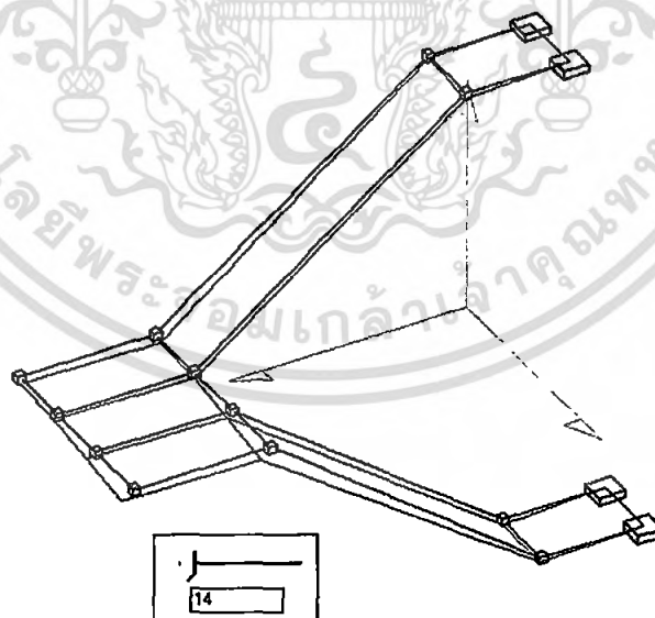
รูปที่ 4.76 การแอนะนในโครงสร้าง Dog Leg Stair เมื่อใช้ Over Scale 14 เท่า (ตัวอย่างที่ 1)
