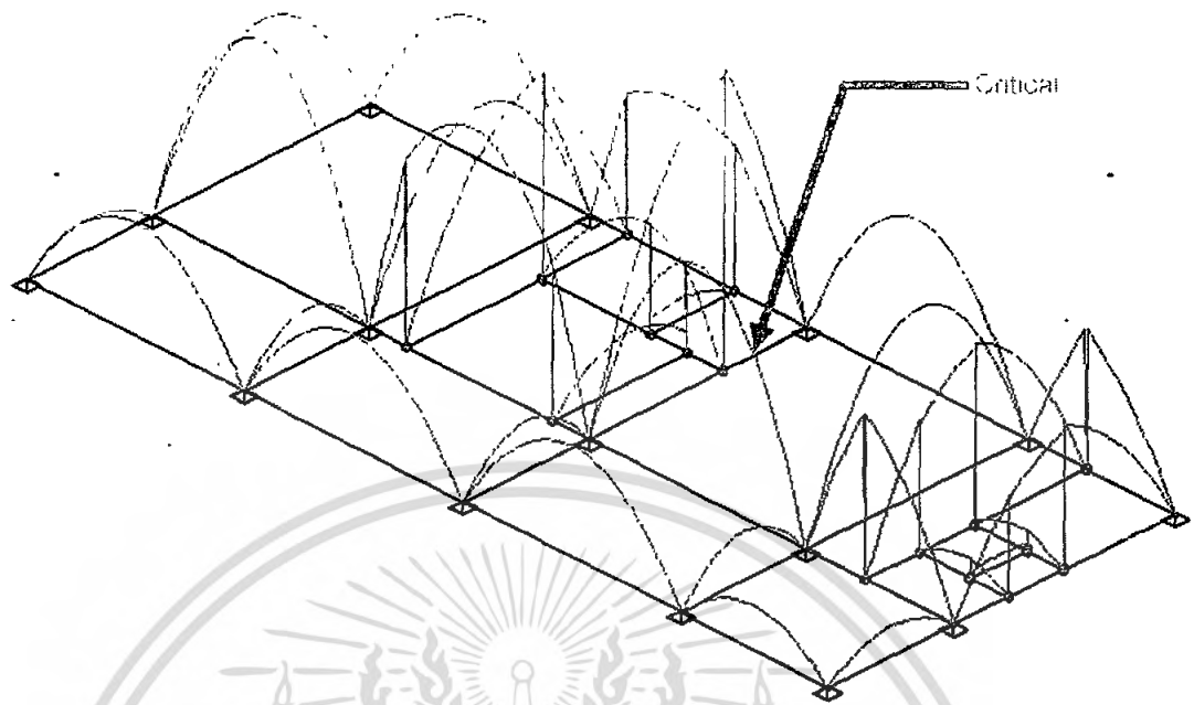
รูปที่ 4.93 Bending Moment Diagram เฉพาะชั้นล่าง
