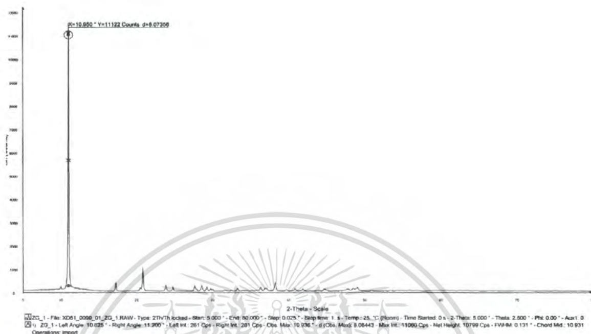
รูปที่ 4.7 สเปกตรัม XRD ของซิงค์กลีเซอโรเลตที่เตรียมจากกลีเซอรอลบริสุทธิ์กับ นาโนซิงค์ออกไซด์
