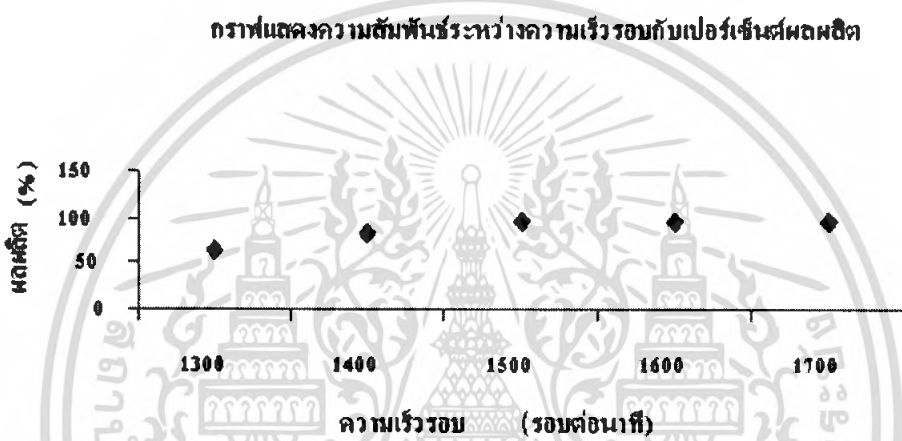
รูปที่ 4.2 ผลของความเร็วรอบในการปั่นกวนต่อการเตรียมซิงค์กลีเซอโรเลต
