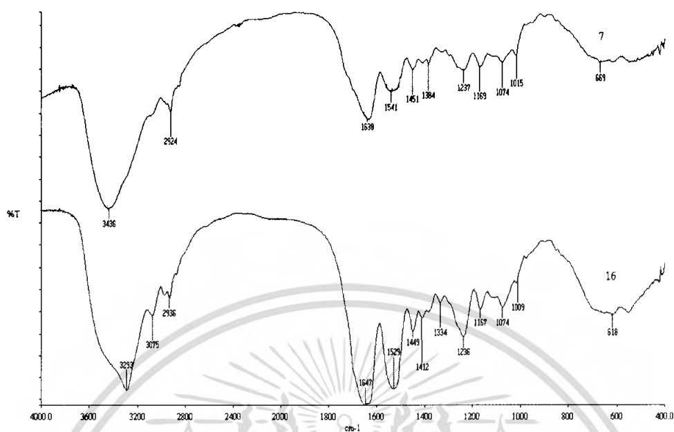
รูปที่ 7 แสดงการเปรียบเทียบของอินฟราเรดสเปกตรัม ของสูตรที่ 7 กับ 16
