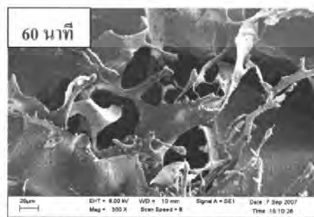
รูปที่ 4.59 แสดงสัณฐานวิทยาของไฟโบรอินที่ทำการต่อกิ่งแล้วของสูตรที่ 1-3 (น้ำไหม 30 mL
