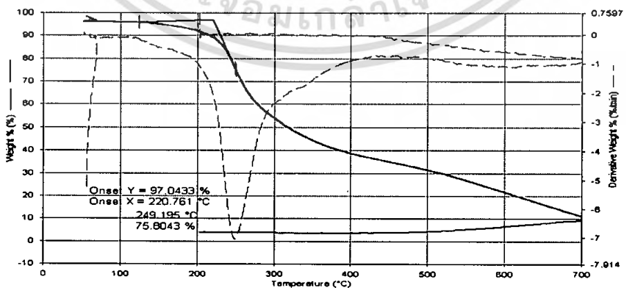
รูปที่ 4.41 เทอร์โมแกรมของสูตรที่ 12 (น้ำใหม่ 30 mL 2-HEMA 5 mL เวลา 60 นาที)
