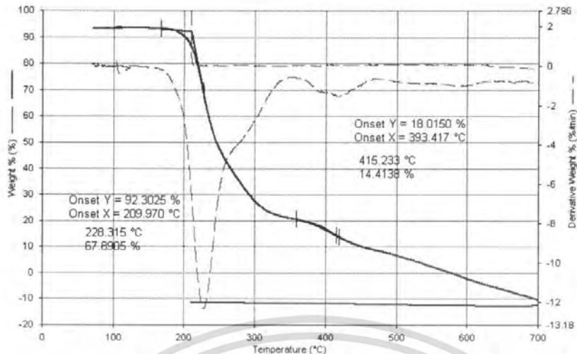
รูปที่ 4.49 เทอร์โมแกรมของพอลิไวนิลแอลกอฮอล์ (PVAl)
