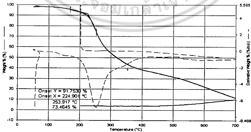
รูปที่ 4.47 เทอร์โมแกรมของสูตรที่ 18 (น้ำใหม่ 25 mL 2-HEMA 15 mL เวลา 15 นาที) เอกสารนี้เผยแพร่โดยศูนย์วิจัยและพัฒนาวัสดุพอลิเมอร์ มหาวิทยาลัยเทคโนโลยีพระจอมเกล้าเจ้าคุณทหารลาดกระบัง การค้า ไม่ว่ากรณีใดๆ ทั้งสิ้น อีกทั้งห้ามมิให้คัดแปลงเนื้อหา และต้องอ้างอิงถึงเจ้าของเอกสารทุกครั้งที่มีการนำไปใช้
