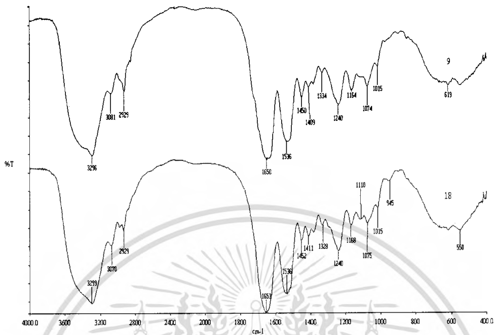
รูปที่ 9 แสดงการเปรียบเทียบของอินฟราเรดสเปกตรัม ของสูตรที่ 9 กับ 18
