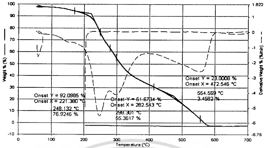
รูปที่ 4.45 เทอร์โมแกรมของสูตรที่ 16 (น้ำใหม่ 20 mL 2-HEMA 20 mL เวลา 15 นาที)
