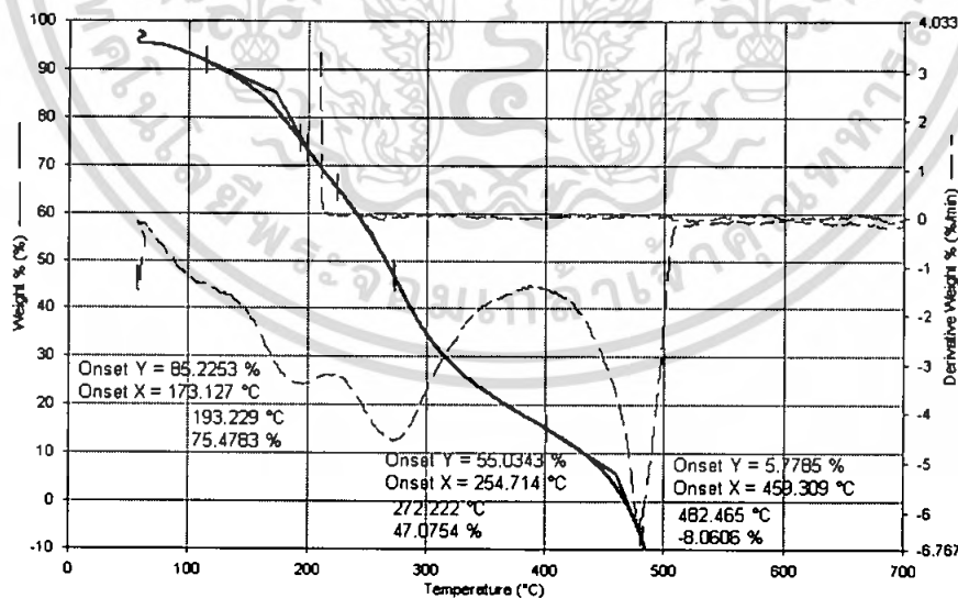
รูปที่ 4.56 เทอร์โมแกรมของสูตรที่ 24 (น้ำกลั่น 30 mL 2-HEMA 5 mL กลูตารัลดีไฮด์ 1 mL PVAI 4 mL เวลา 30 นาที)
