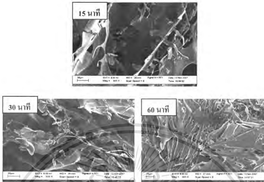
รูปที่ 4.64 แสดงสัณฐานวิทยาของไฟโบรินที่ทำการต่อกิ่งแล้วของสูตรที่ 16-18 (น้ำใหม่ 20 mL 2-HEMA 20 mL ที่เวลา 15 30 60 นาที ตามลำดับ) ที่กำลังขยาย 300 เท่า
