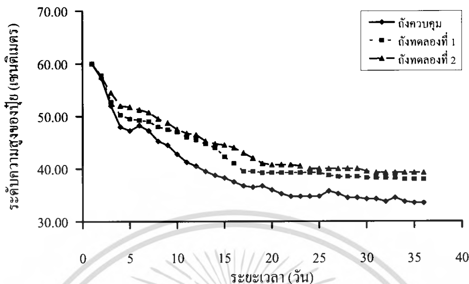
รูปที่ 4.1 อัตราการยุบตัวของกบฏในระหว่างการหมัก
