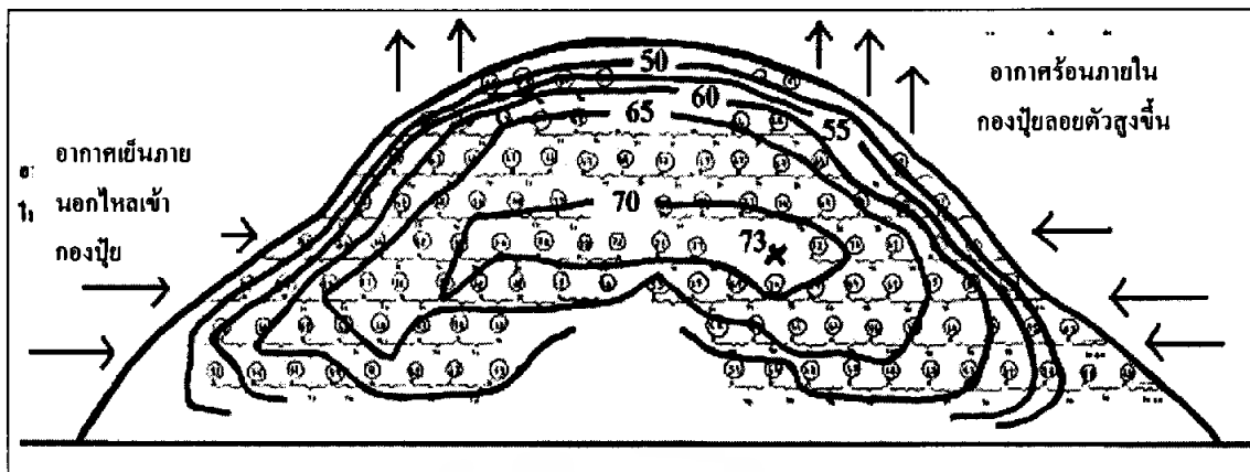
รูปที่ 2.3 ค่าอุณหภูมิในกองปุ๋ยอายุ 5 วัน และการแทนที่ของอากาศภายในกองปุ๋ย
