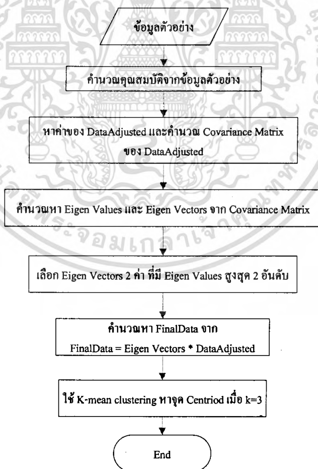
รูปที่ 2.12 การทำงานของการคำนวณหาไอแกนเวกเตอร์และไอแกนแวลูส์ของชุดข้อมูล
