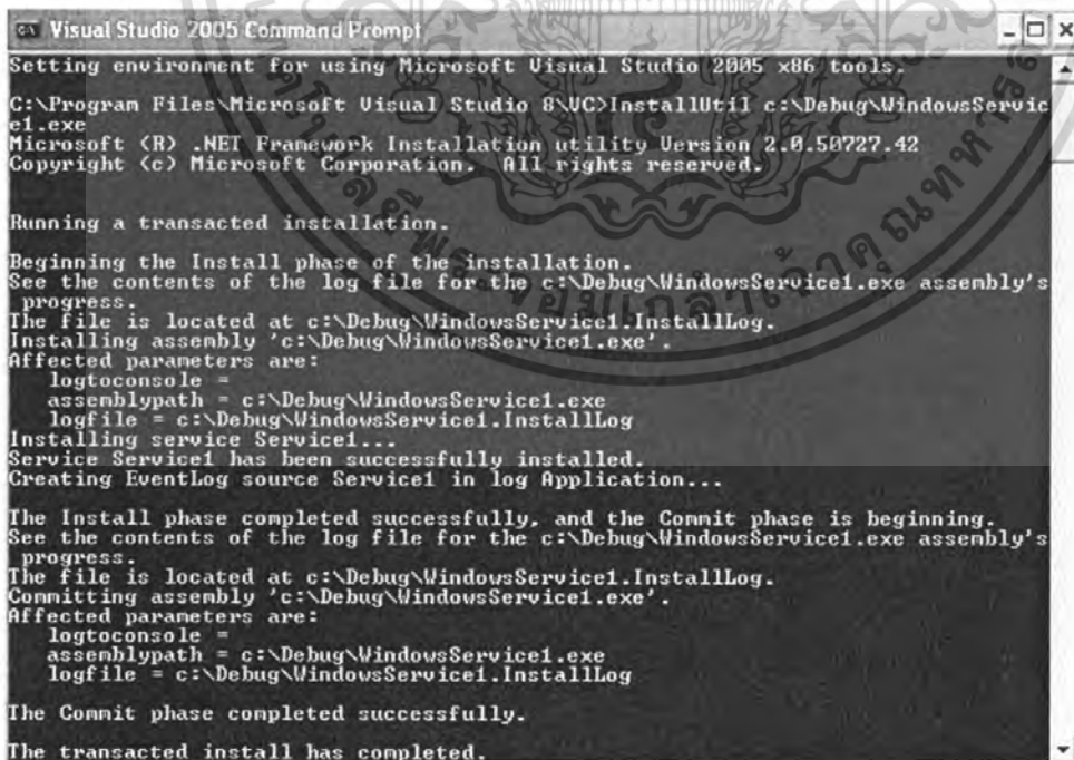
รูปที่ 5.8 ผลลัพธ์เมื่อทำการติดตั้งโปรแกรมวินโดวเซอร์วิสสำเร็จ
