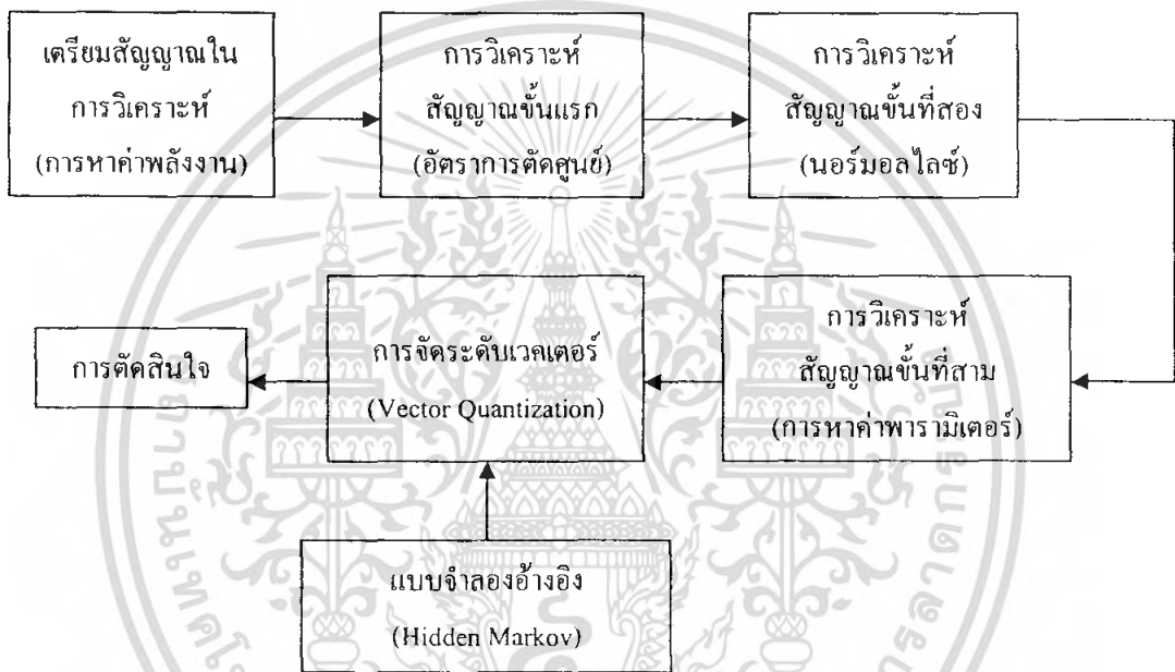
รูปที่ 3.1 บล็อก ไดอะแกรมขั้นตอนการตระหนักรู้เสียงพูด
