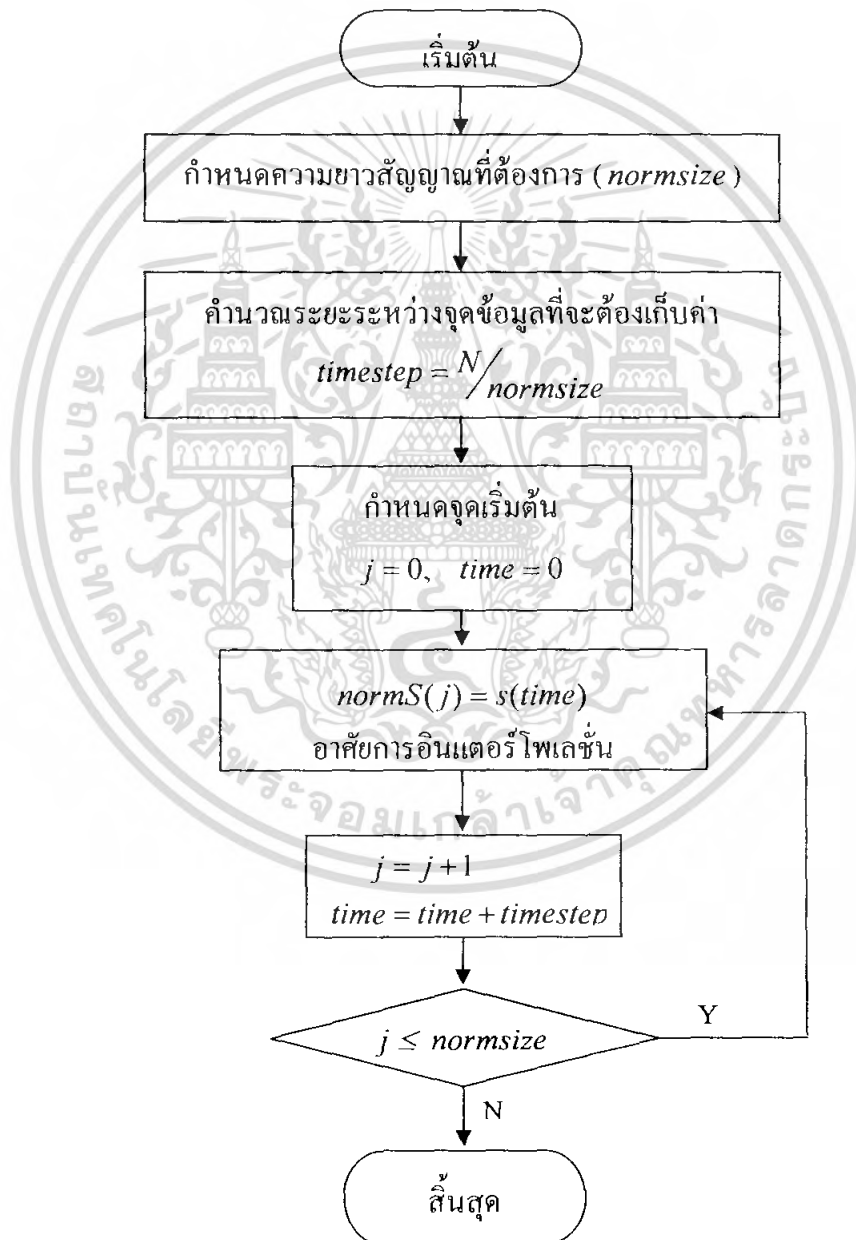
รูปที่ 3.4 ขั้นตอนการนอร์มอลไลซ์สัญญาณ
