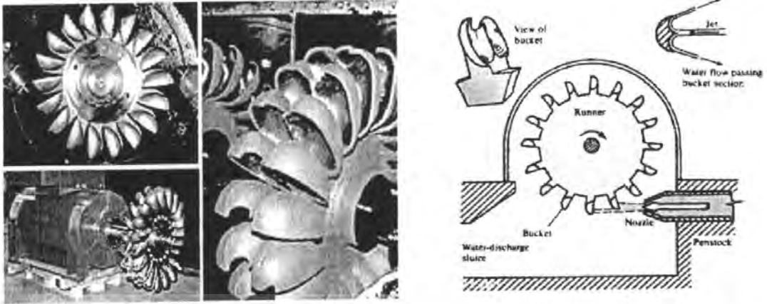
รูปที่ 3.8 แสดงตัวอย่างของกังหันน้ำเพลตัน
