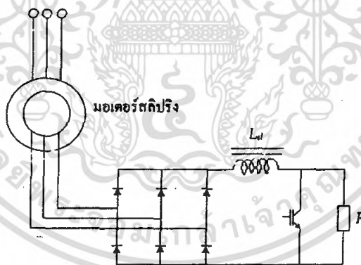
วงจรไดโอดบริดจ์เรกติไฟเออร์ ดิจิตอล
