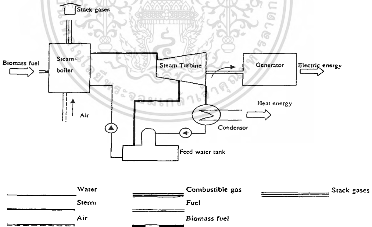
รูปที่ 2.7 แผนภาพโรงไฟฟ้าที่ใช้ความร้อนจากกระบวนการเผาไหม้โดยตรง
