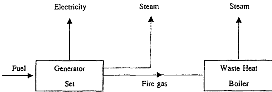
รูปที่ 2.9 แผนภาพการผลิตพลังงานร่วมแบบผลิตไฟฟ้านำหน้า
