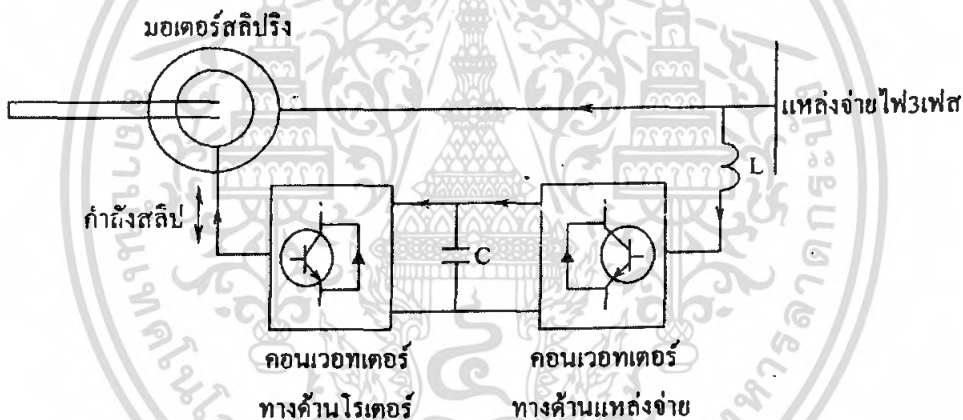
รูปที่ 3.7 วงจรภาคกำลังของเซอร์เบียสคอนเวอเตอร์ต่อแบบ back to back
