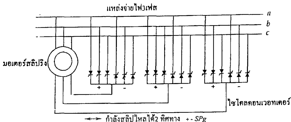
รูปที่ 3.6 วงจรภาคกำลังของระบบขับเคลื่อนเซอร์เบียสแบบสถิต
