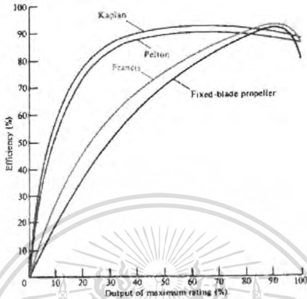
รูปที่ 3.15 แสดงประสิทธิภาพการแปลงรูปพลังงานของกังหันน้ำ
