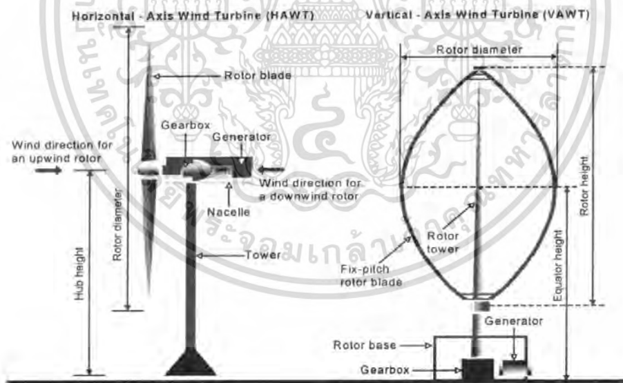
รูปที่ 3.1 กังหันลมผลิตไฟฟ้าแบบแกนนอนและแบบแกนตั้ง
