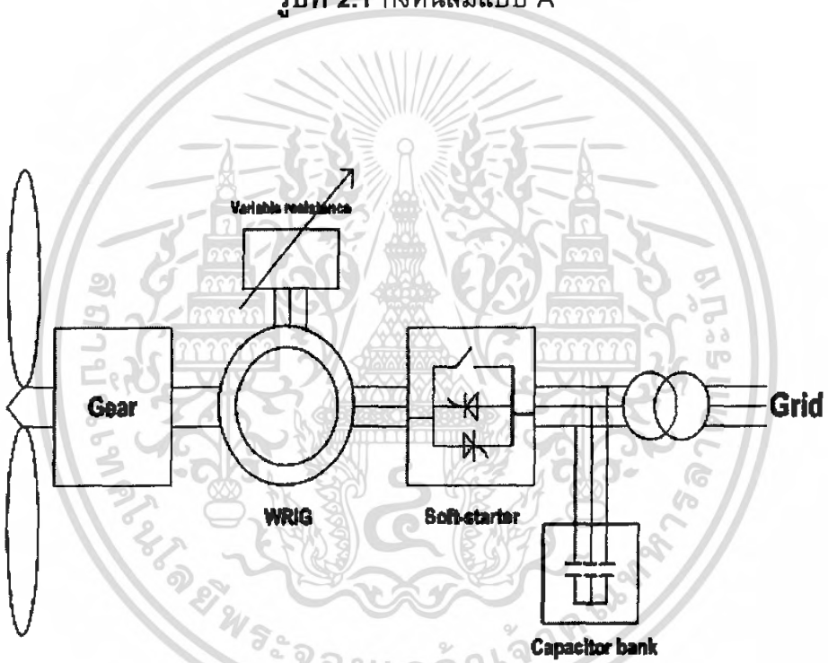
รูปที่ 2.1 กังหันลมแบบ A
