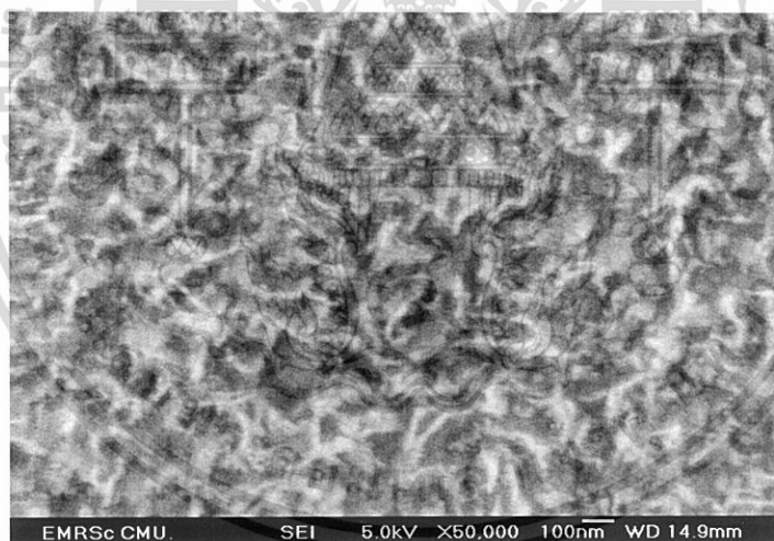
ภาพ SEM แสดงลักษณะทางกายภาพผิวหน้าของฟิล์มบางเมื่อเผาที่อุณหภูมิ 700 องศาเซลเซียส โดยมีสัดส่วนของอินเดียมต่อทินเป็น 7:3 กลุ่มเคลือบจำนวน 25 ชั้น
