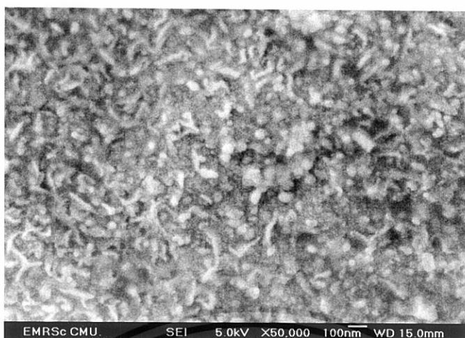
ภาพ SEM แสดงลักษณะทางกายภาพผิวหน้าของฟิล์มบางเมื่อเผาที่อุณหภูมิ 700 องศาเซลเซียส โดยมีสัดส่วนของอินเดียมต่อทินเป็น 9:1 รุ่มเคลือบจำนวน 20 ชั้น
