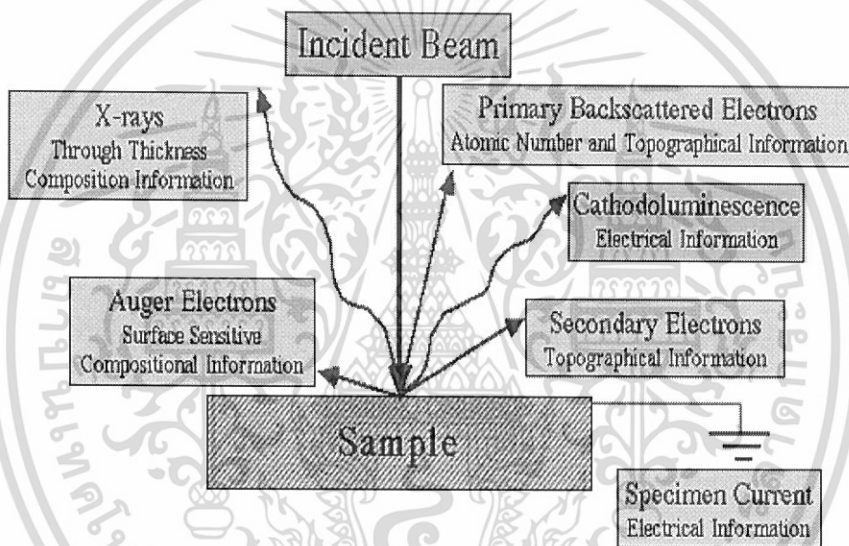
รูปที่ 2.20 การเกิดอันตรกิริยาระหว่างอิเล็กตรอนปฐมภูมิกับตัวอย่าง [27]
