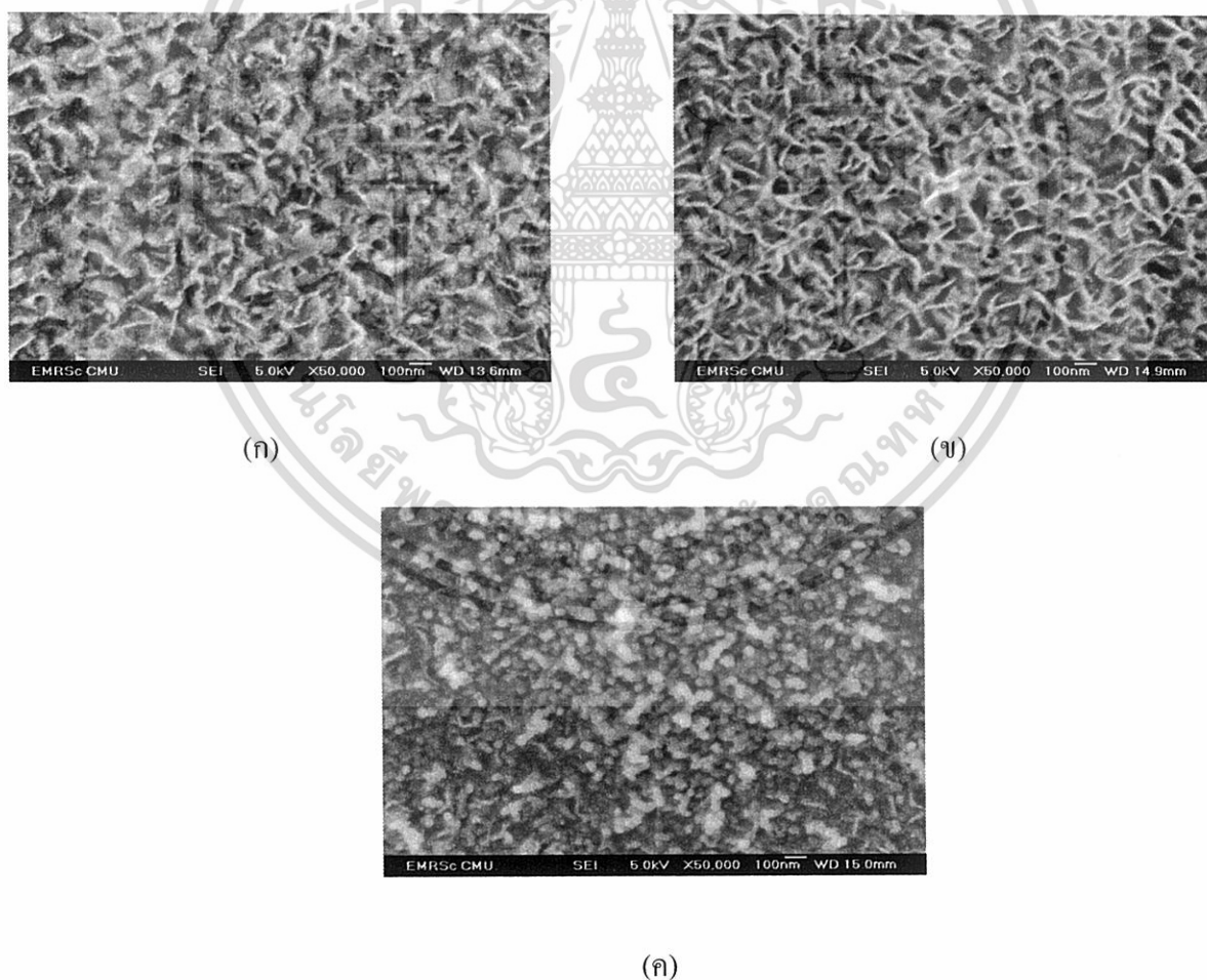
รูปที่ 4.3 ภาพ SEM แสดงลักษณะทางกายภาพผิวหน้าของฟิล์มบางเมื่อเผาที่อุณหภูมิ
