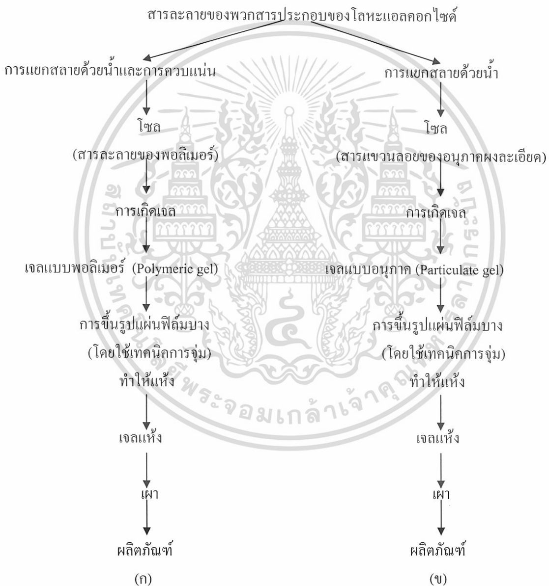
รูปที่ 2.4 ลำดับขั้นตอนต่างๆของกระบวนการเตรียมด้วยเทคนิค โซล-เจล แบบ [19]
