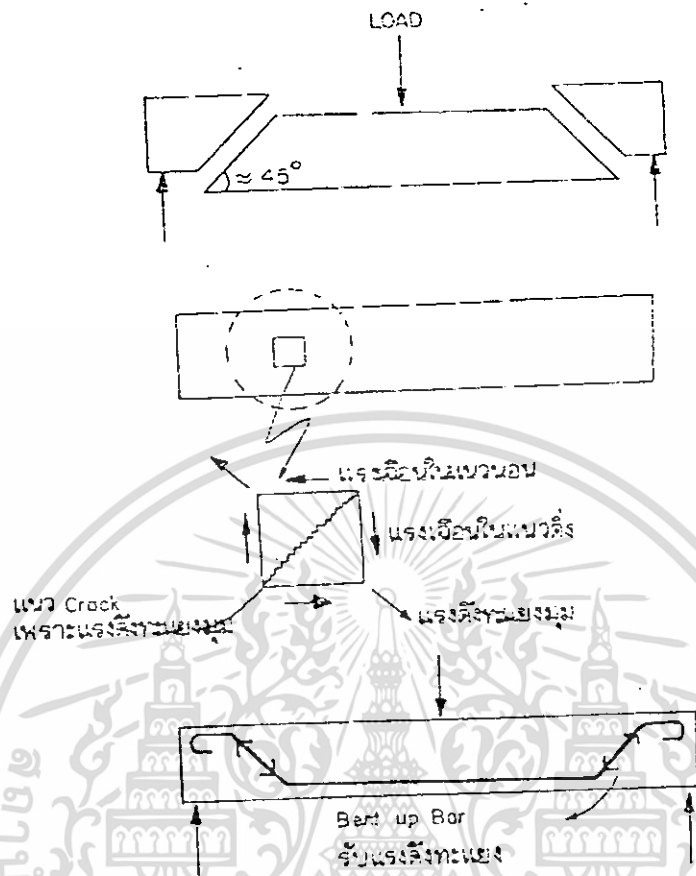
รูปที่ 4.16 แสดงลักษณะแรงเฉือน และแรงดึงทแยงมุมที่เกิดในคาน
