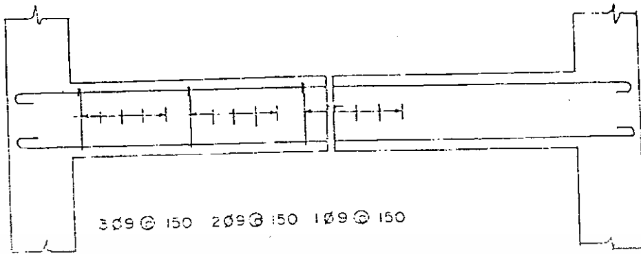
รูปที่ 4.24 แสดงการระบุจำนวนขนาด ระยะเรียง และช่วงเสริมเหล็กปลอกในคาน
