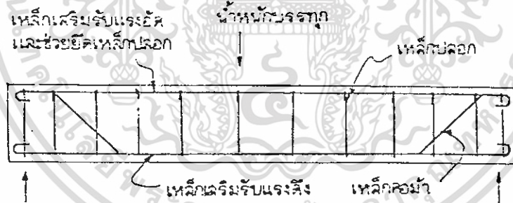
(c) การใช้เหล็กค้ำ และ เหล็กปลอกเพื่อรับแรงเฉือน
