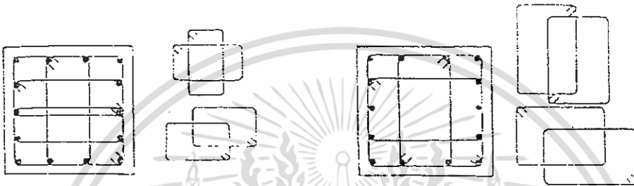
เหล็กชั้น 14 เส้นเหล็กปลอก 4 เส้น
