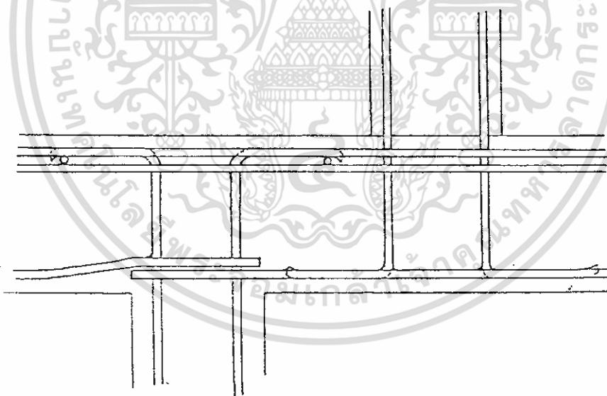
รูปที่ 4.10 แสดงการเสริมเหล็กเสาเยื้องศูนย์กลาง
