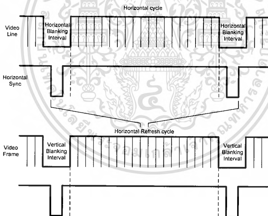
รูปที่ 2.3 ความสัมพันธ์ระหว่างสัญญาณทางด้านแนวอนและแนวตั้ง
