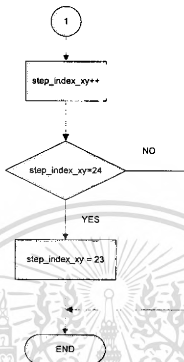
รูปที่ 3.7 แผนภาพแสดงแผนผังคำสั่งให้มอดอร์หมุนซ้าย
