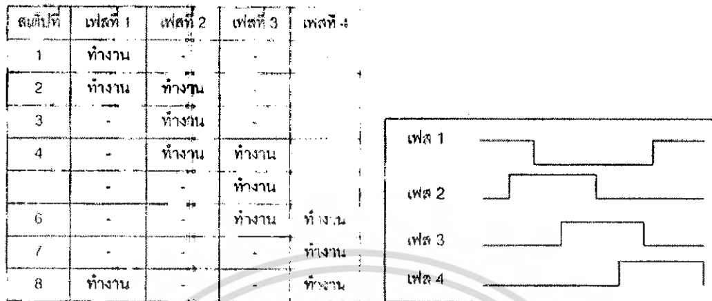
ก) Step Motor
