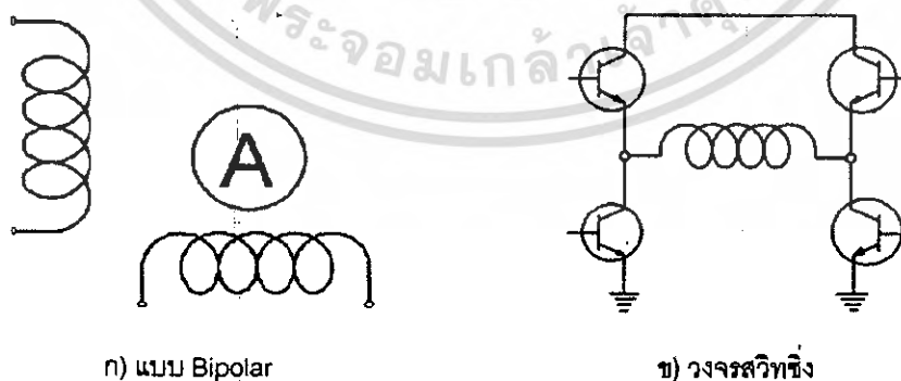
รูปที่ 2.30 แสดงการพันขดลวดและวงจรสวิตซ์แบบ Bipolar
