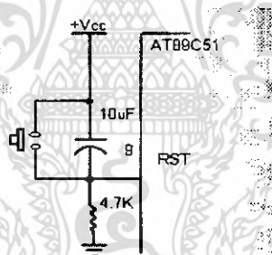
รูปที่ 2.18 วงจร Reset
