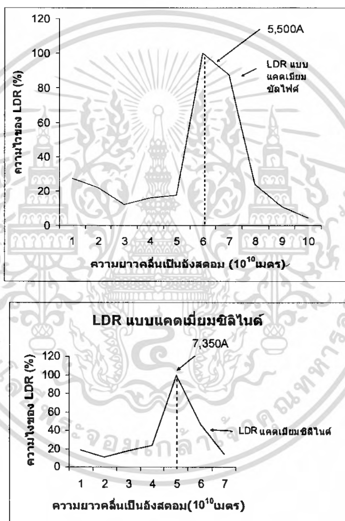
รูปที่ 2.2 ตัวอย่างกราฟแสดงความไวต่อแสงความถี่ต่างๆ ของ LDR ทั้ง 2 แบบ เมื่อเทียบกับความไวของคาคน
