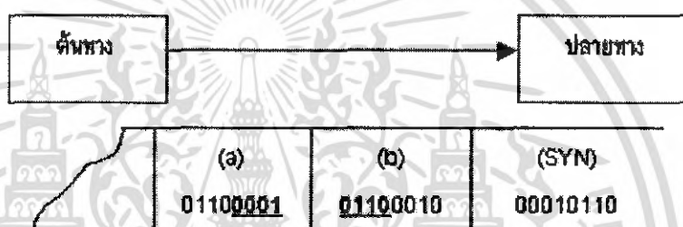
รูปที่ 2.12 รูปแบบบิต 01100001
