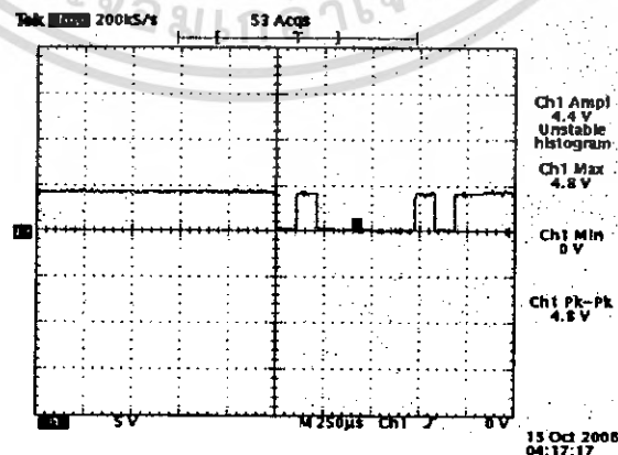
รูปที่ 4.7 สัญญาณเอาต์พุตของวงจรรีซีฟเตอร์ RS-485 ทางด้านรับ
