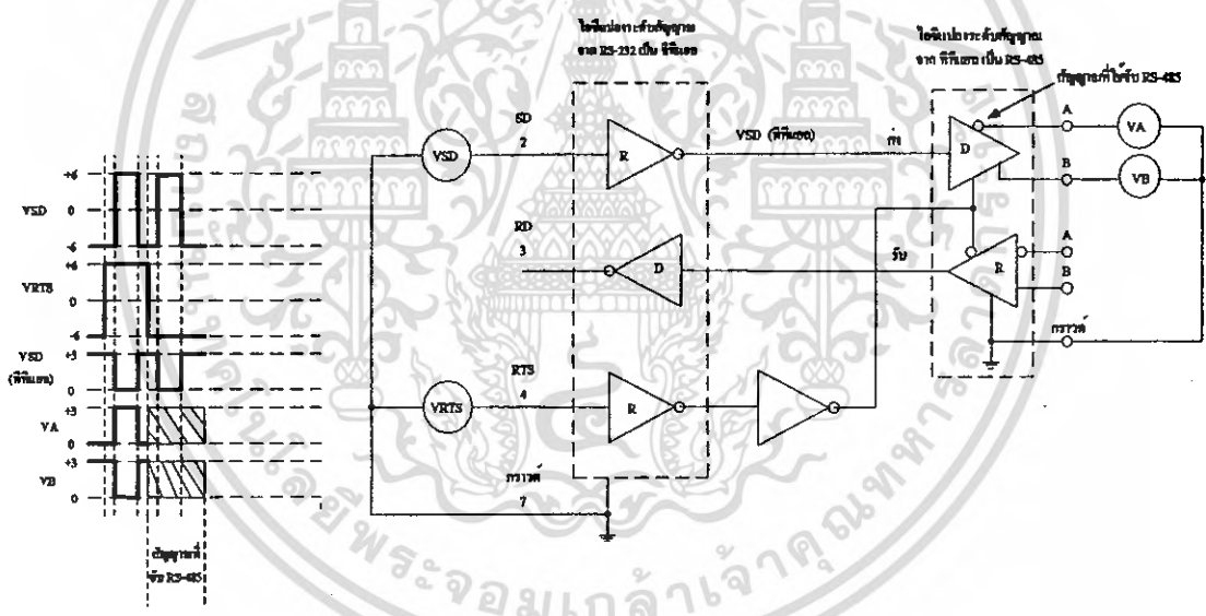
รูปที่ 2.6 แผนภาพแสดงการเปลี่ยนแปลงระดับสัญญาณ RS-232 เป็น RS-485 โดยใช้ RTS ควบคุมการส่งและรับของ RS-485
