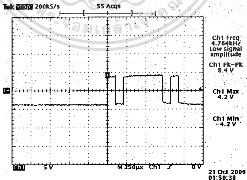
รูปที่ 4.5 สัญญาณข้อมูลสัญลักษณ์ "A" ที่ออกจากเอาต์พุตของวงจรรีซีฟเตอร์เฟส RS-485
