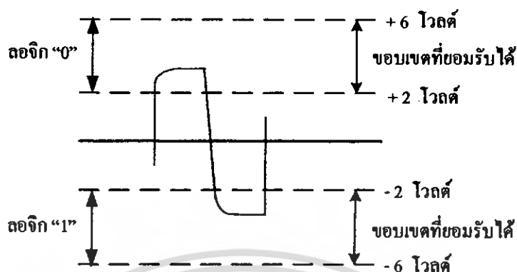
รูปที่ 2.2 เอาดัฟุดของตัวส่งแบบสมดุล
