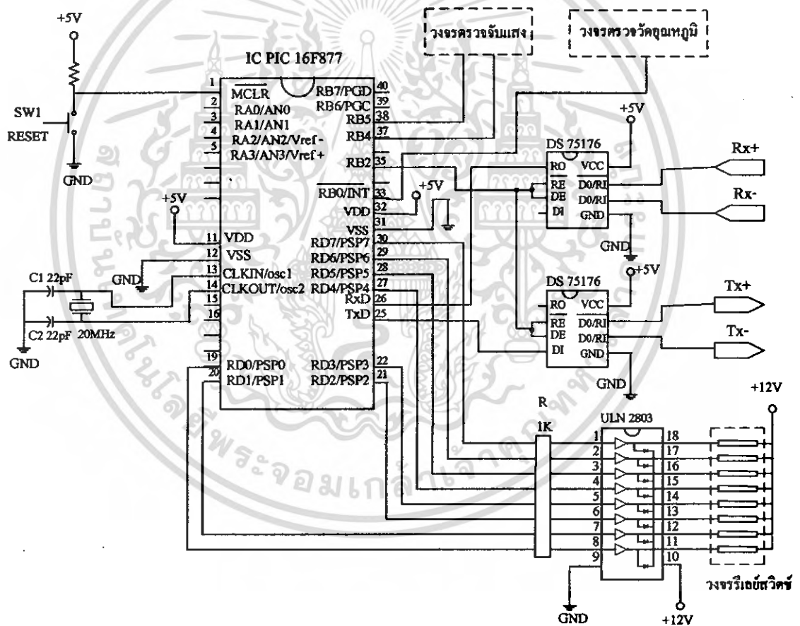
รูปที่ 3.4 วงจรไมโครคอนโทรลเลอร์ PIC 16F877
