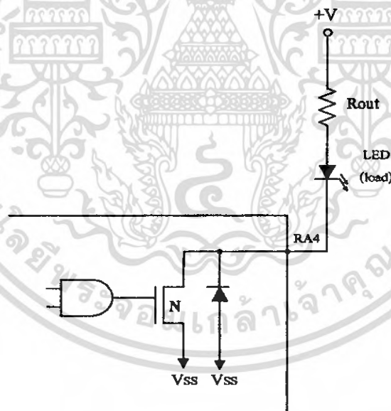
รูปที่ 2.12 การต่ออุปกรณ์เข้าที่ขาพอร์ต์ RA4 เมื่อใช้งานเป็นพอร์ต์เอาต์พุต
