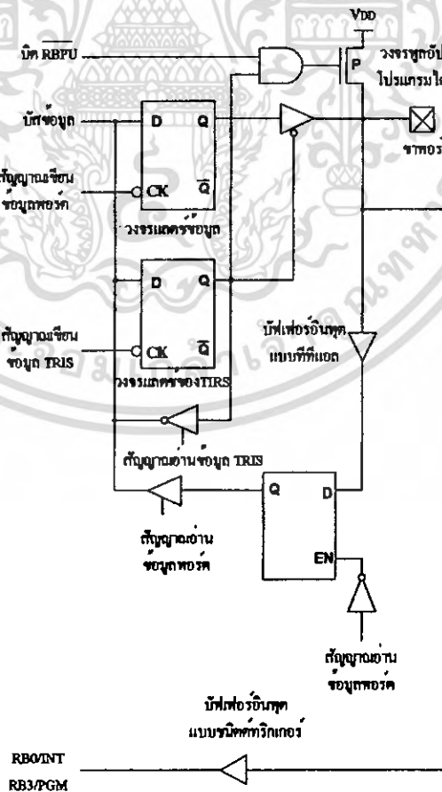
รูปที่ 2.13 โครงสร้างของขาพอร์ต B ในไมโครคอนโทรลเลอร์ PIC16F877 ขา RB0-RB3
