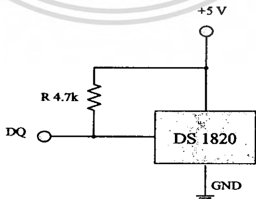
รูปที่ 3.7 วงจรตรวจจับอุณหภูมิ
