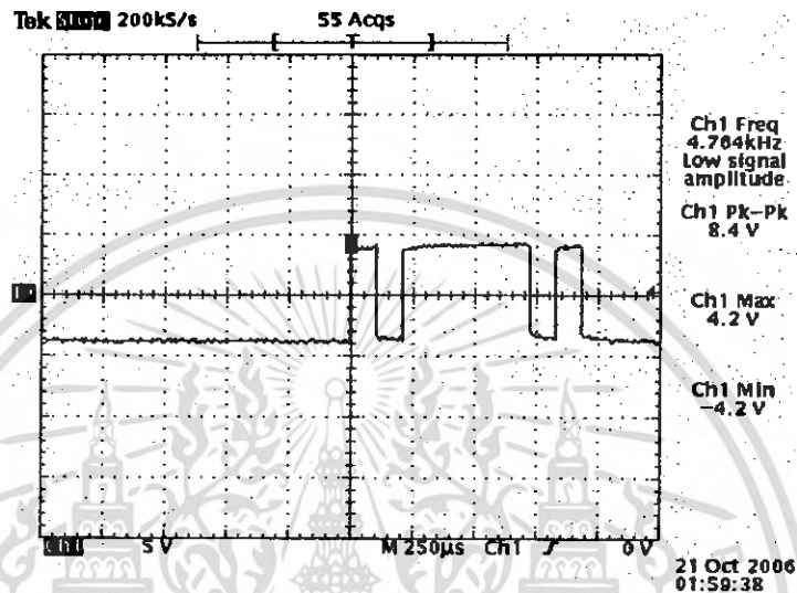
รูปที่ 4.6 สัญญาณอินพุตของวงจรรีซีฟเตอร์ RS-485 ทางด้านรับ
