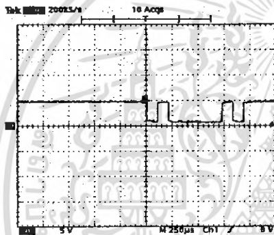
รูปที่ 4.3 สัญญาณเอาต์พุตที่ขา Tx-
