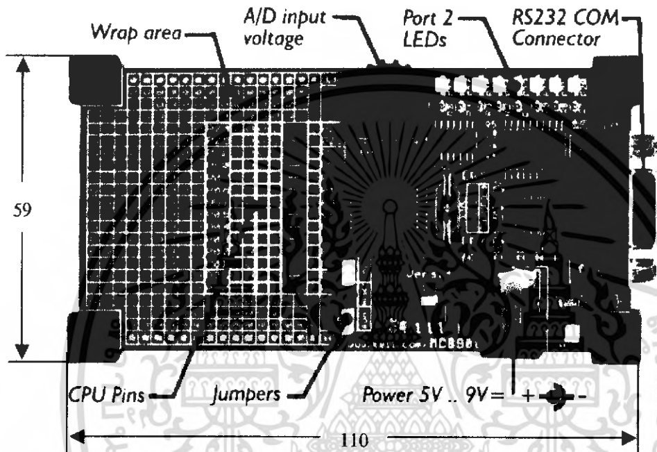
รูปที่4.5 บอร์ดพัฒนาโปรแกรม
