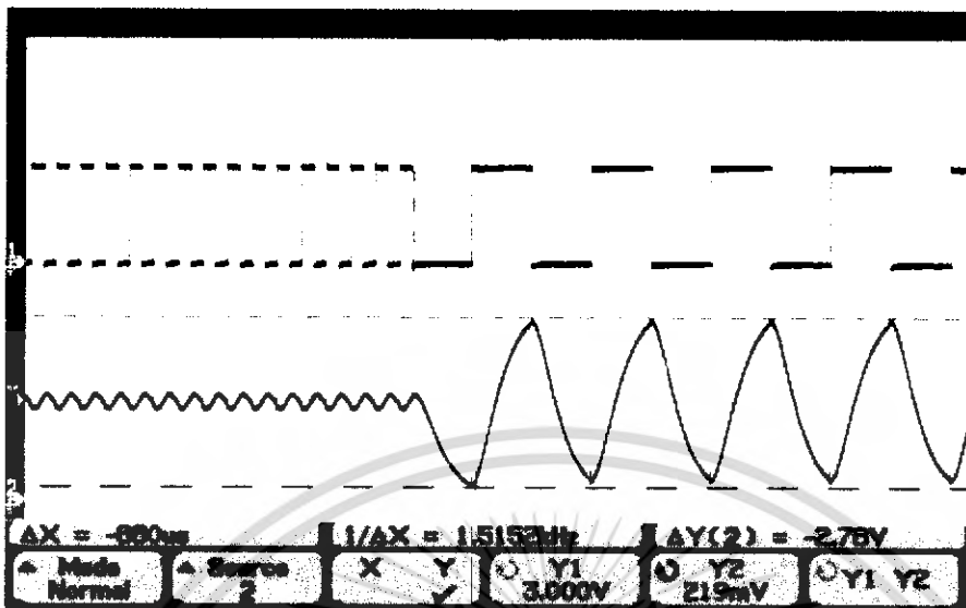
รูปที่ 4.9ก แสดง Transient ตอนเปลี่ยนสัญญาณจาก 4,000Hz เป็น 800Hz
