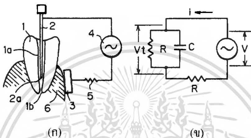
รูปที่ 2.9 ก แสดงถึงวงจรการกระตุ้นระหว่างลวดไฟล์กับขั้วอ้างอิงด้านแหล่งสัญญาณไฟฟ้าสลับ ข แสดงถึงวงจรสมมูลที่ใช้ในการวัด
