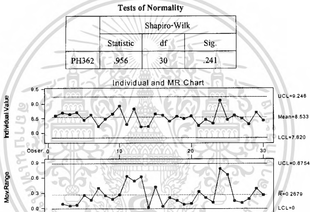
รูปที่ 4.24 แผนภูมิควบคุมสำหรับตัวอย่างเดี่ยว และแผนภูมิควบคุมค่าพิสัยเคลื่อนที่ของค่าความเป็นกรด-ด่างของผลิตภัณฑ์สีน้ำ V - Coat # E - 362
