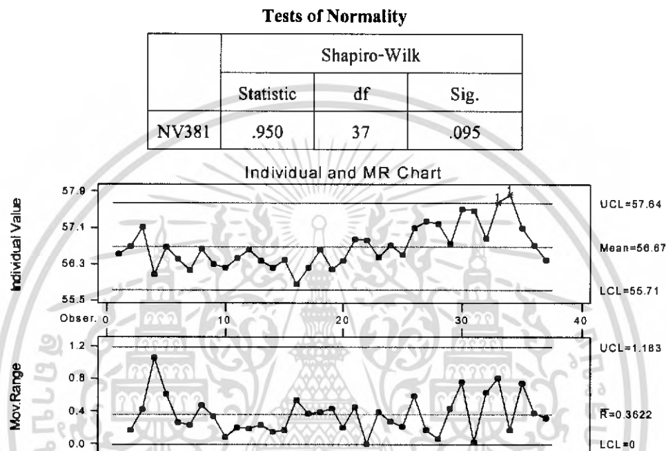
รูปที่ 4.26 แผนภูมิควบคุมสำหรับตัวอย่างเดี่ยว และแผนภูมิควบคุมค่าพิสัยเคลื่อนที่ของค่าปริมาณสารที่ไม่ระเหยของผลิตภัณฑ์สีน้ำ V - Coat # E - 381
