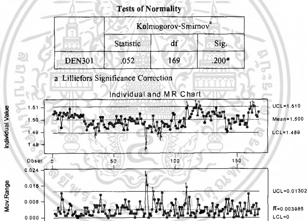
รูปที่ 4.3 แผนภูมิควบคุมสำหรับตัวอย่างเดี่ยว และแผนภูมิควบคุมค่าพิสัยเคลื่อนที่ของค่าความหนาแน่นของผลิตภัณฑ์สีน้ำ V - Coat # 301 White
