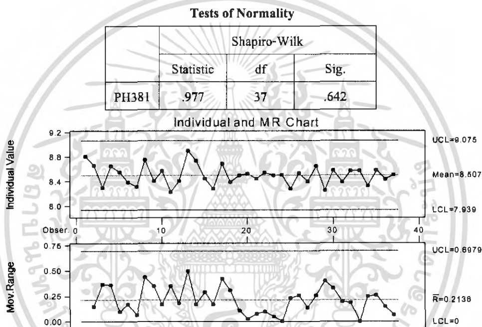
รูปที่ 4.29 แผนภูมิควบคุมสำหรับตัวอย่างเดี่ยว และแผนภูมิควบคุมค่าพิสัยเคลื่อนที่ของค่าความเป็นกรด-ด่างของผลิตภัณฑ์สีน้ำ V - Coat # E - 381
