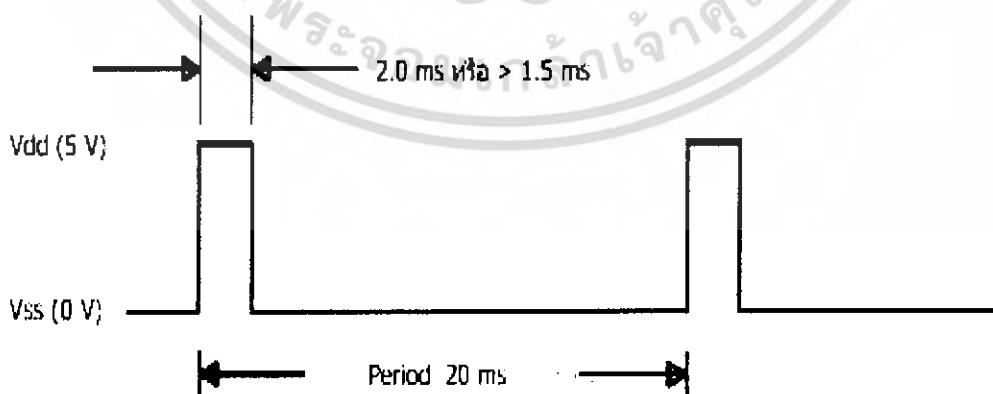
รูป 2.11 ความกว้างพัลส์
