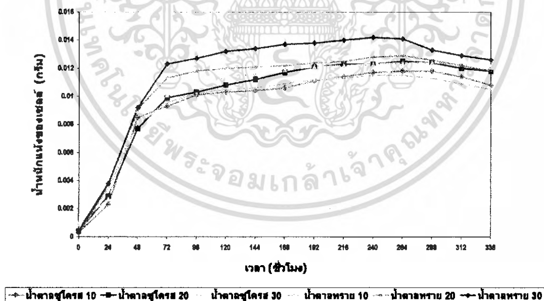
รูปที่ 4.7 น้ำหนักแห้งของเซลล์ที่เปลี่ยนแปลงเมื่อใช้น้ำตาลซูโครสและน้ำตาลทรายที่มีความเข้มข้นต่างๆ เป็นแหล่งคาร์บอน
