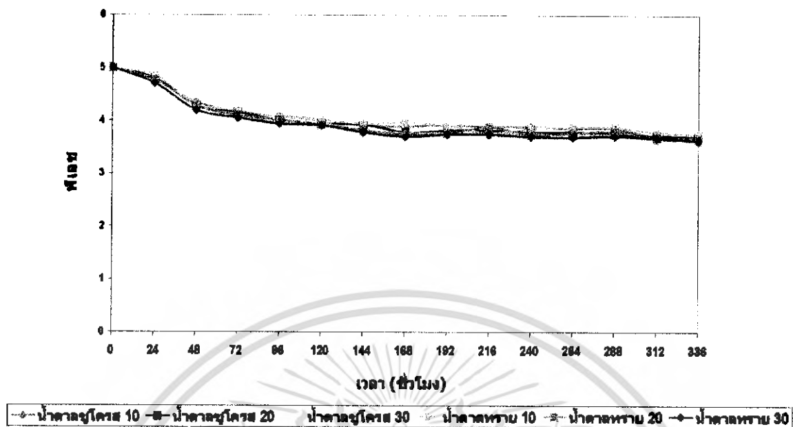
รูปที่ 4.10 ค่าความเป็นกรด - ค่างที่เปลี่ยนแปลงเมื่อนำน้ำตาลซูโครสและน้ำตาลทรายที่มีความเข้มข้นต่างๆ เป็นแหล่งคาร์บอน
