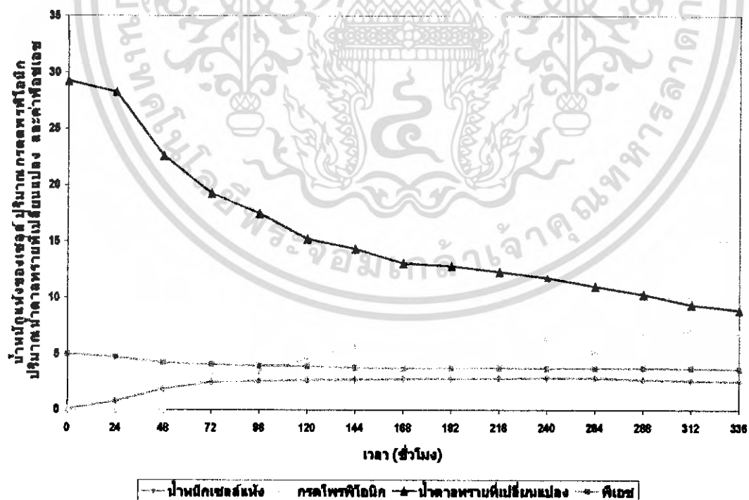
รูปที่ 4.11 น้ำหนักแห้งของเซลล์ ปริมาณกรดโพธิโณนิก ปริมาณน้ำตาลที่ใช้ไป และค่า
