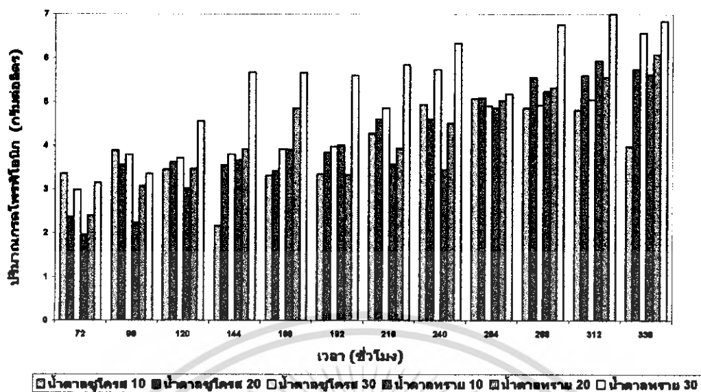
รูปที่ 4.8 ปริมาณกรดไพรูวิกที่ผลิตโดยเชื้อ P. acidipropionici ATCC4965 เมื่อใช้น้ำตาลซูโครสและน้ำตาลทรายที่ความเข้มข้นต่างๆ เป็นแหล่งคาร์บอน
