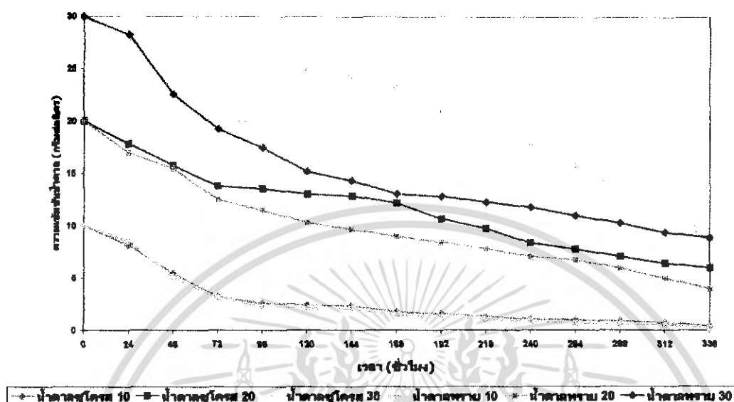
รูปที่ 4.9 ปริมาณน้ำตาลที่เปลี่ยนแปลงเมื่อใช้น้ำตาลชูโครสและน้ำตาลทรายที่มีความเข้มข้นต่างๆ เป็นแหล่งคาร์บอน
