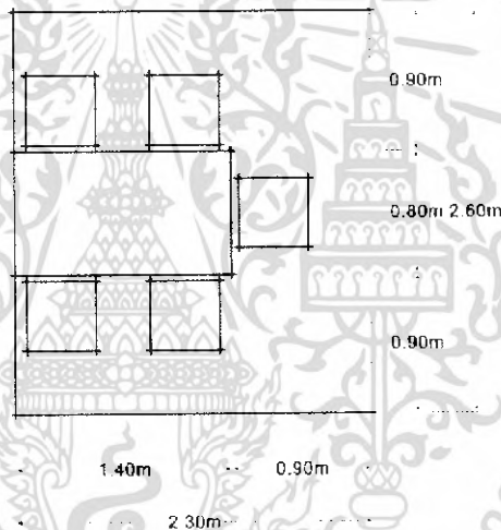
รูปที่ 4.6 รูปแบบการจัดพื้นที่นั่งรับประทานอาหาร ภายในส่วนอาคารร้านอาหาร แบบที่ 7
