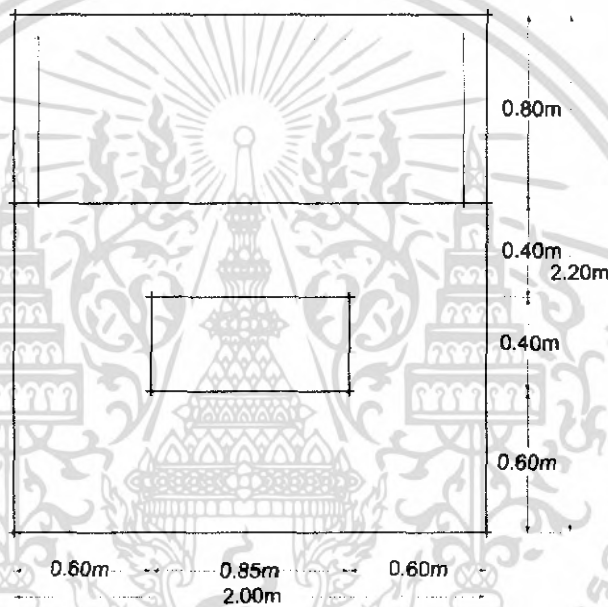
รูปที่ 4.14 รูปแบบการจัดที่นั่งส่วน พักผ่อน ภายในอาคารส่วนอาคารห้องพักแบบ Suite type แบบที่ 1
