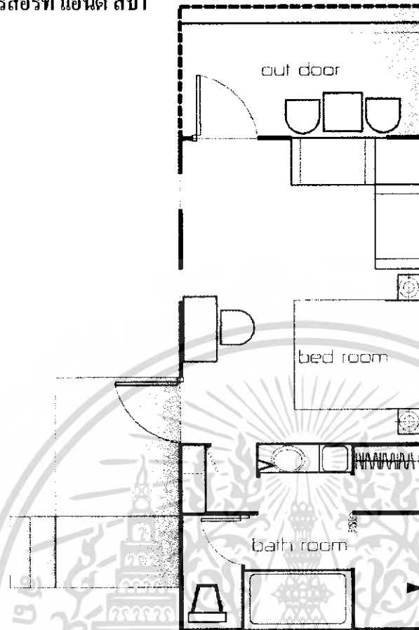
รูปที่ 2.23 ผังห้องพักแบบ DELUXE TYPE ของโครงการภูเก็ต รีสอร์ท แอนด์ สปา
