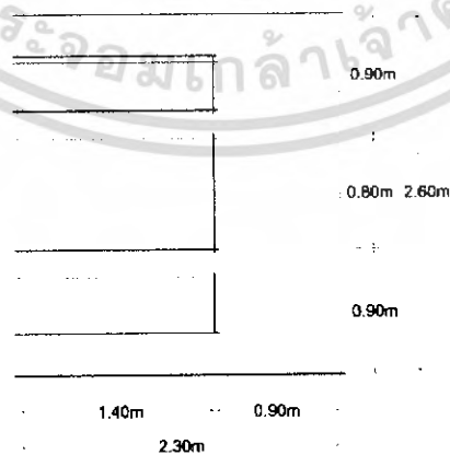
รูปที่ 4.7 รูปแบบการจัดพื้นที่นั่งรับประทานอาหาร ภายนอกอาคารส่วนอาคารร้านอาหาร แบบที่ 8
