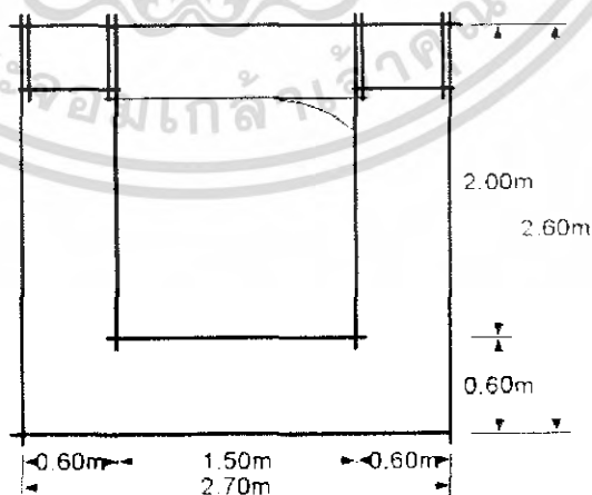
รูปที่ 4.13 รูปแบบการจัดส่วนห้องนอนแบบเตียงเดี่ยว (Double bed) ภายในส่วนอาคารห้องพักแบบ Suite type แบบที่ 3
