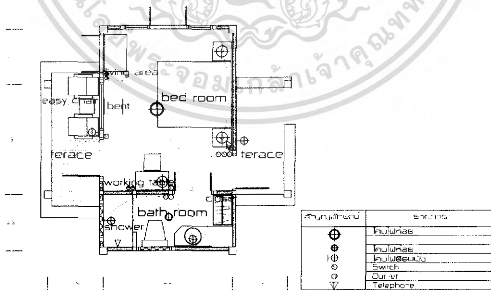
รูปที่ 5.24 ผังแปลนElectronic ห้องพักแบบDeluxe type
