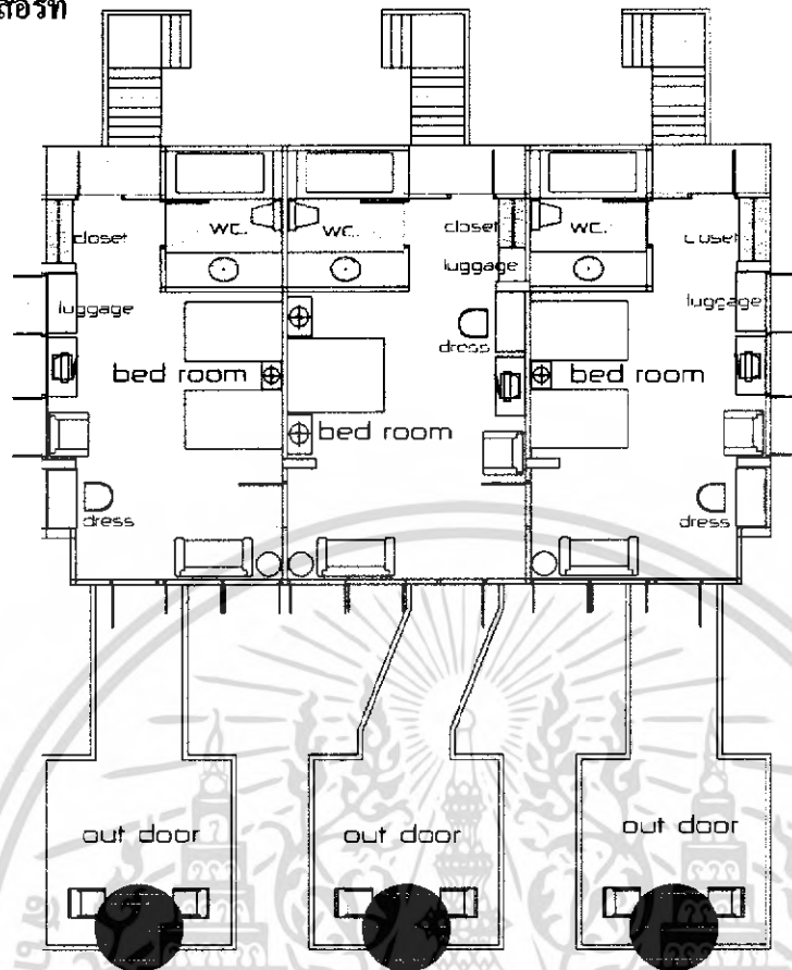
รูปที่ 3.49 ผังส่วนห้องพักแบบDELUXE TYPE สวนทิพย์วนารีสอร์ท
