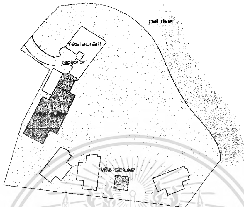
รูปที่ 2.6 ผังโดยรวม(Lay out) ของปายริเวอร์ คอนเนอท์ รีสอร์ท
