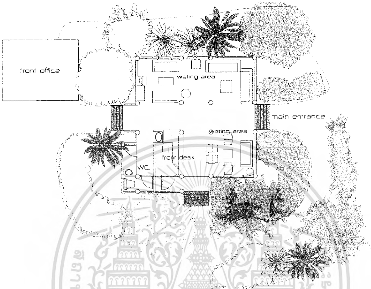
รูปที่ 2.10 การจัดแปลนส่วน อาคาร LOBBY บ้านกระทิง ปาย รีสอร์ท
