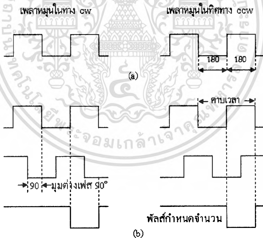
รูปที่ 2.13 (a) ตัวอย่างรูปคลื่นเอาท์พุทสี่เหลี่ยมของอุปกรณ์แอนโค้ดเดอร์ช่องเดียว (ไบไดเร็ก)
