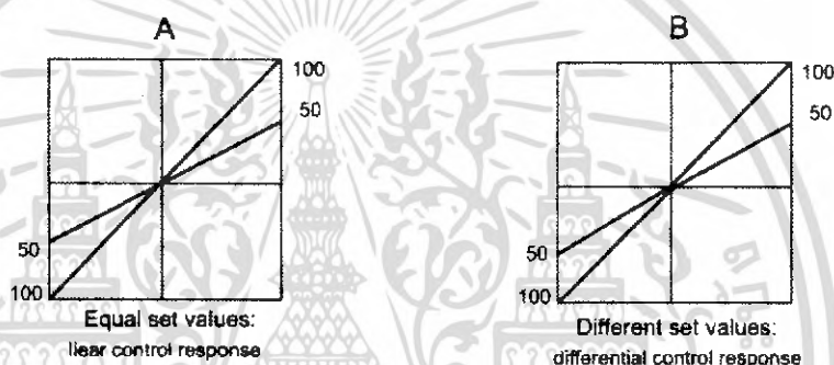
รูปที่ 3.10 ภาพโคออร์เดเนตของการปรับที่สมดุลกัน และการปรับที่ไม่สมดุลกัน
