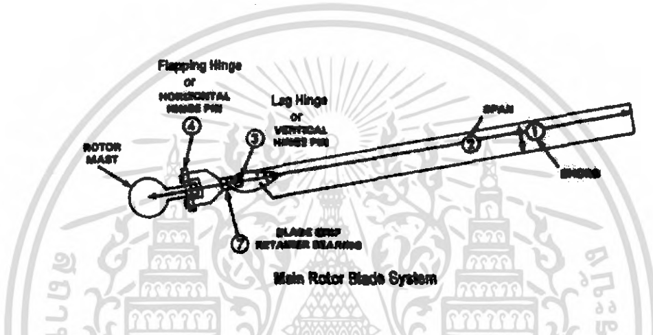
รูปที่ 2.16 ระบบการทำงานของใบพัดของมอเตอร์หลัก
