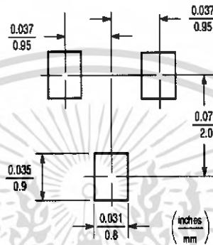
SOT-23
