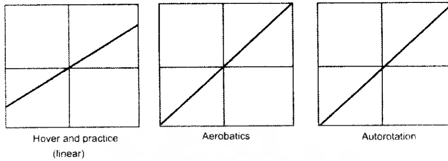
รูปที่ ๑.๘ ภาพระยะการเอียงท่ามุมของใบพัด
