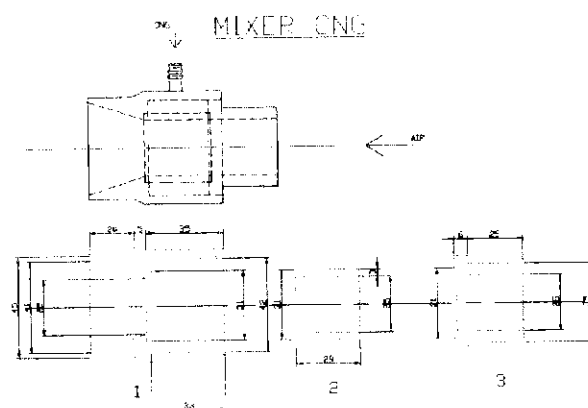
รูปที่ 4.6 แบบภายในก๊าชมิคเซอร์
