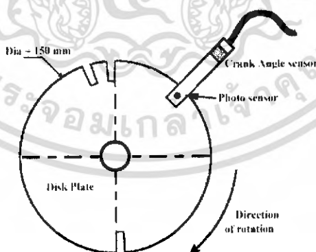
รูปที่ 4.18 การออกแบบและติดตั้ง Photo sensor กับแผ่น Plate ของตัวตรวจจับมุมมองสเตอริโอของเพลลาข้อเหวี่ยง
