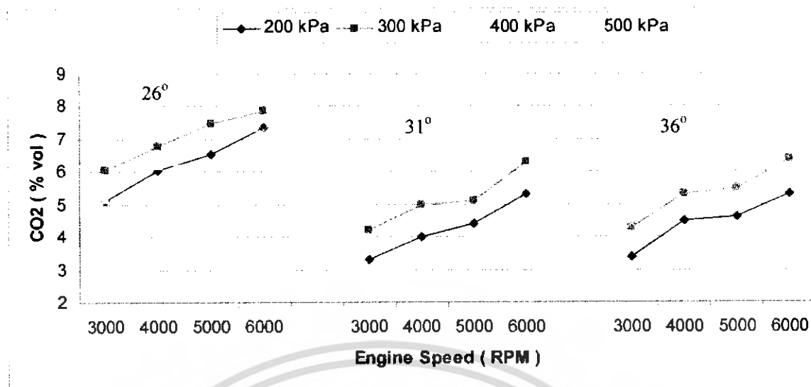
รูปที่ 6.26 ปริมาณคาร์บอนไดออกไซด์ที่ภาระงานและความเร็วรอบต่างๆ เปรียบเทียบผลระหว่างการเดินเครื่องที่องศาการจู่ระเบิดต่างๆ
