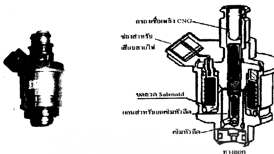
รูปที่ 4.11 หัวฉีดเชื้อเพลิงก๊าซธรรมชาติและส่วนประกอบ
