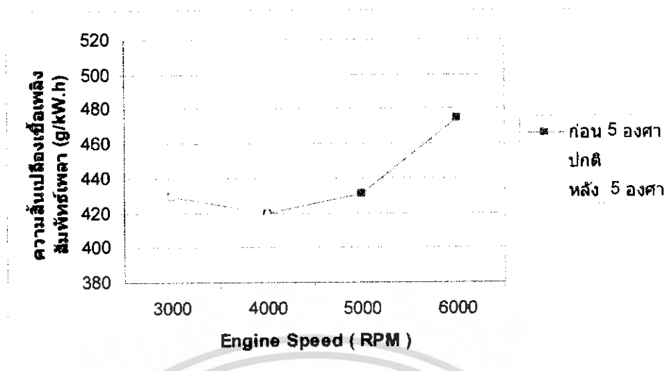
รูปที่ 6.14 ความสิ้นเปลืองเชื้อเพลิงสัมพัทธ์พล็อตที่ภาระงานคงที่ 200 kPa ที่องศาเพลาลูกเบี้ยวต่างๆ
