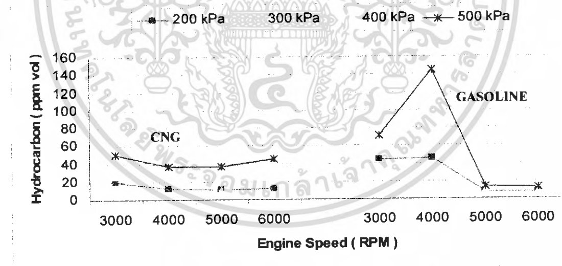
รูปที่ 6.12 เปรียบเทียบปริมาณสารไฮโดรคาร์บอนในไอเสียระหว่าง การติดเครื่องด้วยก๊าซธรรมชาติและน้ำมันแก๊สโซลีน
