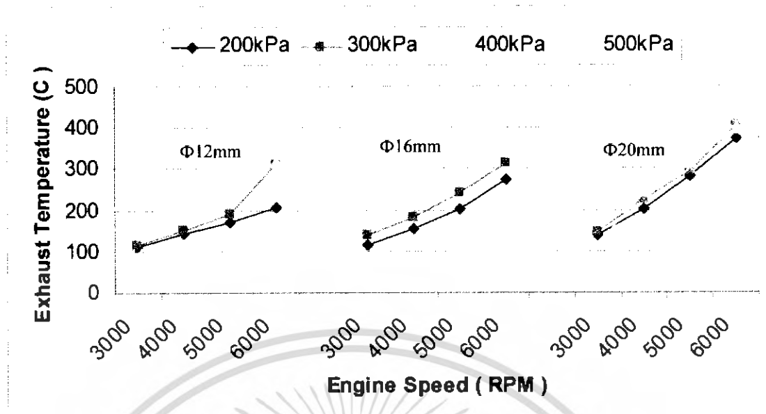
รูปที่ 6.9 เปรียบเทียบอุณหภูมิของก๊าซไอเสีย ณ จังหวะการเปิด-ปิดวาล์วไอเสียต่างๆกัน ที่สภาวะภาระคงที่ต่างๆ
