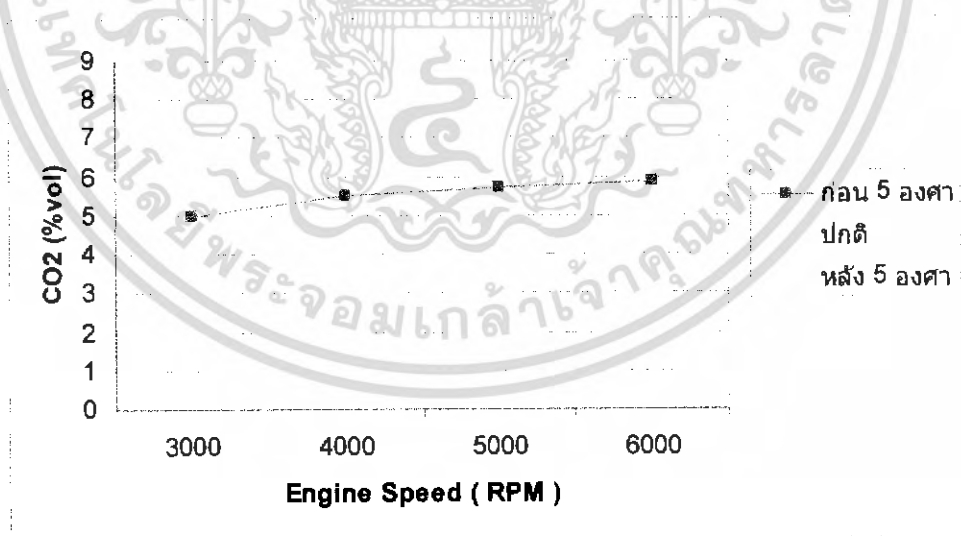
รูปที่ 6.18 ปริมาณคาร์บอนไดออกไซด์ที่ภาระงานคงที่ 300 kPa ที่องศาพลาถูกเบี้ยวต่างๆ
