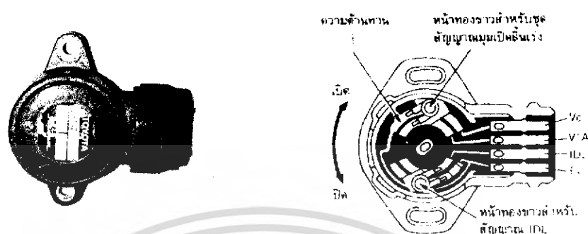
รูปที่ 4.23 ตัวตรวจจับตำแหน่งลิ้นเร่งและส่วนประกอบ
