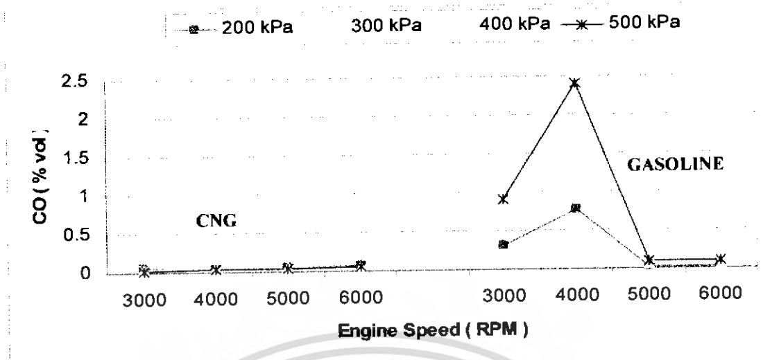
รูปที่ 6.11 เปรียบเทียบปริมาณคาร์บอนมอนอกไซด์ในไอเสียระหว่าง การติดเครื่องด้วยก๊าซธรรมชาติและน้ำมันแก๊สโซลีน
