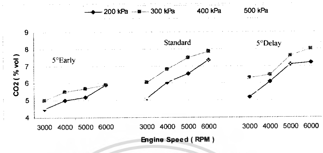
รูปที่ 6.17 ปริมาณคาร์บอนไดออกไซด์ที่ภาระงานและความเร็วรอบต่างๆ เปรียบเทียบผลระหว่างการเดินเครื่องที่องศาพลาถูกเบี้ยวต่างๆ
