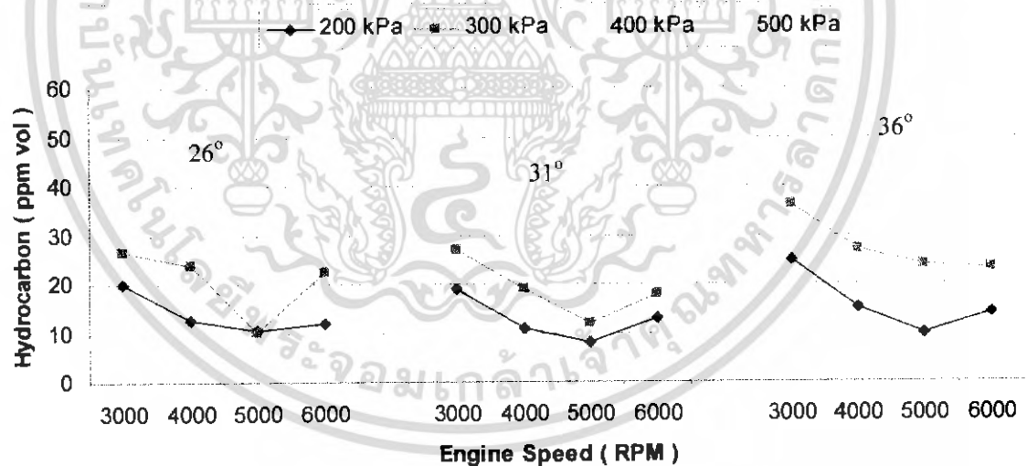
รูปที่ 6.28 ปริมาณสารไฮโดรคาร์บอนภาระงานและความเร็วรอบต่างๆ เปรียบเทียบผลระหว่างการเดินเครื่องที่องศาการจูดระเปิดต่างๆ
