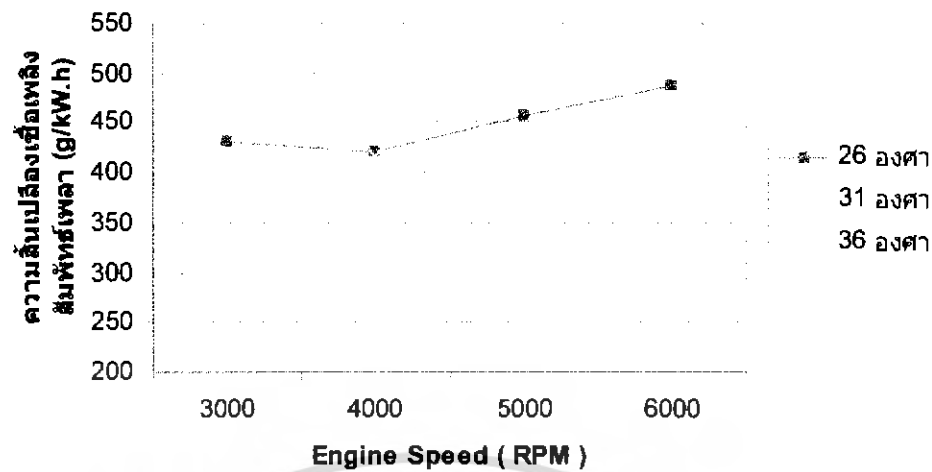
รูปที่ 6.23 อัตราสิ้นเปลืองเชื้อเพลิงสัมพัทธ์พล็อตที่ภาระงานคงที่ 200 kPa ที่องศาการจู่ระเบิดต่างๆ
