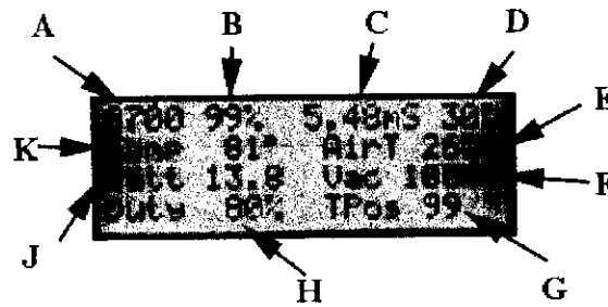
รูปที่ 4.16 จอแสดงผลค่าพารามิเตอร์ต่างๆในตัว hand controller
