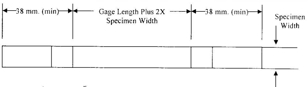
รูปที่ 3.9. แสดงชิ้นส่วนวัสดุที่ใช้สำหรับทดสอบเพื่อหาค่ารับแรงดึง เอกสารนี้เป็นเอกสารที่สงวนไว้สำหรับการใช้งานเพื่อการศึกษาเท่านั้น ไม่นิยมนำไปใช้ประโยชน์ด้านการค้า ไม่ว่าจะกรณีใดๆ ทั้งสิ้น อีกทั้งห้ามมิให้ดัดแปลงเนื้อหา และต้องอ้างอิงถึงเจ้าของเอกสารทุกครั้งที่มีการนำไปใช้
