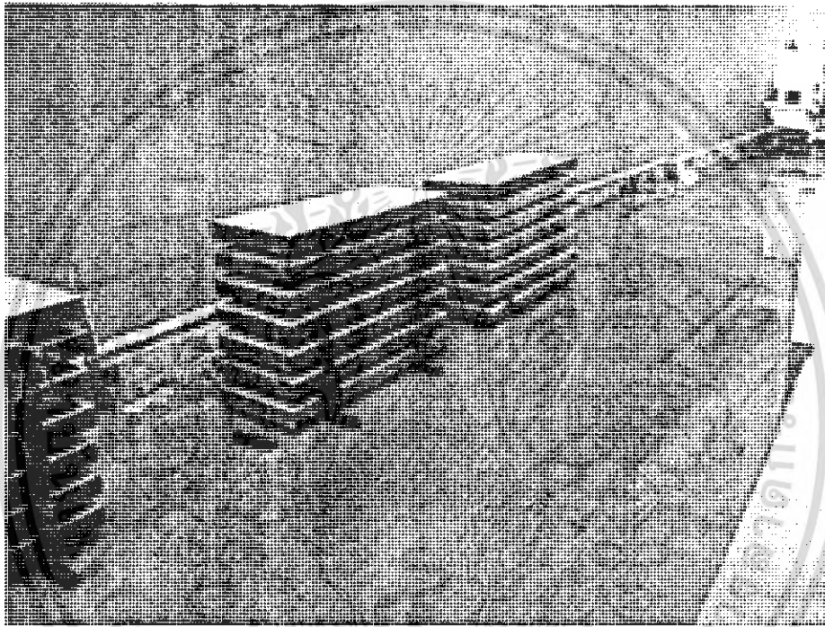
รูปที่ 3.27 แสดงการเตรียมแผ่นพื้นก่อนนำไปเสริมตาข่ายเส้นใยคาร์บอนด้านนอก
