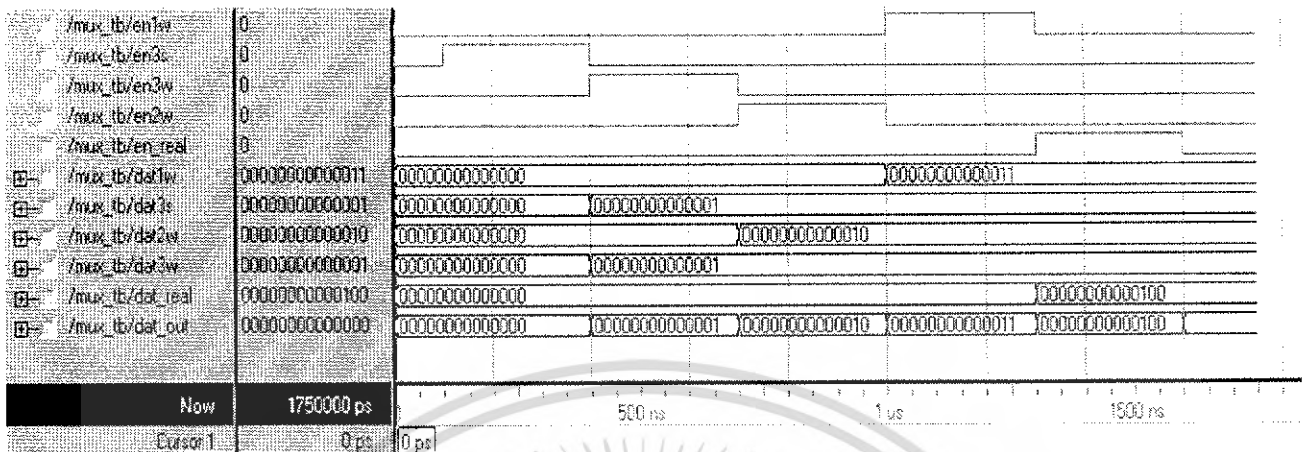
รูปที่ 4.53 แสดงผลการจำลองการทำงานของวงจรถมมุมวงจรวจรรมัลติเพล็กซ์
