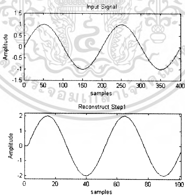
รูปที่ 4.11 แสดงผลในด้านตั้งเคราะห์ขั้นที่ 1 โดยจะมีส่วนของ input signal และส่วน
