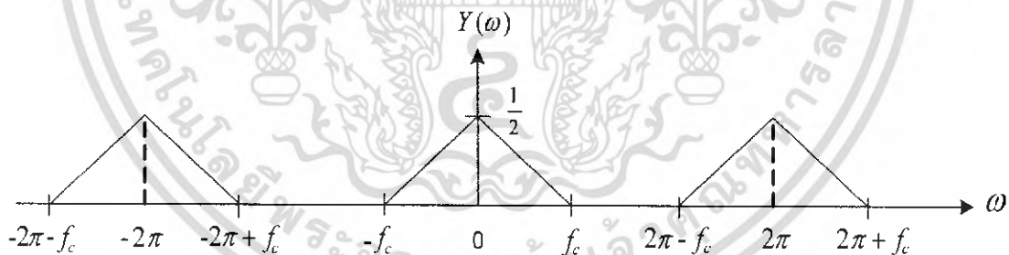
รูปที่ 2.9 สเปกตรัมของสัญญาณเอาต์พุตหลังจากผ่านการ downsampling
