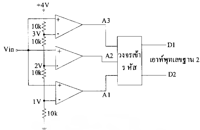
รูปที่ 2.42 แสดงการต่อวงจร Parallel Comparator A/D Converter
