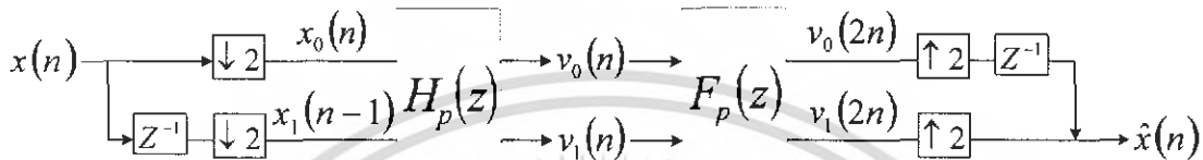
รูปที่ 2.31 แสดงรูปแบบส่วนวิเคราะห์และส่วนสังเคราะห์ ของฟิลเตอร์แบงก์
