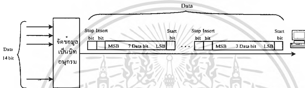
รูปที่ 3.24 แสดงบล็อกไดอะแกรมการแปลงข้อมูลส่งออกพอร์ตอนุกรมจากบอร์ด FPGA ไปยังคอมพิวเตอร์
