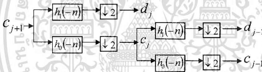
รูปที่ 2.11 แสดงการแตกกิ่งก้านสาขาแบบสองแถบสองขั้นของภาคส่ง
