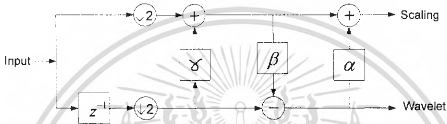
รูปที่ 2.36 แสดงโครงสร้างทัวไปของ Lifting scheme ทางภาควิเคราะห์
