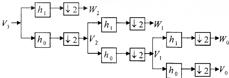
รูปที่ 2.12 แสดงการแตกกิ่งก้านสาขาแบบสองแถบสามขั้นของภาคส่ง
