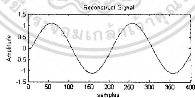
รูปที่ 4.13 แสดงผลในด้านสังเคราะห์ขั้นที่ 3 โดยจะมีส่วนของ input signal และส่วนของ reconstruct step3
