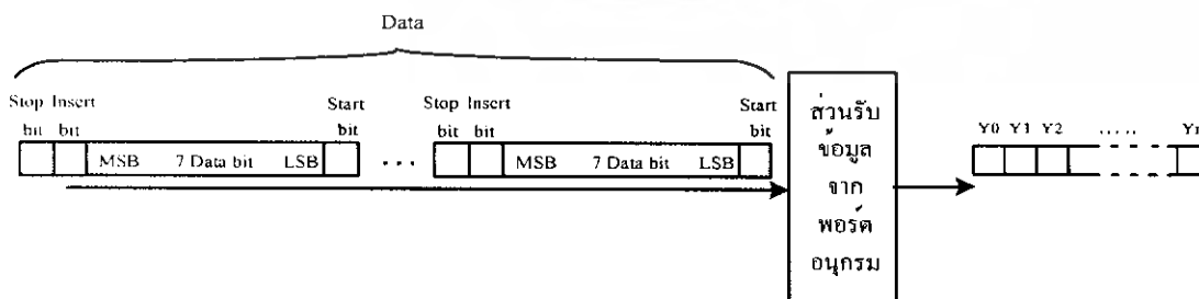
รูปที่ 3.25 แสดงบล็อกไดอะแกรมการรับบิตข้อมูลจากบอร์ด FPGA ผ่านทางพอร์ตอนุกรม
