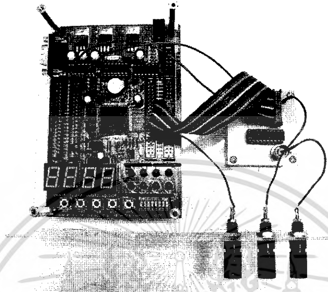
รูปที่ 4.66 แสดงบอร์ดเฟฟฟิจเอที่ทำการเชื่อมต่อกับพอร์ทอนุกรม
