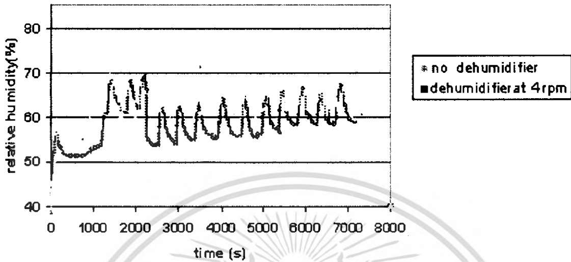
รูปที่ 4.1 กราฟเปรียบเทียบความชื้นสัมพัทธ์ในช่วงความเร็วรอบ 4 rpm ของวงล้อ ที่ระดับความชื้นสัมพัทธ์ 58 - 65 เปอร์เซ็นต์ ชิลิกาเจล 7 กิโลกรัม
