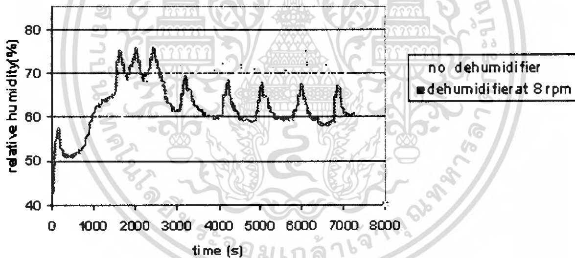
รูปที่ 4.18 กราฟเปรียบเทียบความชื้นสัมพัทธ์ในช่วงความเร็วรอบ 8 rpm ของวงล้อ ที่ระดับความชื้นสัมพัทธ์ 65-75 เปอร์เซ็นต์ ซิสิกานจอ 5.75 กิโลกรัม
