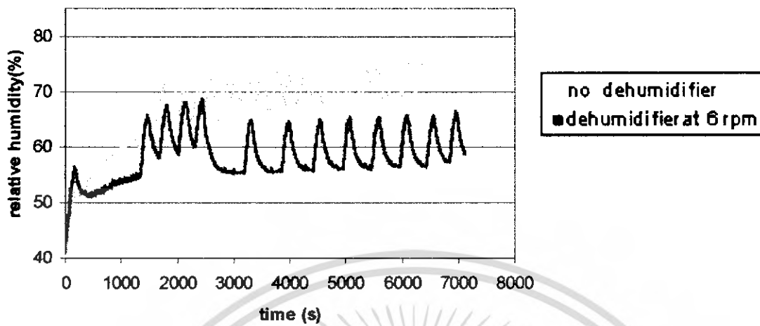
รูปที่ 4.11 กราฟเปรียบเทียบความชื้นสัมพัทธ์ในช่วงความเร็วรอบ 6 rpm ของวงล้อ ที่ระดับความชื้นสัมพัทธ์ 65-75 เปอร์เซ็นต์ ซิอิกาเจด 7 กิโลกรัม
