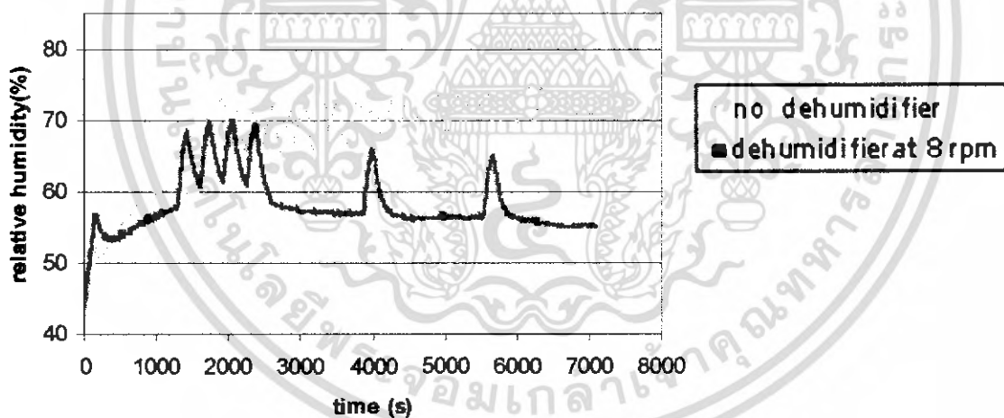
รูปที่ 4.12 กราฟเปรียบเทียบความชื้นสัมพัทธ์ในช่วงความเร็วรอบ 8 rpm ของวงล้อ ที่ระดับความชื้นสัมพัทธ์ 65-75 เปอร์เซ็นต์ ซิอิกาเจด 7 กิโลกรัม
