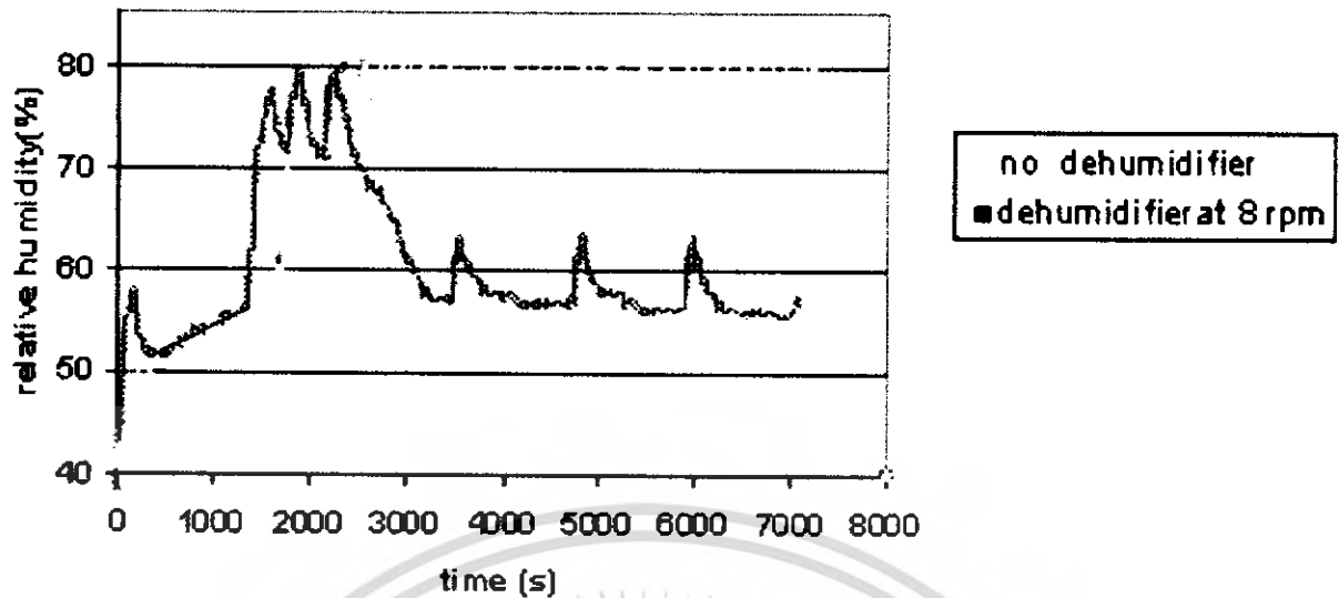
รูปที่ 4.27 กราฟเปรียบเทียบความชื้นสัมพัทธ์ในช่วงความเร็วรอบ 8 rpm ของวงล้อ ที่ระดับความชื้นสัมพัทธ์ 75 - 80 เปอร์เซ็นต์ จลิกานจอต 5.75 กิโลกรัม
