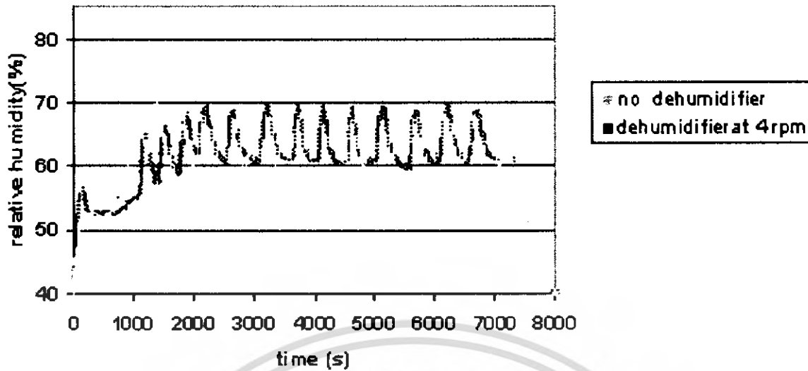
รูปที่ 4.7 กราฟเปรียบเทียบความชื้นสัมพัทธ์ในช่วงความเร็วรอบ 4 rpm ของวงล้อ ที่ระดับความชื้นสัมพัทธ์ 58 - 65 เปอร์เซ็นต์ ซิสิกานอล 5.75 กิโลกรัม
