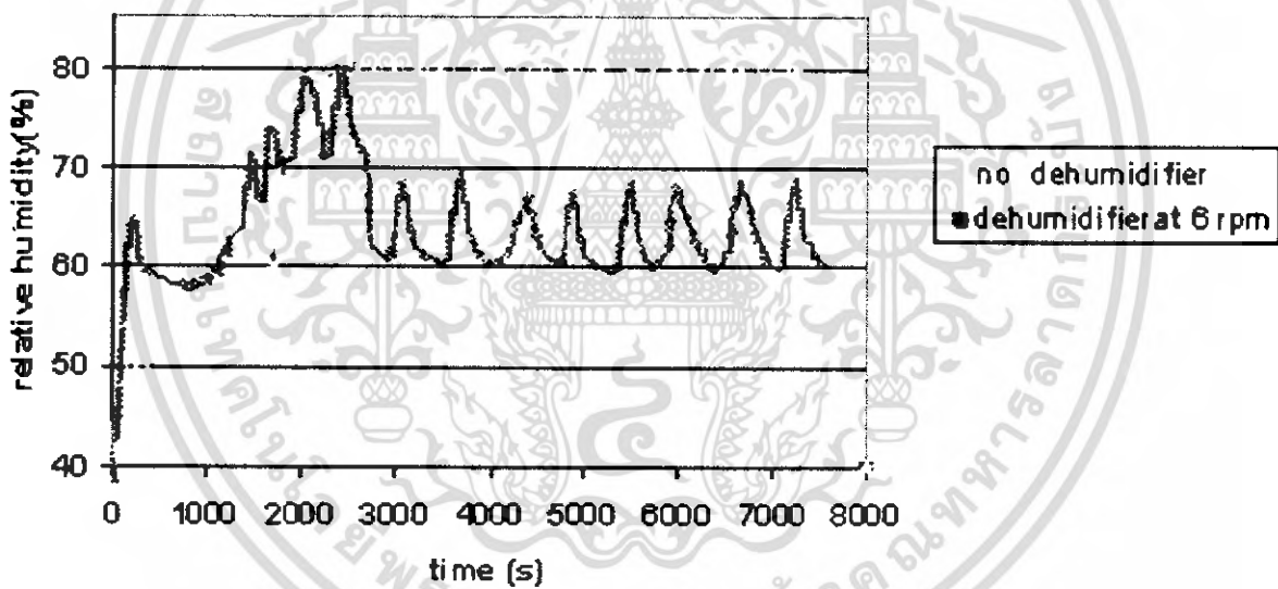
รูปที่ 4.26 กราฟเปรียบเทียบความชื้นสัมพัทธ์ในช่วงความเร็วรอบ 6 rpm ของวงล้อ ที่ระดับความชื้นสัมพัทธ์ 75 - 80 เปอร์เซ็นต์ จลิกานจล 5.75 กิโลกรัม
