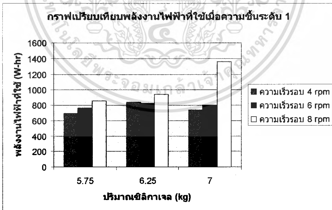
รูปที่ 4.30 กราฟเปรียบเทียบพลังงานไฟฟ้าที่ใช้เมื่อความชื้นสัมพัทธ์ 58-65 เปอร์เซ็นต์ นำไปใช้ประโยชน์ด้านการค้า
