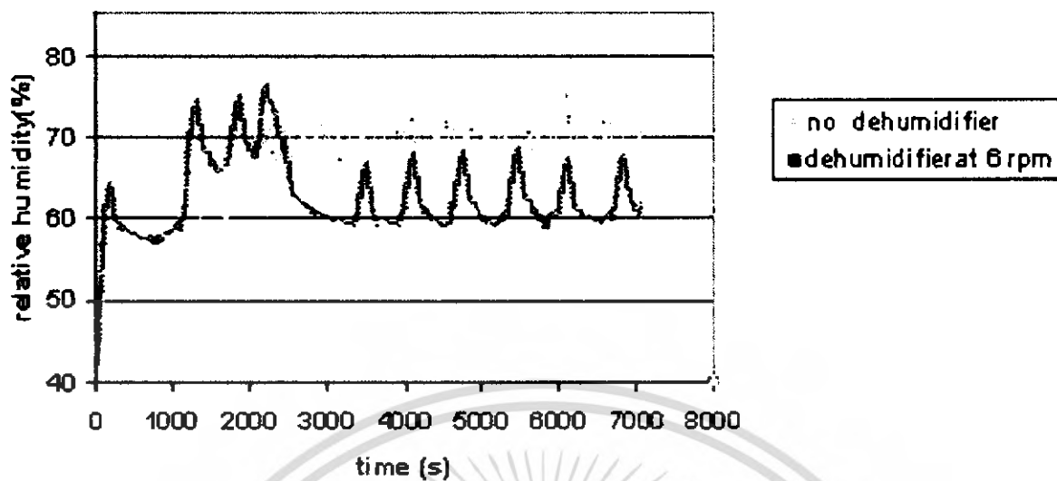
รูปที่ 4.17 กราฟเปรียบเทียบความชื้นสัมพัทธ์ในช่วงความเร็วรอบ 6 rpm ของวงล้อ ที่ระดับความชื้นสัมพัทธ์ 65-75 เปอร์เซ็นต์ ซิสิกานจอ 5.75 กิโลกรัม
