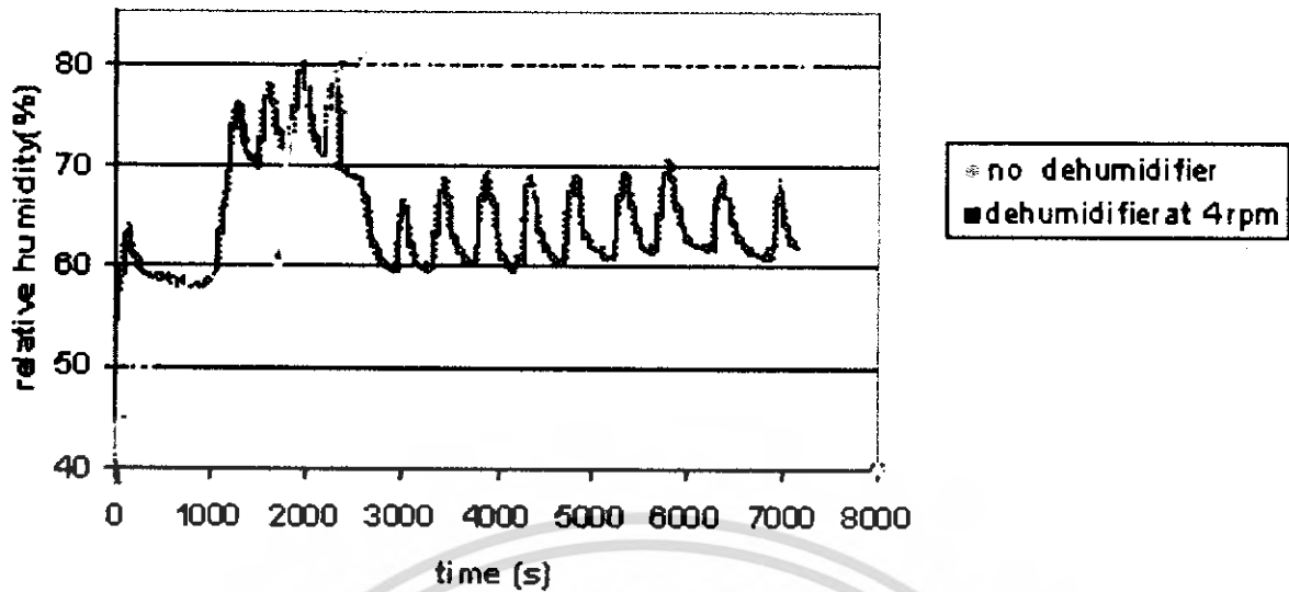
รูปที่ 4.25 กราฟเปรียบเทียบความชื้นสัมพัทธ์ในช่วงความเร็วรอบ 4 rpm ของวงล้อ ที่ระดับความชื้นสัมพัทธ์ 75 - 80 เปอร์เซ็นต์ จลิกานจล 5.75 กิโลกรัม
