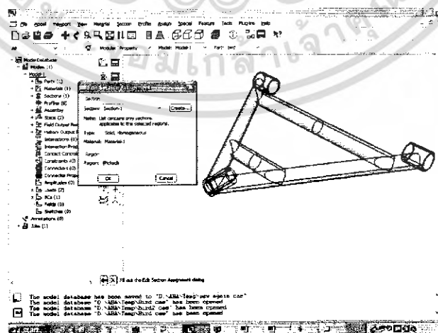
รูปที่ 5-70 แสดงการกำหนด Section ลงในปีกนก
