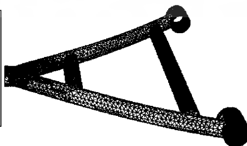
รูปที่ 3-14 การทดลองความเสียหายของปีกนกจากโปรแกรม ABAQUS
