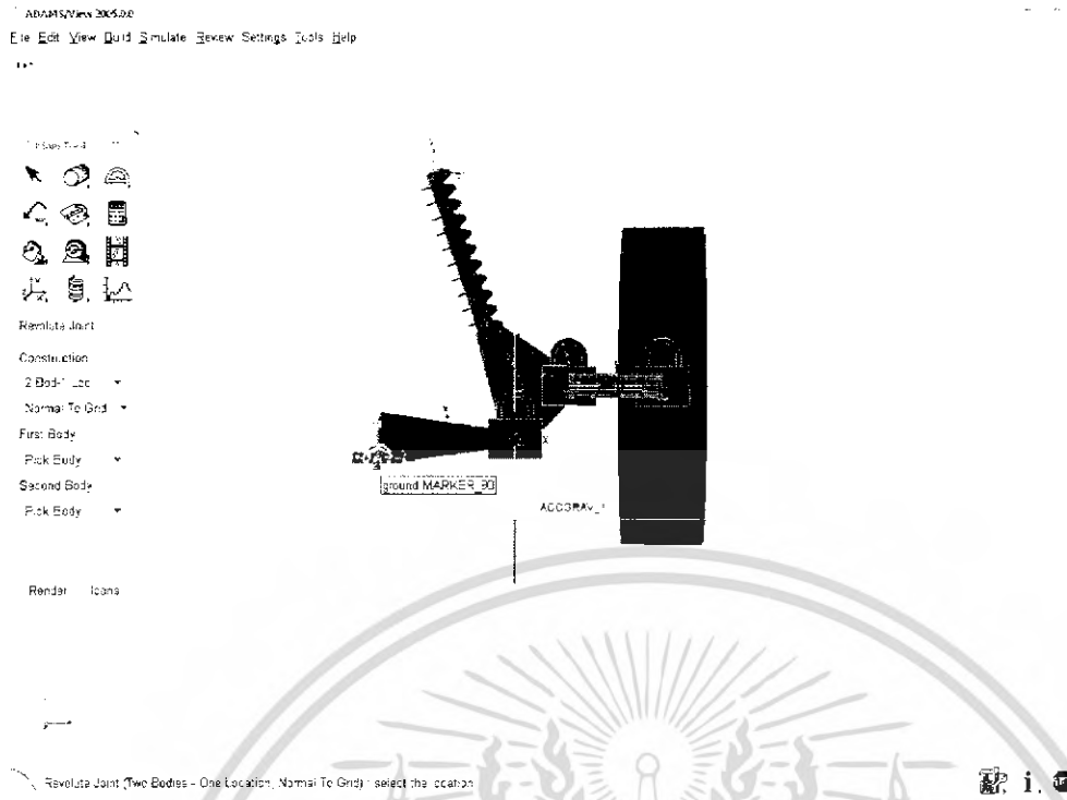
รูปที่ 5-12 การยึดจุดหมุนที่ปีกนกกับโครงรถ
