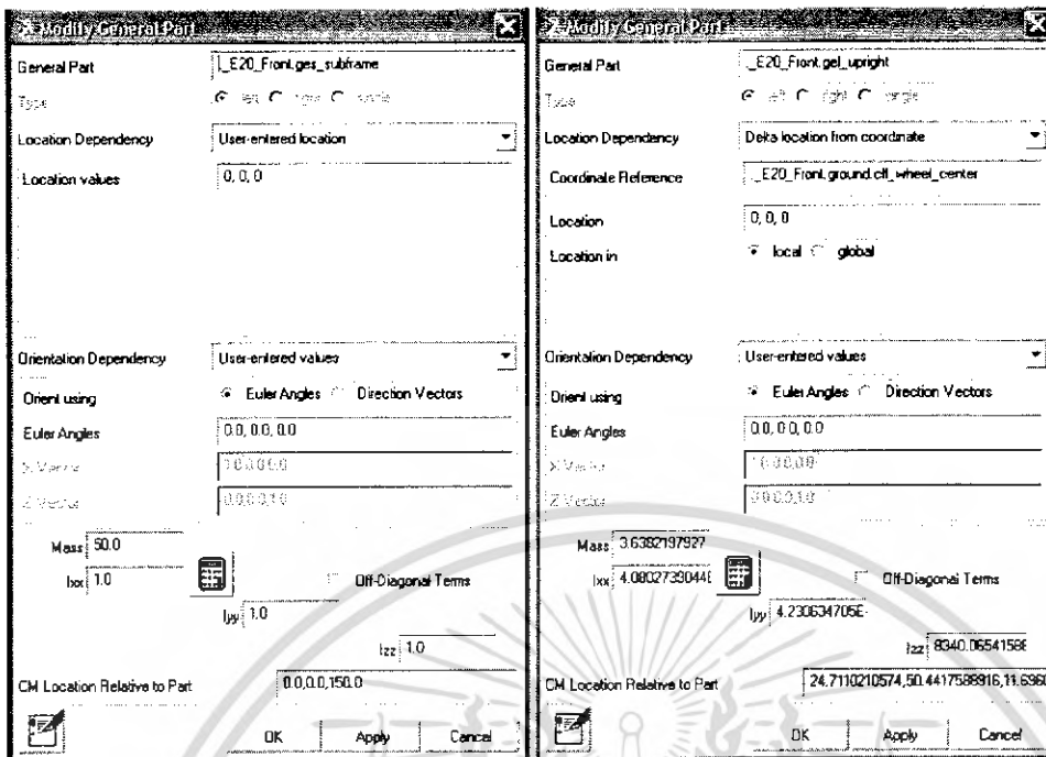
รูปที่ 5-55 แสดงหน้าต่างการสร้างพาร์ท subframe และ upright
