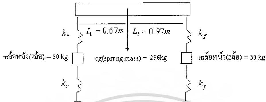
รูปที่ 4-2 แบบจำลองการสั่นแบบระดับชั้นความเร็วเท่ากับ 4 ของรถไฟฟ้า
