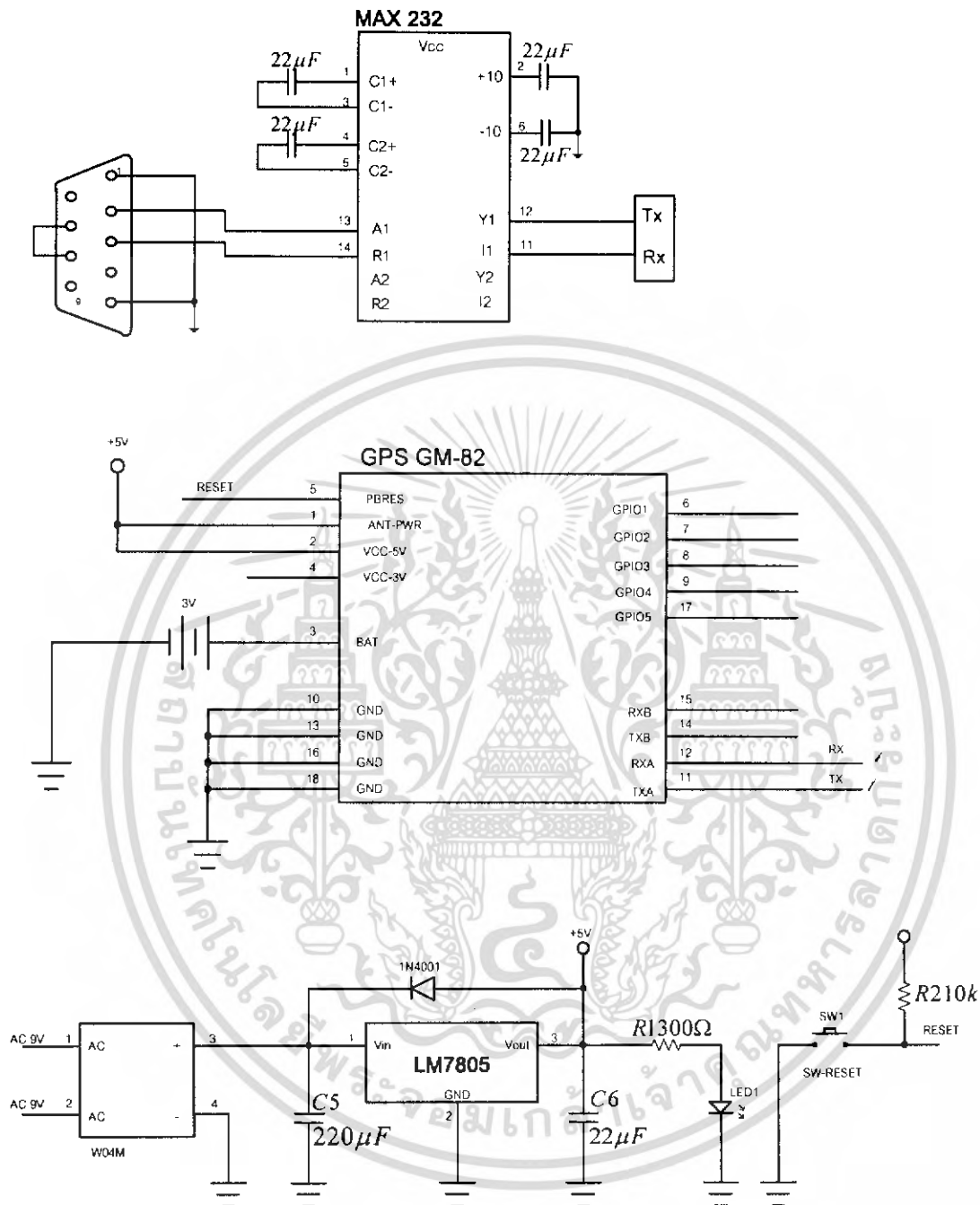
รูปที่ 3.3 วงจร Connect GPS Module
