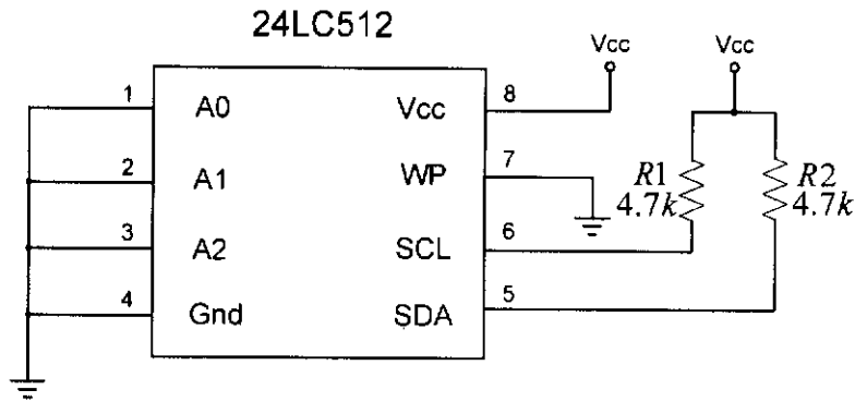
รูปที่ 3.6 วงจรหน่วยความจำอีสแควพรวม
