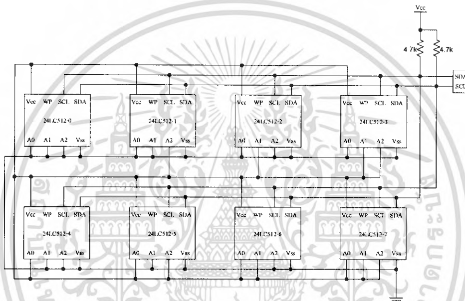
รูปที่ 3.7 วงจรหน่วยความจำอีสแควพรวมแบบหลายตัว
