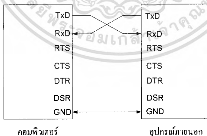
รูปที่ 2.19 การต่ออุปกรณ์ภายนอกเข้ากับคอมพิวเตอร์แบบ RS-232 โดยใช้สัญญาณเพียง3 เส้น
