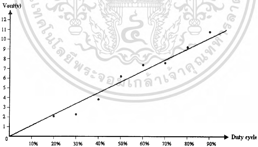
รูปที่ 4.3 กราฟแสดงความสัมพันธ์ระหว่าง ค่าตัวชี้ ไซเคิลแรงดันที่มอเตอร์
