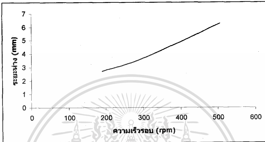
รูปที่ 4.7 แสดงกราฟผลการทดลองกับตัวกลางที่เป็นน้ำโดยมีภาระมากกระทำที่ 4 bar
