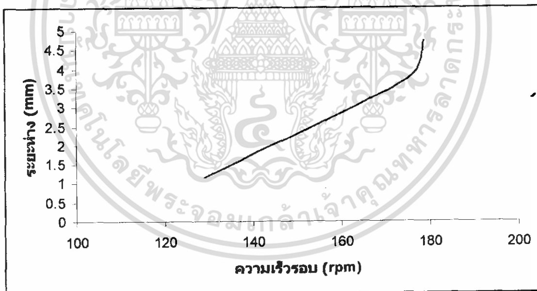
รูปที่ 4.5 แสดงกราฟผลการทดลองกับตัวกลางที่เป็นน้ำโดยมีภาระกระทำที่ 3 bar
