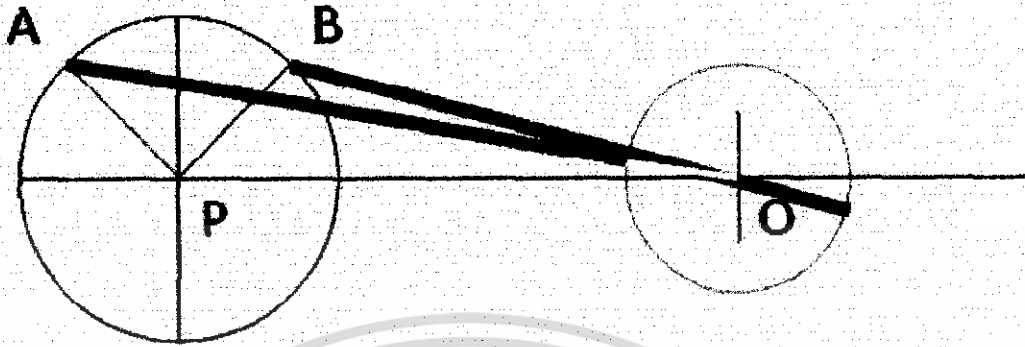
รูปที่ 2.5 แสดงการคำนวณหาความยาวแขนของ Four Bar Linkage จีนที่ 2 และ จีนที่ 3
