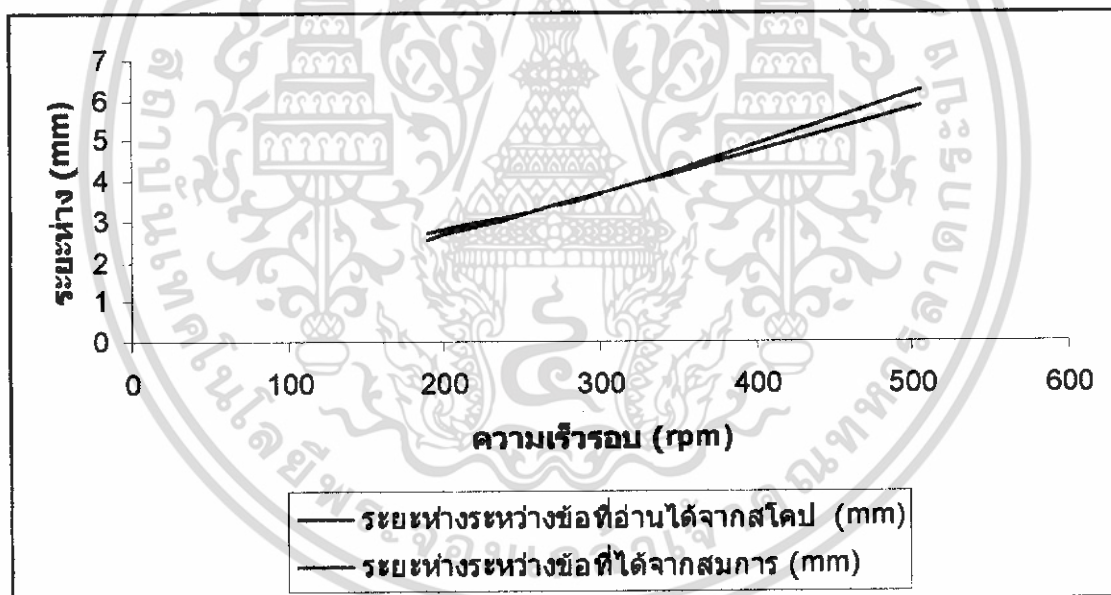
รูปที่ 4.8 แสดงกราฟผลการทดลองกับตัวกลางที่เป็นน้ำโดยมีภาระกระทำที่ 4 bar เปรียบเทียบกับผลของการตรวจสอบประสิทธิภาพการทำงานของเครื่องมือ โดยใช้ตัวกลางเป็นน้ำ
