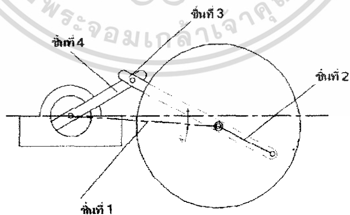
รูปที่ 2.3 แสดงหลักการการทำงานของ Four Bar Linkage
