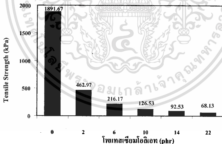
รูปที่ 4.4 ค่าต้านทานแรงดึงของโคมยางธรรมชาติที่ปริมาณโพแทสเซียมโอเลอเท 0, 2, 6, 10, 14 และ 22 phr
