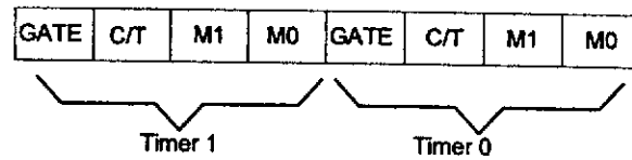
รูปที่ 2.27 โครงสร้างของ TMOD
