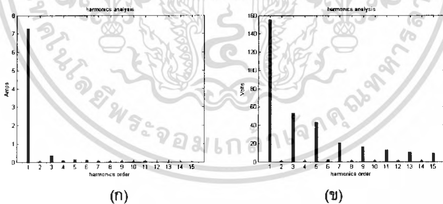
รูปที่ 6.13 ฮาร์โมนิกส์กระแสกับแรงดันที่ความถี่ 60 kHz และ Duty 50 %
