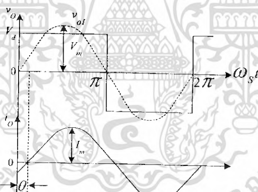
รูปที่ 3.7 คลื่นแรงดันและกระแสเอาต์พุตของวงจรฟูลบริดจ์อินเวอร์เตอร์เรโซแนนท์อนุกรม
