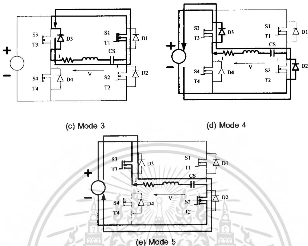
รูปที่ 2.9 โหมดการทำงานของวงจรฟูลบริดจ์อินเวอร์เตอร์ที่ควบคุมด้วยการปรับแรงดัน
