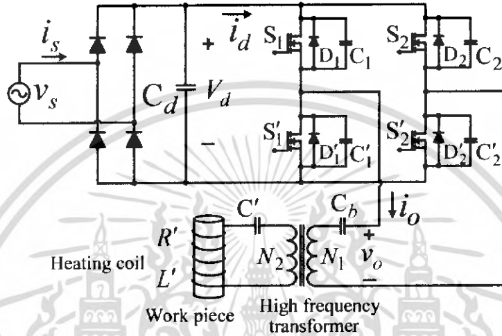
รูปที่ 3.3 โครงสร้างของวงจรฟูลบริดจ์อินเวอร์เตอร์เรโซแนนซ์อนุกรม
