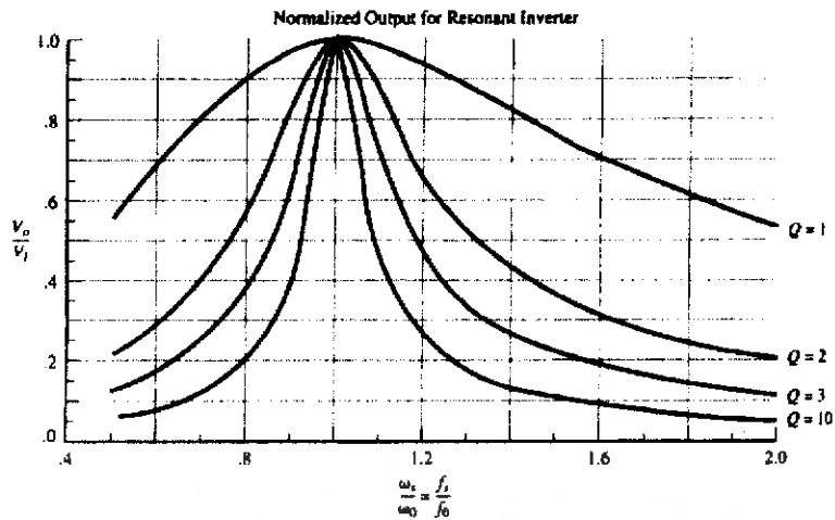
รูปที่ 3.1 วงจรอินเวอร์เตอร์เรโซแนนซ์แบบอนุกรม (ข) วงจรสมมูล R – L – C (ค) ค่าบรรทัดฐานของผลตอบสนองเชิงความถี่
