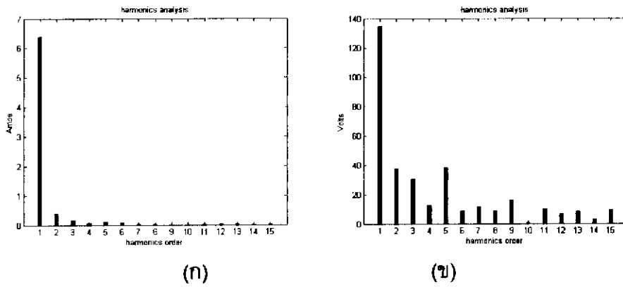
รูปที่ 6.11 ฮาร์โมนิกส์กระแสกับแรงดันที่ความถี่ 60 kHz และ Duty 22 %
