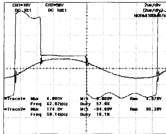
รูปที่ 6.6 เวก์พุทที่มีความถี่ 58 kHz โดยเปรียบเทียบกับขณะตัดสัญญาณพัลส์ทางซีกบวก
