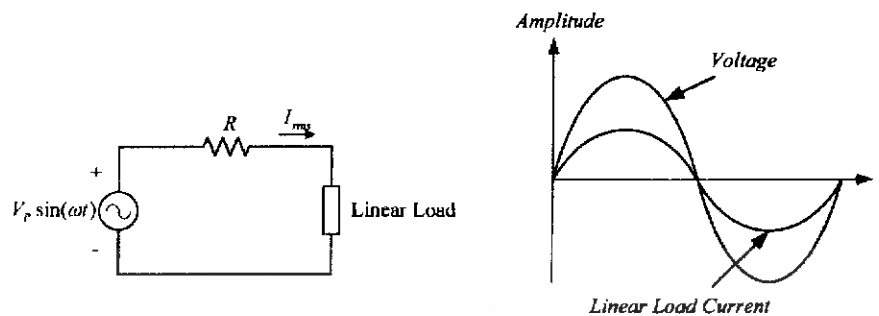
รูปที่ 4.2 จำลองสถานะที่การไฟฟ้าจ่ายพลังงานไฟฟ้าให้กับโหลดแบบเชิงเส้น
