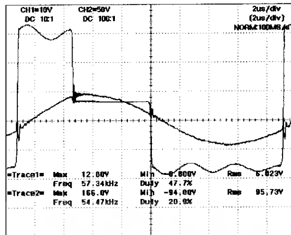
รูปที่ 6.7 เอาร์ทพุทที่ความถี่ 54 kHz โดยเปรียบเทียบกับขณะตัดสัญญาณพัลส์ทางซีกบวก
