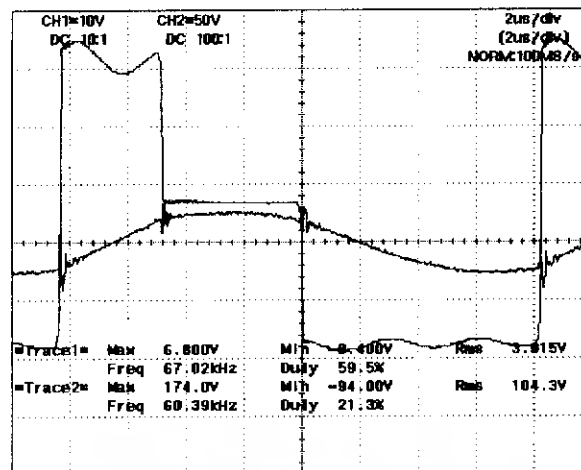
รูปที่ 6.5 เวก์พุกที่ความถี่ 60 kHz โดยเปรียบเทียบกับขณะตัดสัญญาณพัลส์ทางซีกบวก
