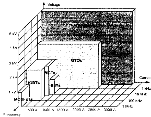
รูปที่ 2.10 ความสัมพันธ์ระหว่างความถี่ใช้งานกับพิกัดกำลังไฟฟ้าสำหรับอุปกรณ์สวิตซ์แต่ละชนิด
