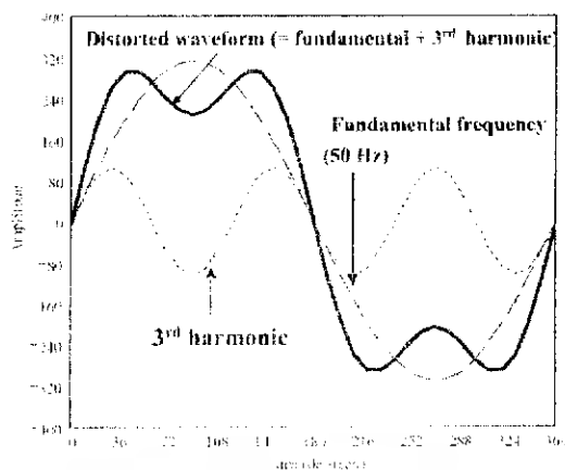
รูปที่ 4.1 รูปคลื่นที่ผิดเพี้ยนไปจากไซน์ซึ่งประกอบด้วยส่วนประกอบความถี่หลักมูล โดยมีฮาร์โมนิกที่ 3 และค่าความเพี้ยนฮาร์โมนิกส์รวม (THD) เท่ากับ 30%
