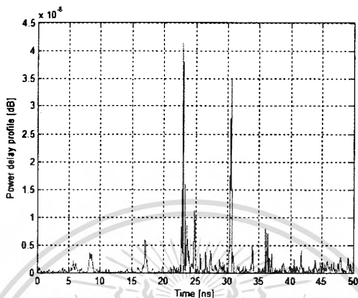
รูปที่ 4.2 (จ) ค่าของกำลังงานที่รับสัญญาณได้ในเวลาต่างๆ ขณะที่ระยะทางระหว่างสายอากาศทางด้านส่งและสายอากาศทางด้านรับห่างกัน 6.7 เมตร
