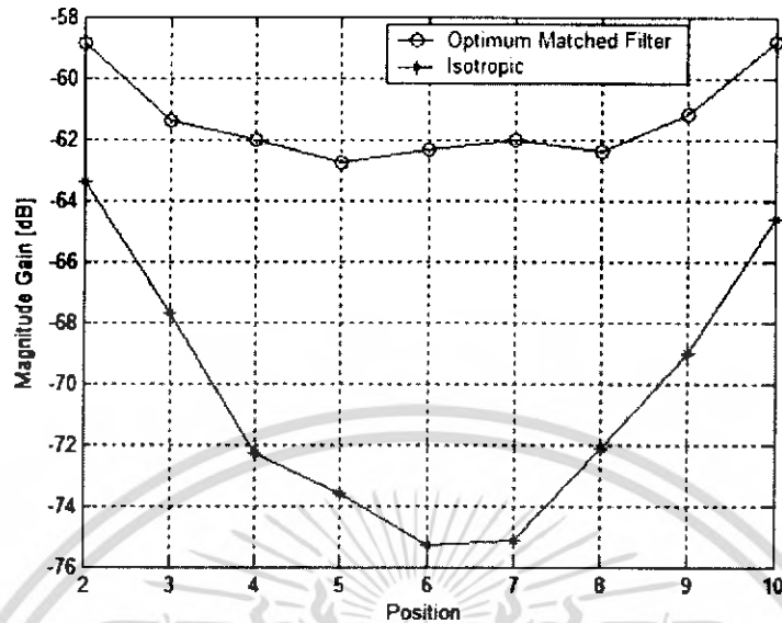
รูปที่ 4.7 (ข) ค่าความแตกต่างระดับการขยายขนาด กับ ไอโซโทปิก แมทฟิวเตอร์ที่ตำแหน่งต่างๆ
