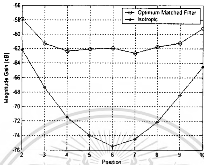
รูปที่ 4.8 (ซ) ค่าความแตกต่างระดับการขยายขนาด กับ ไอโซโทปิก แมทพิวเคอร์ที่ตำแหน่งต่างๆ
