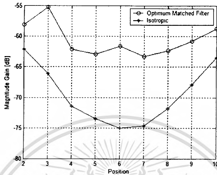
รูปที่ 4.9 (ข) ค่าความแตกต่างระดับการขยายขนาด กับ ไอโซโทปิก แมทฟิวเตอร์ที่ตำแหน่งต่างๆ
