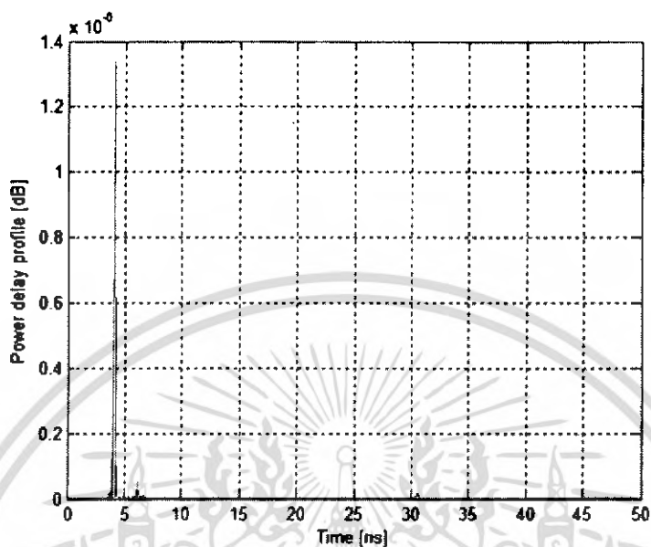
รูปที่ 4.4 (ง) ค่าของกำลังงานที่รับสัญญาณได้ในเวลาต่างๆ ขณะที่ระยะทางระหว่างสายอากาศทางด้านส่งและสายอากาศทางด้านรับห่างกัน 1 เมตร
