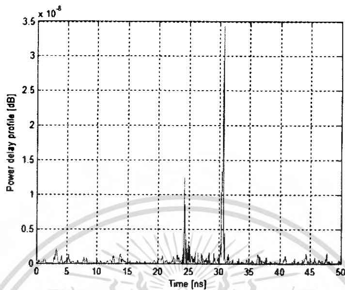
รูปที่ 4.10 (ฉ) ค่าของกำลังงานที่รับสัญญาณได้ในเวลาต่างๆ ขณะที่ระยะทางระหว่างสายอากาศทางด้านส่งและสายอากาศทางด้านรับห่างกัน 7.05 เมตร
