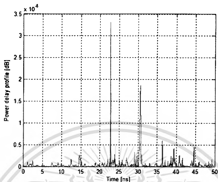
รูปที่ 4.3 (ข) ค่าของกำลังงานที่รับสัญญาณได้ในเวลาต่างๆ ขณะที่ระยะทางระหว่างสายอากาศทางด้านส่งและสายอากาศทางด้านรับห่างกัน 6.65 เมตร
