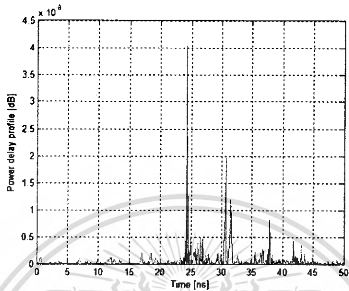
รูปที่ 4.9 (จ) ค่าของกำลังงานที่รับสัญญาณได้ในเวลาต่างๆ ขณะที่ระยะทางระหว่างสายอากาศทางด้านส่งและสายอากาศทางด้านรับห่างกัน 7.05 เมตร
