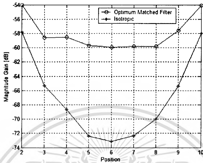
รูปที่ 4.2 (ข) ค่าความแตกต่างระดับการขยายขนาดกับ ไอโซโทปิก แมทฟิวเตอร์ที่ตำแหน่งต่างๆ
