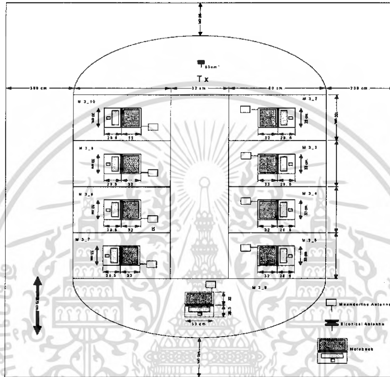
รูปที่ 3.14 (ก) รูปแบบ โมเดล1 กรณีที่ 2.1,2.2
