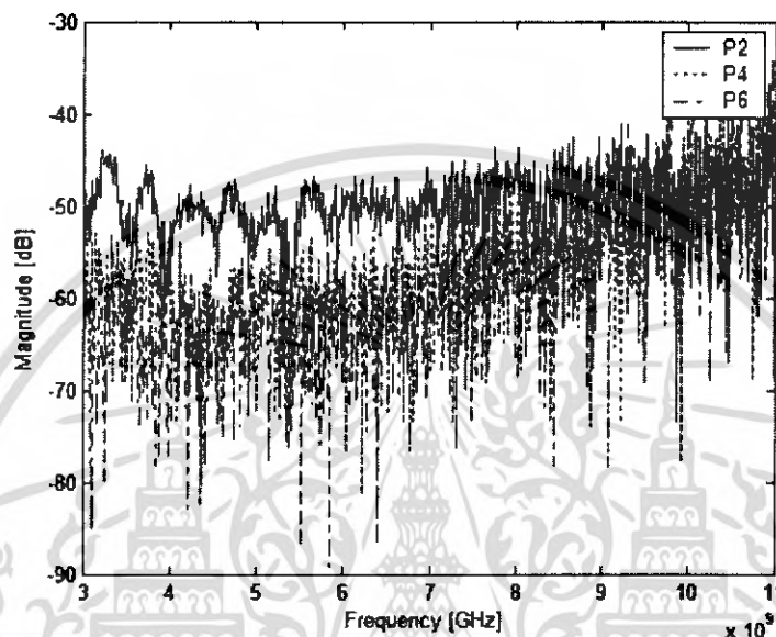
รูปที่ 4.4 (จ) ความสัมพันธ์ระหว่าง แม็กนิจูด กับ ความถี่
