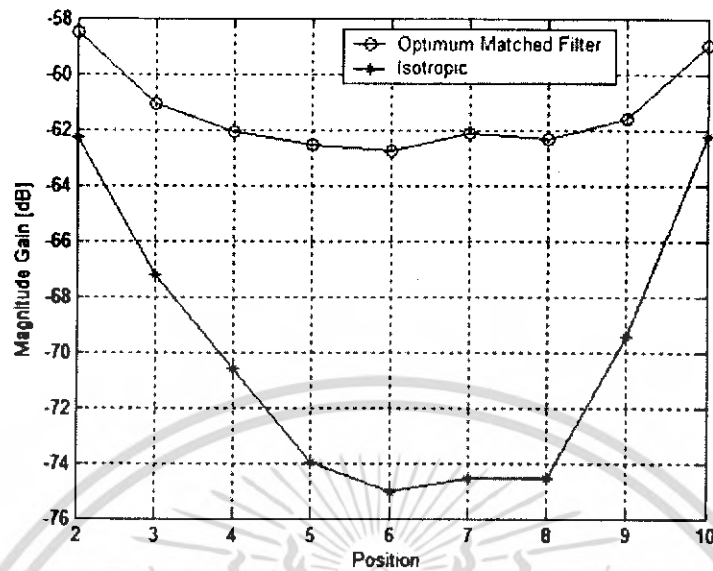
รูปที่ 4.10 (ข) ค่าความแตกต่างระดับการขยายขนาด กับ ไอโซโทปิก แมทฟิวเตอร์ที่ตำแหน่งต่างๆ
