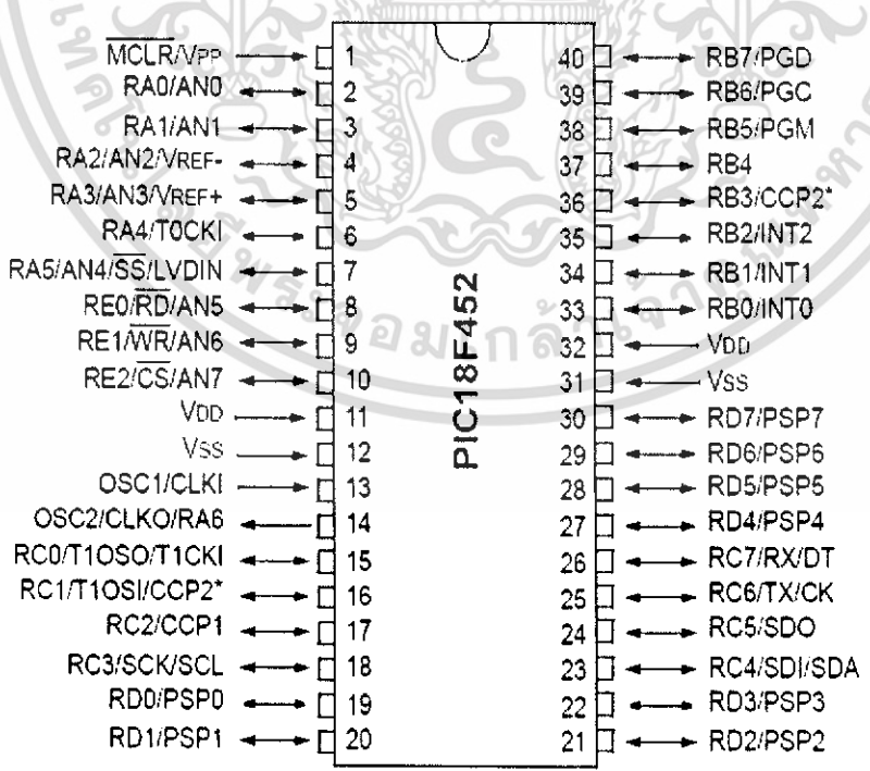
รูปที่ 3.2 แสดงไดอะแกรมของ PIC18F452
