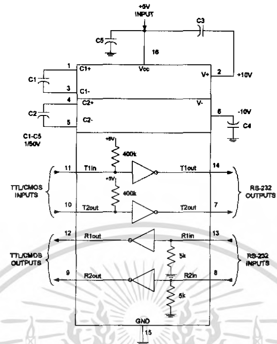
รูปที่ 2.4 โครงสร้างภายในของ MAX232 หรือ ICL232
