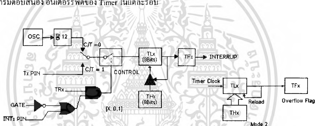
รูปที่ 2.2 แสดงการทำงานของ Timer/counter ในโหมด 2 (8 bit Auto reload)
