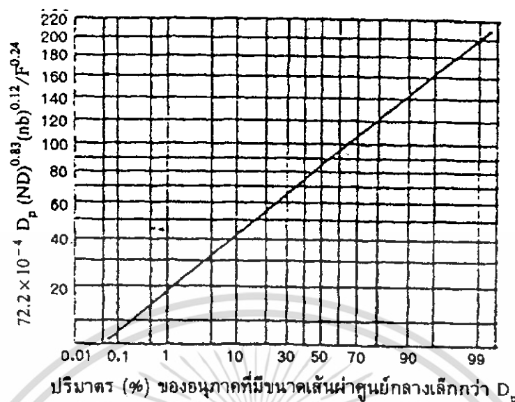
รูปที่ 2.6 ความสัมพันธ์ระหว่างเส้นผ่านศูนย์กลางของหยดของเหลวกับปริมาตรที่ฟุ้งฝอย [1]
