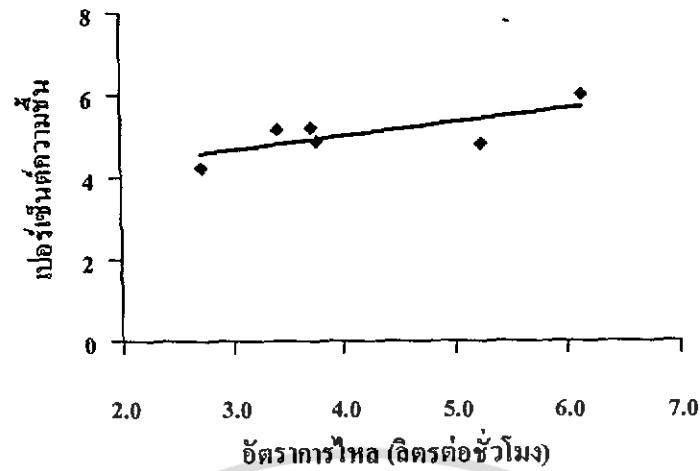
รูปที่ 6.1 ความสัมพันธ์ของอัตราการไหลกับเปอร์เซ็นต์ความชื้นของผลิตภัณฑ์ ที่อุณหภูมิต่ำ 175 องศาเซลเซียส ความเร็วของอากาศขาเข้า 4.8 เมตรต่อวินาที
