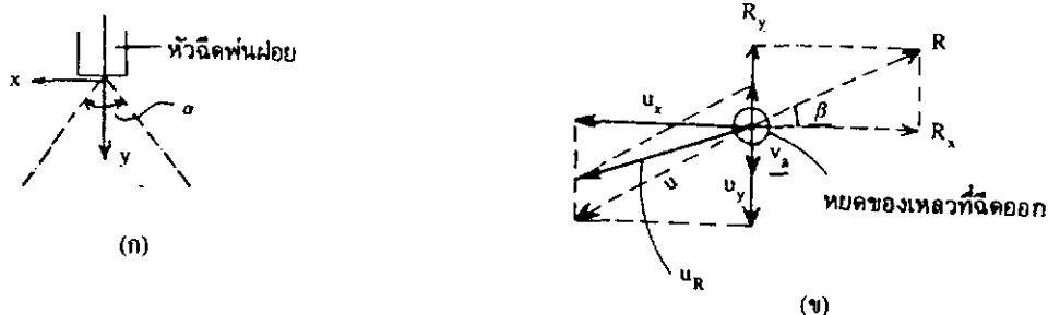
รูปที่ 2.8 แบบจำลองสำหรับคำนวณเส้นโคจรของหยดของเหลวที่พ่นฝอยโดยหัวฉีดด้วยความดัน
