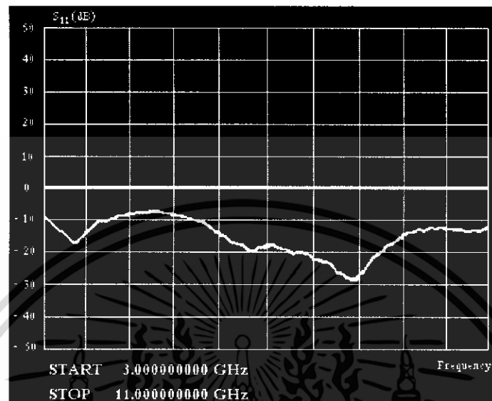
รูปที่ 4.5 ค่า S_{11} ของสายอากาศแบบจานกรวยขนาดเส้นผ่านศูนย์กลางกรวย 67.5 มิลลิเมตร และเส้นผ่านศูนย์กลางแผ่นจาน 67.5 มิลลิเมตร
