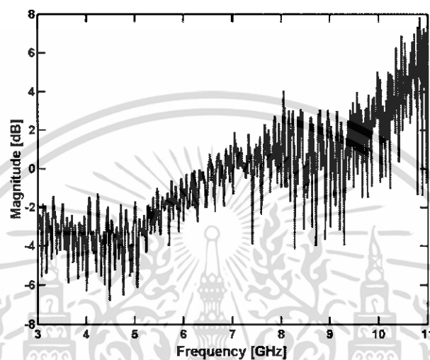
รูปที่ 4.19 ค่า Magnitude ของสายอากาศรวยคู่
