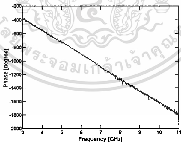
รูปที่ 4.20 ค่า Phase ของสายอากาศรวยคู่
