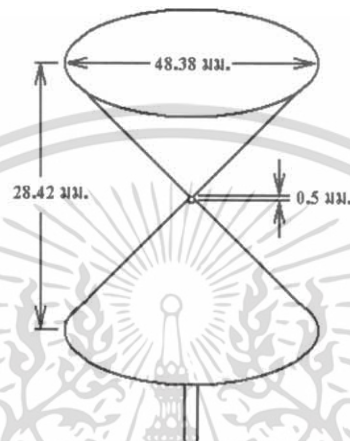
รูปที่ 3.5 แบบสายอากาศกรวยคู่ที่ทำการออกแบบ
