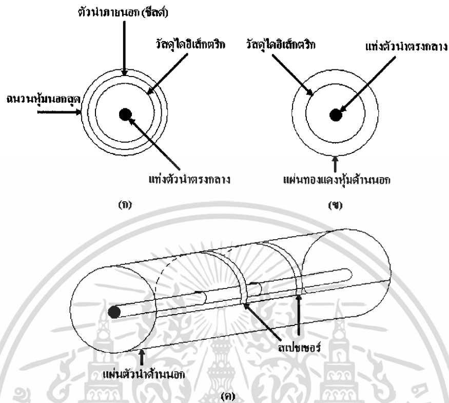
รูปที่ 2.22 (ก) สายแบบสามารถงอได้ (Flexible), (ข) แบบกึ่งแข็ง (Semirigid), (ค) แบบแข็ง (Rigid)
