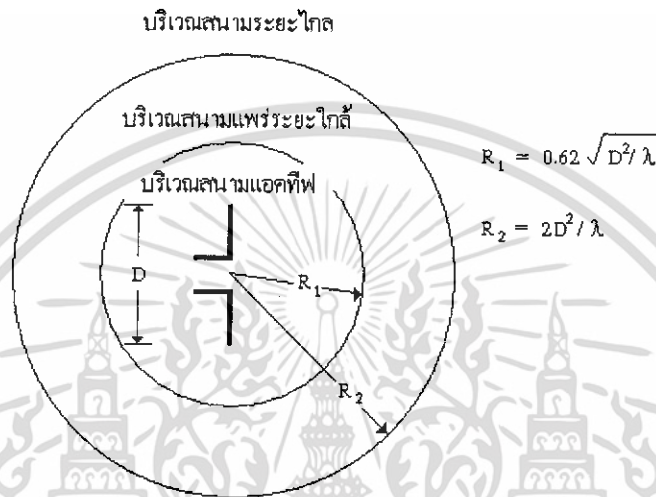
รูปที่ 2.11 การแบ่งบริเวณของสนามจากสายอากาศ
