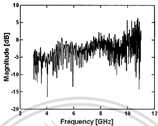
รูปที่ 4.21 ค่า Magnitude ของสายอากาศแบบจานกรวย
