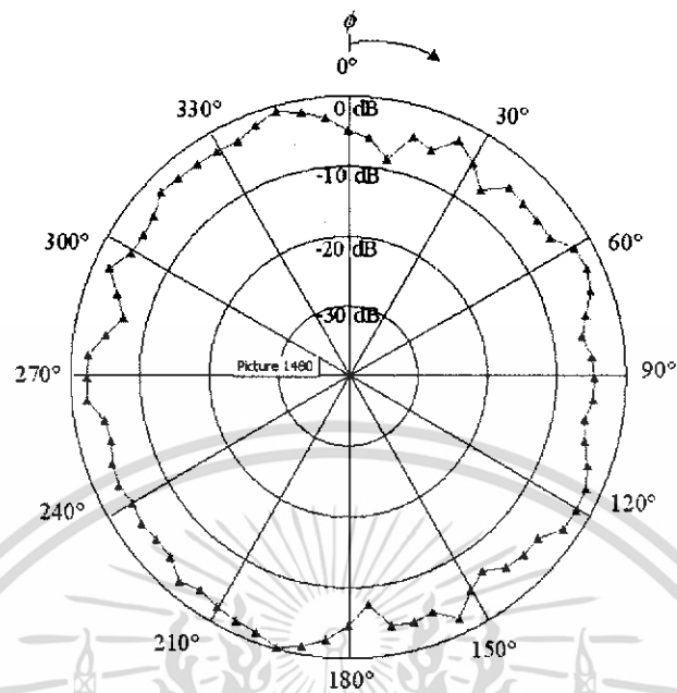
รูปที่ 4.31 รูปแบบการแพร่กระจายคลื่นของสายอากาศสี่เหลี่ยมคางหมู
