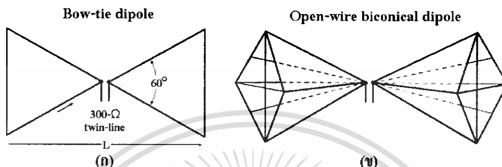
รูปที่ 2.21 สายอากาศ Bow-tie แบบแผ่น (ก) และสายอากาศไดโพลโครงสร้างกรวยแบบสายเปิด (ข)
