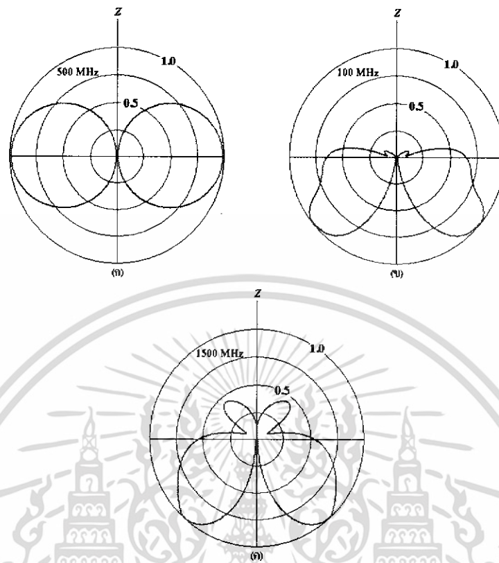
รูปที่ 2.20 แพทเทอรันการวัดของสายอากาศแบบจานกรวย
