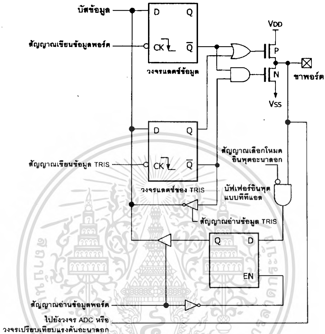
รูปที่ 2-31 โครงสร้างขา RA0-RA3 ของพอร์ต A
