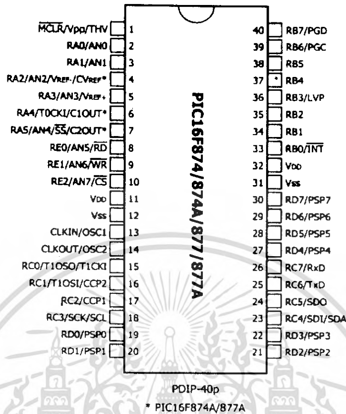
รูปที่ 2-22 การจัดขาไมโครคอนโทรลเลอร์ PIC 16F877A
