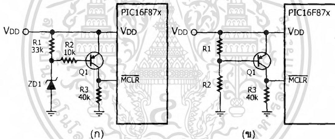
รูปที่ 2-30 ตัวอย่างการต่อวงจรบรรเทาเอาต์พุตที่เก็ทเข้าที่ขา \overline{MCLR} ในกรณีที่ผู้ใช้ไม่เลือกใช้ความสามารถของวงจรบรรเทาเอาต์พุตที่เก็ทภายในไมโครคอนโทรลเลอร์
