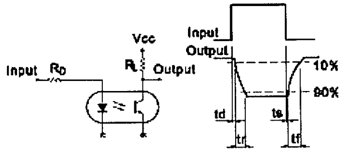
รูปที่ 2-40 การหน่วงสัญญาณของ Photocoupler LTV-847
