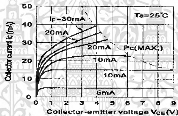
รูปที่ 2-37 ความสัมพันธ์ระหว่าง Ic และ Vce
