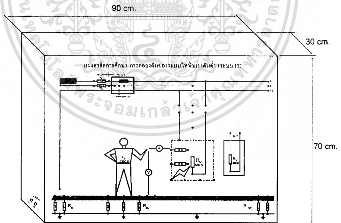
รูปที่ 3.3 แผนผังการศึกษาการต่อลงดินของระบบไฟฟ้าแรงดันต่ำ (ระบบ IT)
