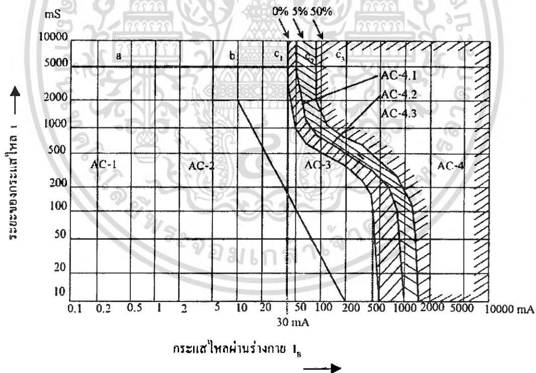
รูปที่ 2.1 โชนของเวลา/กระแสของผลของกระแสไฟฟ้าสลับความถี่ระหว่าง 15 Hz ถึง 100 Hz ที่ไหลจากมือซ้ายไปยังเท้าทั้งสอง(ที่มา : IEC 60479 -1 ) [2]
