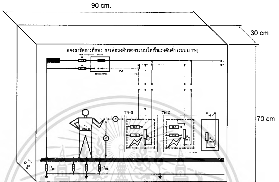
รูปที่ 3.2 แผนผังการศึกษาการต่อลงดินของระบบไฟฟ้าแรงดันต่ำ (ระบบ TN)
