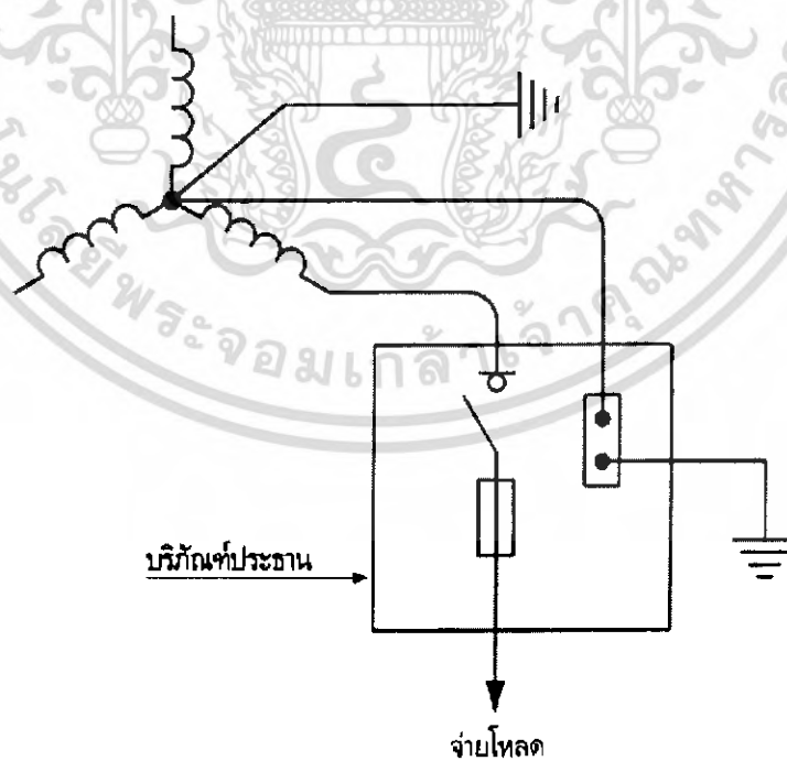
รูปที่ 2.13 หม้อแปลงที่มีการต่อลงดินต้องเดินสายที่มีการต่อลงดินมายังบริเวณที่ประธานด้วย
