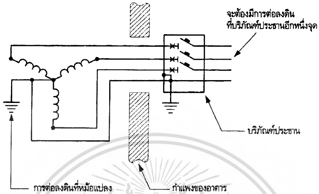
รูปที่ 2.15 การต่อลงดินที่หม้อแปลงนอกอาคารและที่บริการณ์ประธาน
