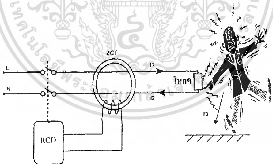
รูปที่ 2.3 เมื่อกระแสไม่สมดุล RCD จะทำงาน
