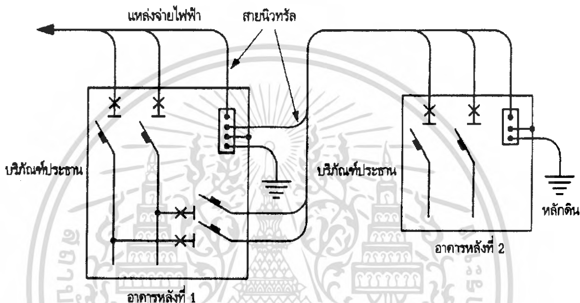
รูปที่ 2.18 อาคารแต่ละหลังต้องมียุทธดินเป็นของตัวเอง
