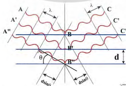
รูปที่ 2.10 แสดงหลักการเลี้ยวเบนของรังสีเอ็กซ์ [58]
