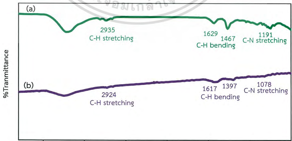
เอกสารนี้เป็นเอกสารที่สงวนไว้สำหรับการใช้งานเพื่อการศึกษาเท่านั้น ไม่อนุญาตให้นำไปใช้ประโยชน์ด้านกำไร ไม่ว่ากรณีใดๆ ทั้งสิ้น อีกทั้งห้ามมิให้ดัดแปลงเนื้อหา และเผยแพร่ไปยังเจ้าของเอกสารทุกครั้งที่มีการนำไปใช้ รูปที่ 4.11 สเปกตรัม FT-IR ของ (a) PDADMAC (b) AuNPs-PDADMAC
