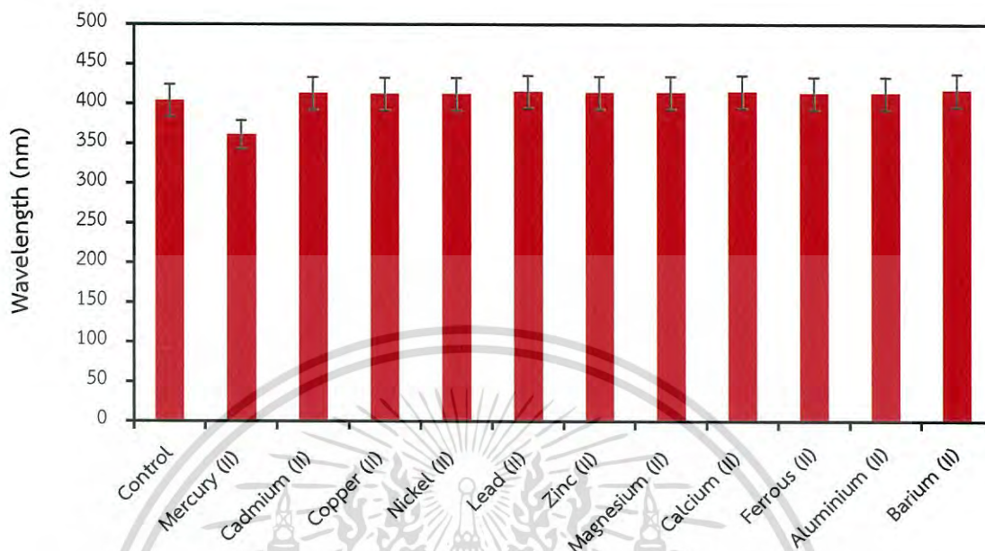
รูปที่ 4.35 ค่าความยาวคลื่นสูงสุดของตัวรบกวนต่างๆ ที่เติมลงไปในสารละลาย Au-Ag BNPs
