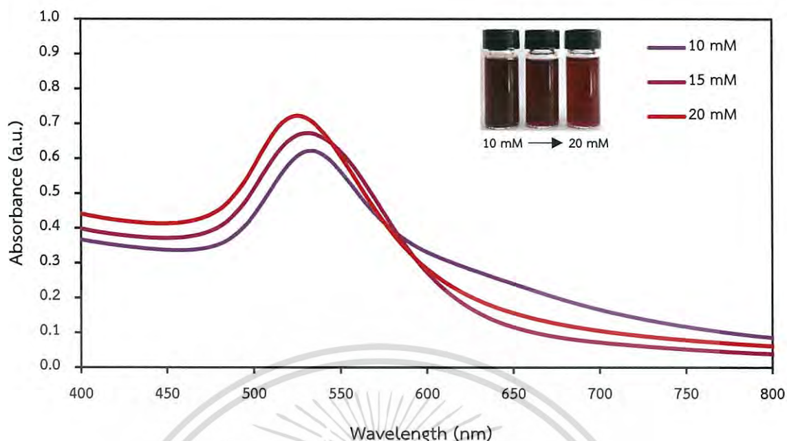
รูปที่ 4.3 ค่าการดูดกลืนแสงของสารละลาย AuNPs ที่สังเคราะห์ด้วยสารละลายไตรโซเดียมซิเตรท ความเข้มข้น 10 15 และ 20 mM
