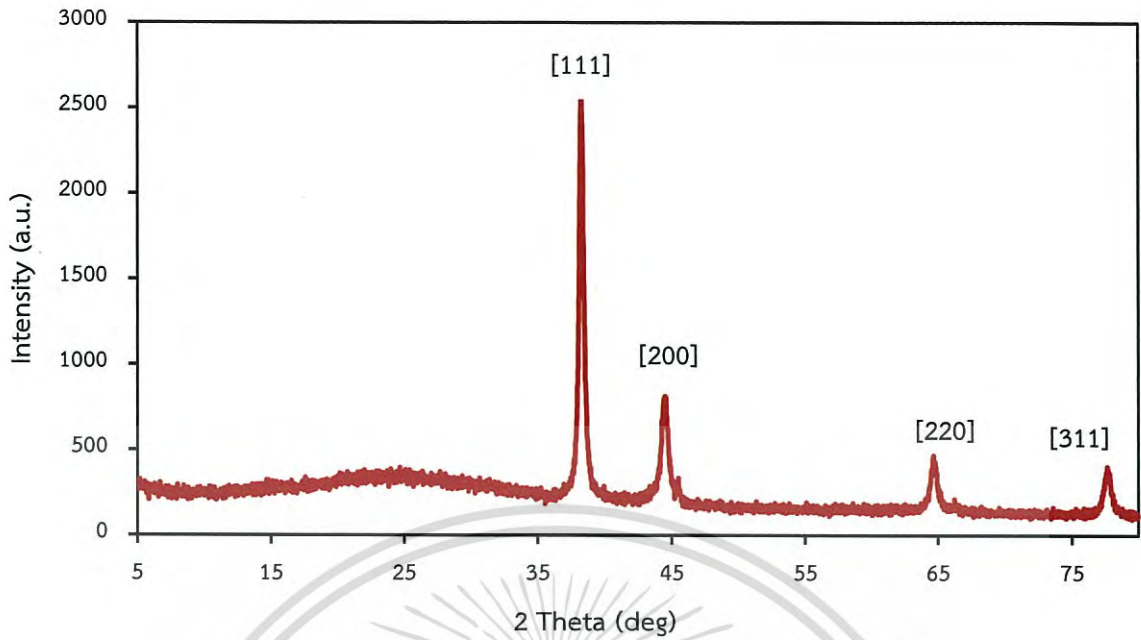
รูปที่ 4.6 ผลการวิเคราะห์โครงสร้างผลึกของ AuNPs ด้วยเครื่อง XRD
