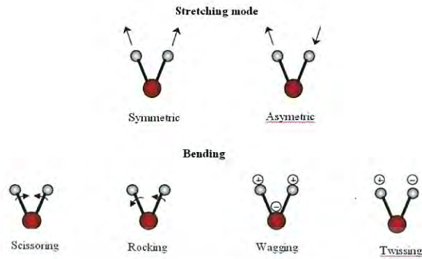
รูปที่ 2.9 ลักษณะการสั่นในโมเลกุลของสาร [57]
