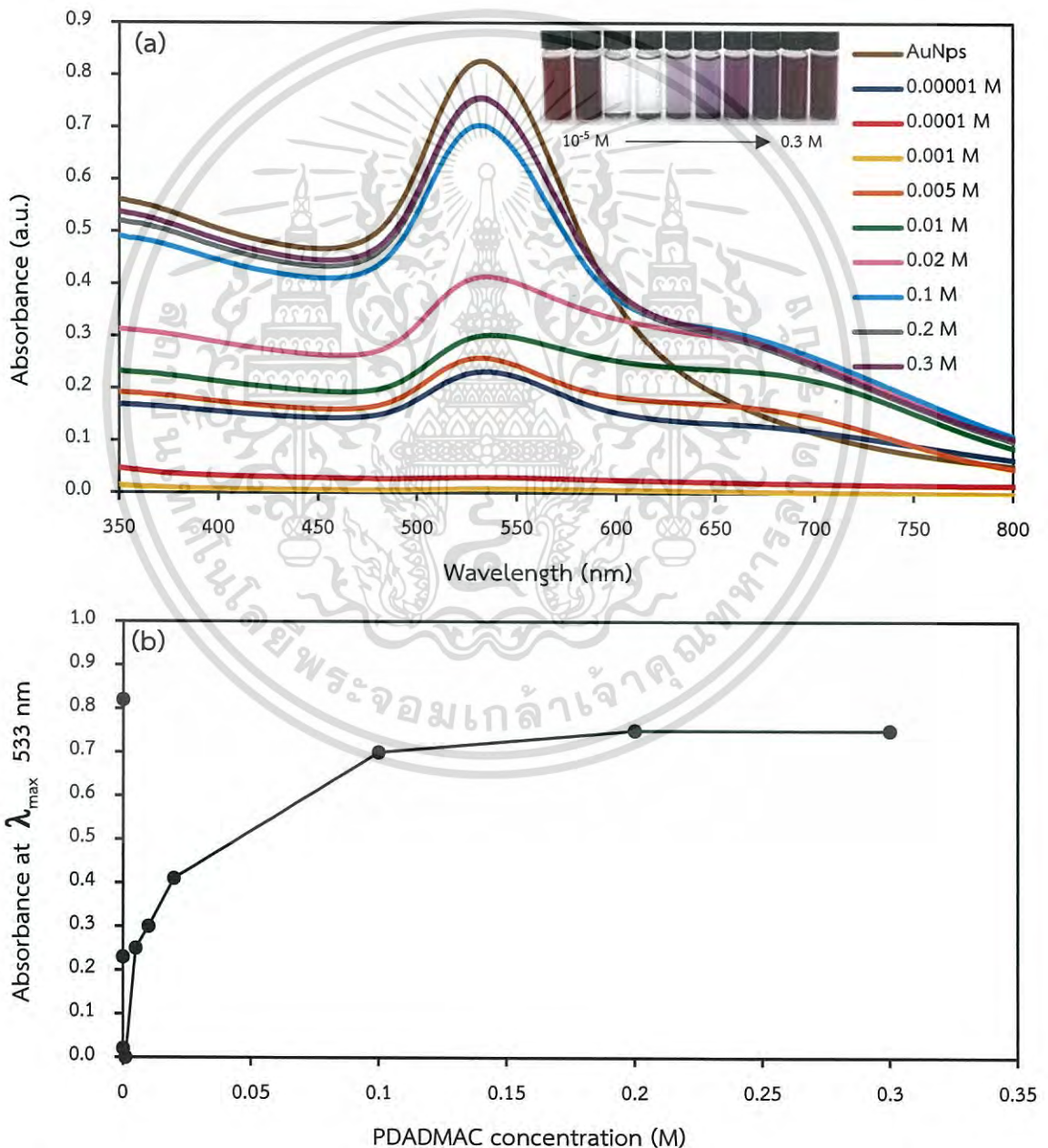
รูปที่ 4.8 (a) สเปกตรัมการดูดกลืนแสงของ AuNPs-PDADMAC (b) ค่าการดูดกลืนแสงที่ความยาวคลื่น 533 nm ของ AuNPs-PDADMAC
