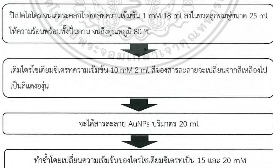
รูปที่ 3.1 แผนผังวิธีการสังเคราะห์ AuNPs ด้วยไตรโซเดียมซิเตรทความเข้มข้น 10 15 และ 20 mM
