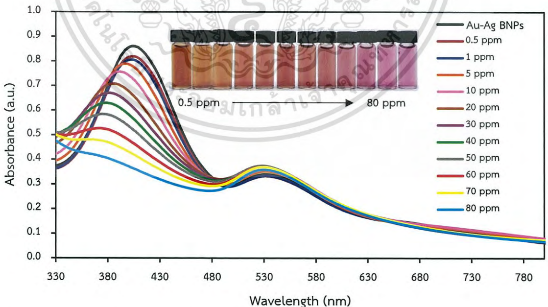
รูปที่ 4.26 ค่าการดูดกลืนแสงของ Au-Ag BNPs ที่ใช้เป็นตัวรับรู้เชิงสีในการวิเคราะห์ปรอทความเข้มข้น 0.5 ถึง 80 ppm
