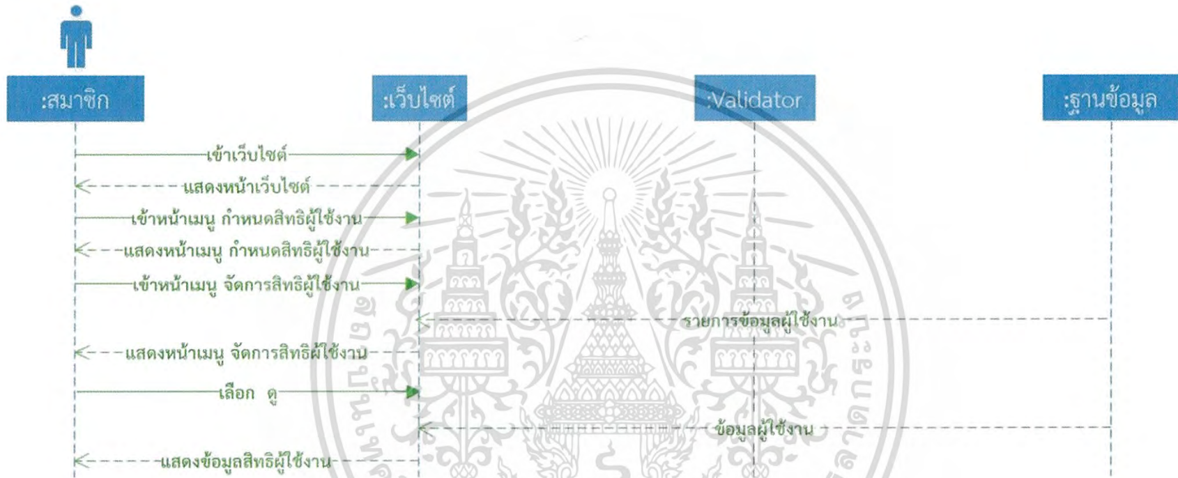
รูปที่ 3.96 Sequence Diagram แสดงการดูสิทธิ
