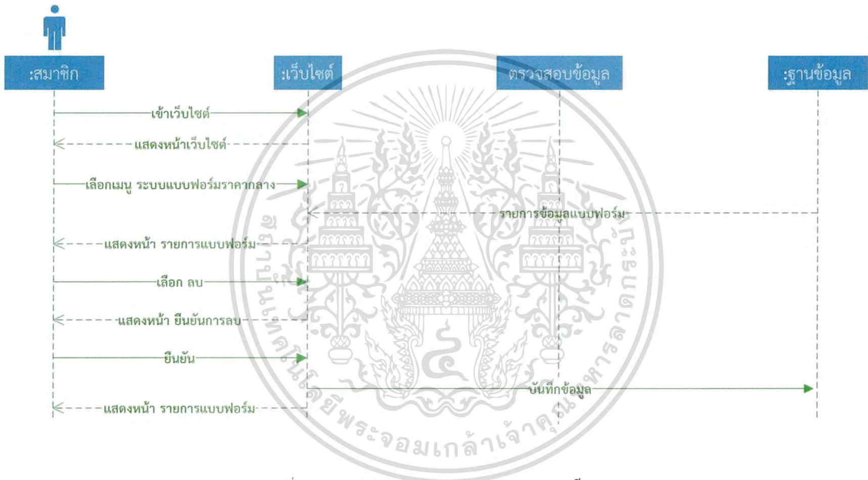
รูปที่ 3.101 Sequence Diagram แสดงการลบกฎระเบียบ
