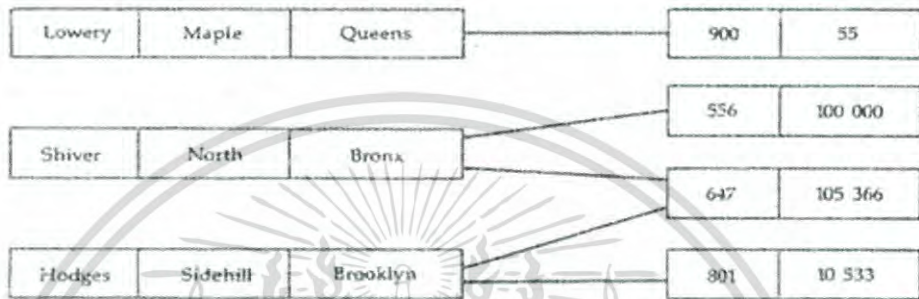
รูปที่ 2.2 ตัวอย่างข้อมูลที่มีความสัมพันธ์ระหว่างข้อมูลเป็นแบบโครงข่าย
