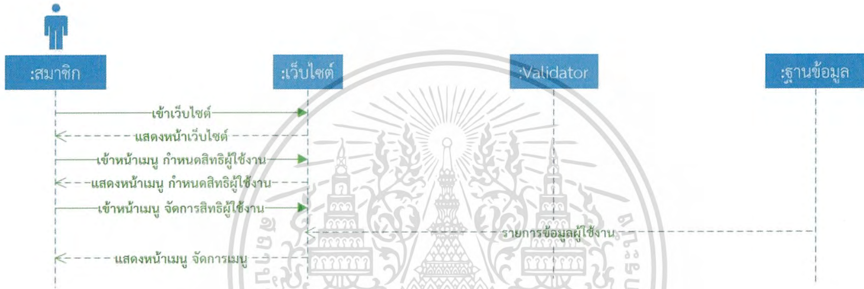
รูปที่ 3.92 Sequence Diagram แสดงการดูเมนู
