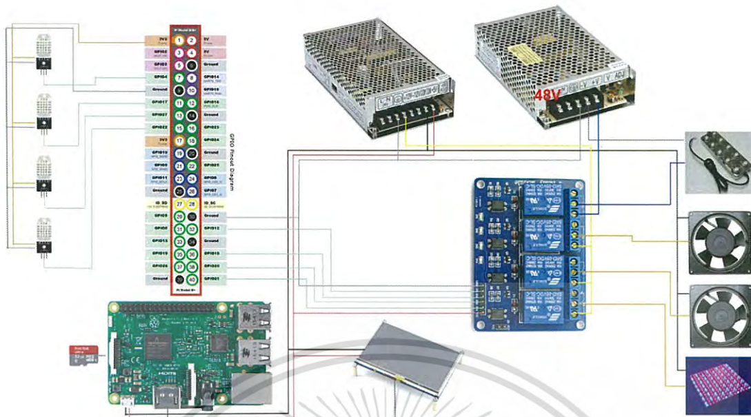
รูป 3.2 Hardware I/O Diagram
