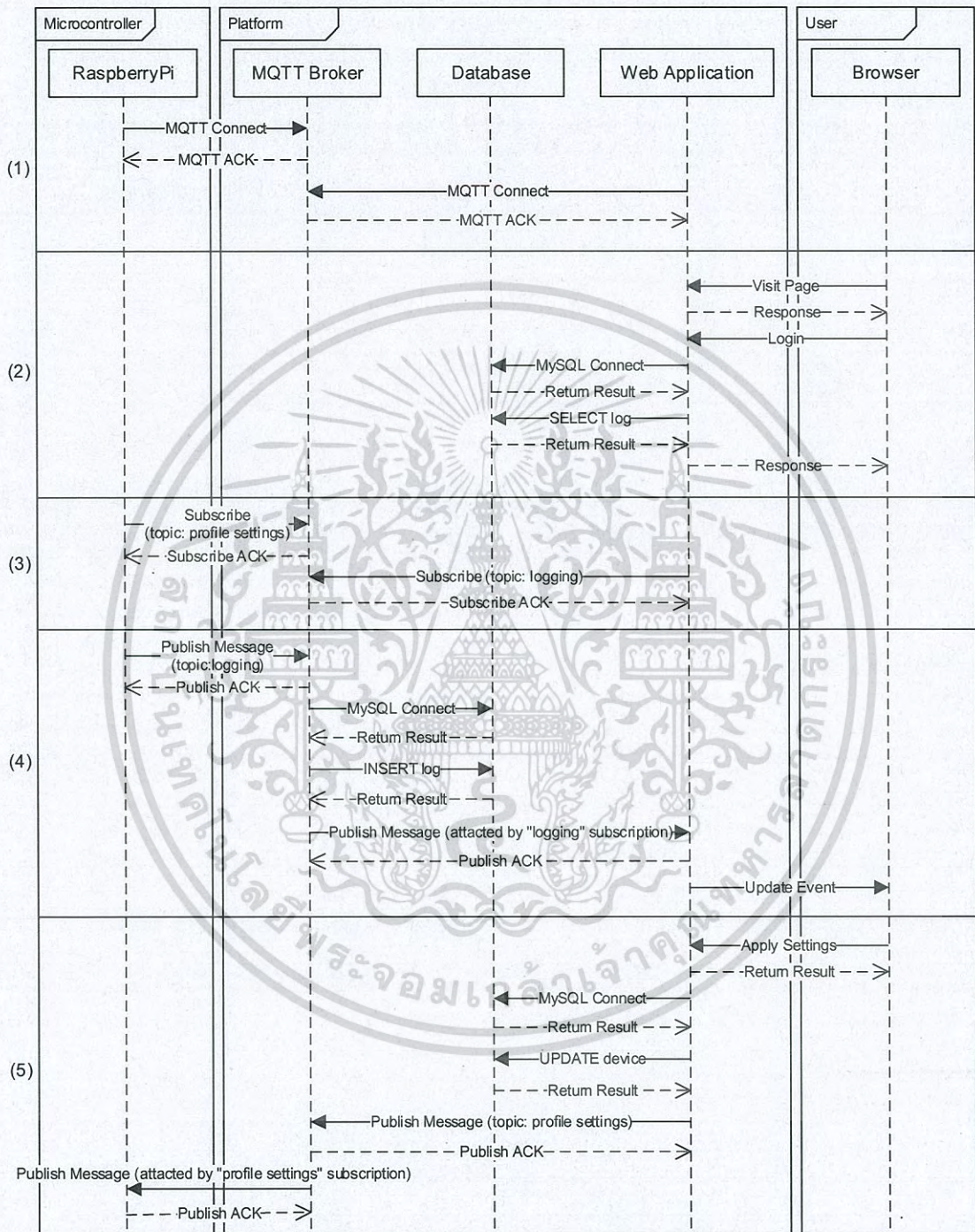
รูป 3.3 Sequence Diagram
