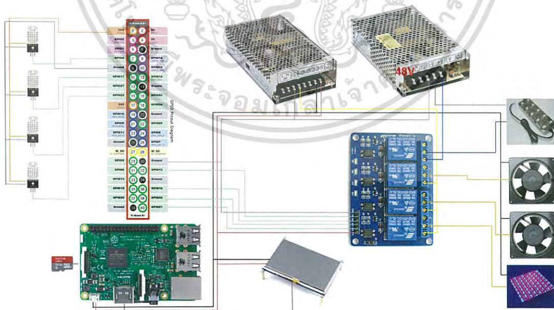
รูป 1.3 Hardware I/O Diagram
