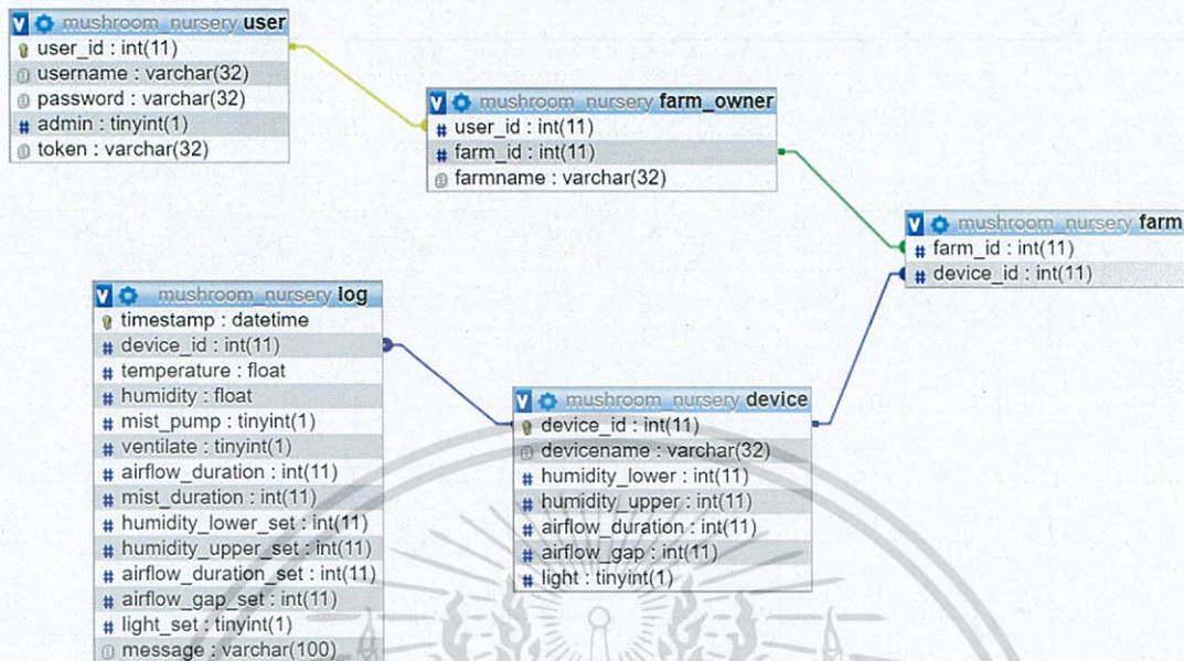
รูป 3.5 Database Schema
