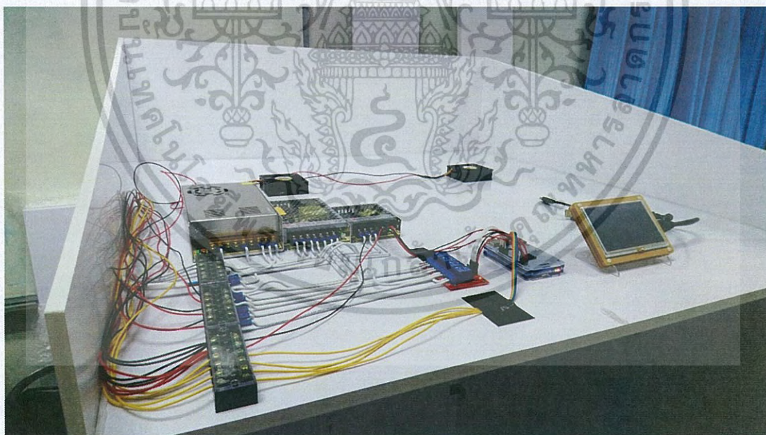
รูป 4.2 ส่วนแผงควบคุม
