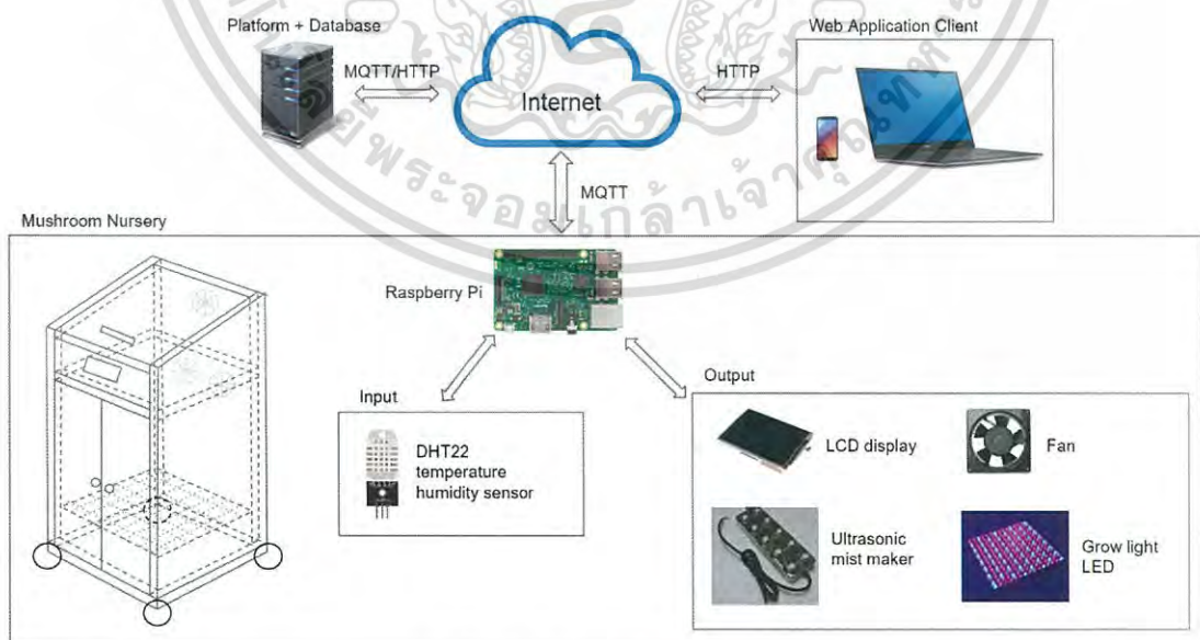
รูป 3.1 System Diagram
