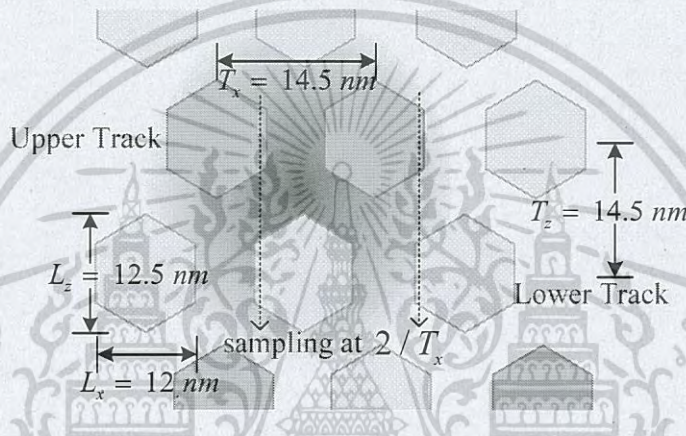
รูปที่ 3.1 สื่อบันทึกแบบเฮกซะโกนอล ที่ความหนาแน่นเชิงพื้นที่ 3.0 \text{ Tb/in}^2
