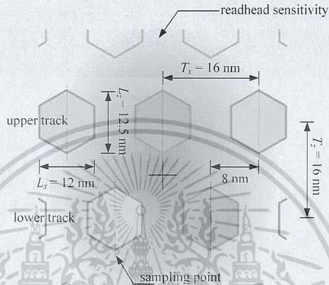
รูปที่ 2.13 ตัวอย่างบิตแพทเทิร์นมีเดียกริดแบบเยื้องที่ 2.5 Tb/in 2 ถูกปกคลุมด้วยผลตอบสนองความไวของหัวอ่าน [13]
