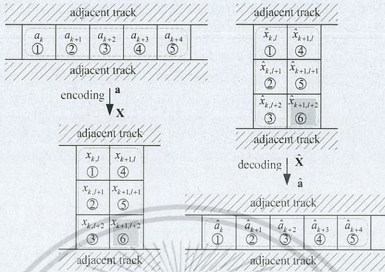
รูปที่ 2.11: วิธีการเข้ารหัสข้อมูลด้วยรหัสมอดดูเลขชั้นแบบสองมิติด้วยอัตราหัส 5/6
