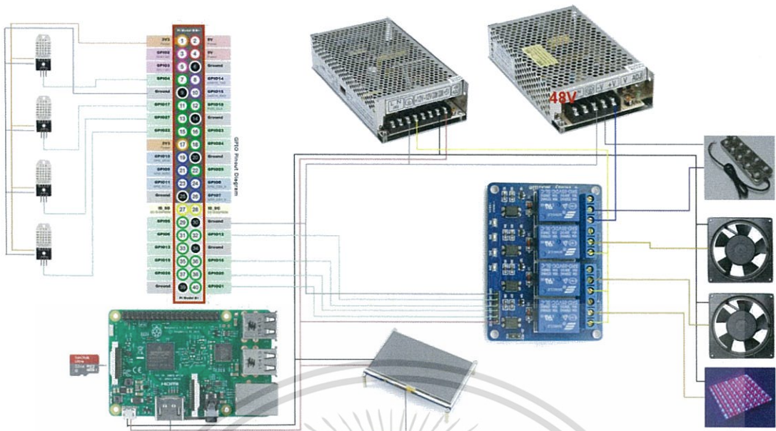
รูป 1.3 Hardware I/O Diagram
