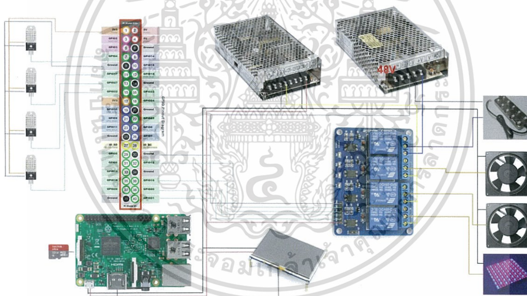
รูป 3.2 Hardware I/O Diagram
