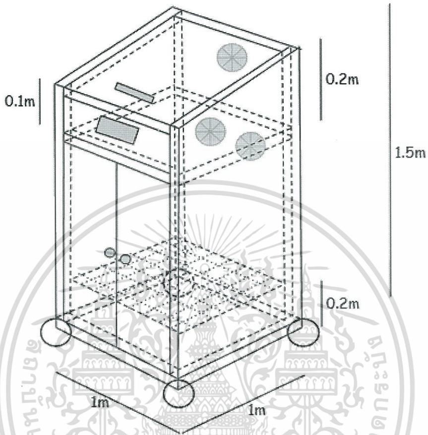
รูป 1.2 Model ตู้จำลองโรงเรียนเพาะเห็ด
