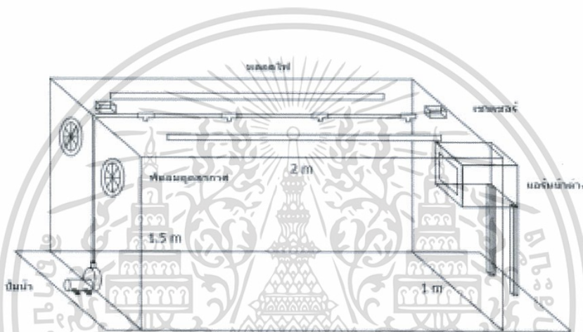
รูป 2.9 รายละเอียดของส่วนประกอบภายในโรงเรือนจำลอง
