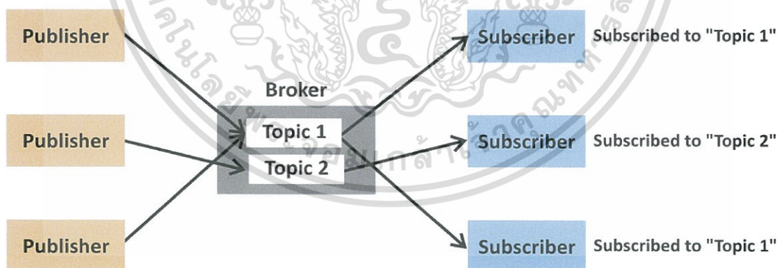
รูป 2.7 MQTT
