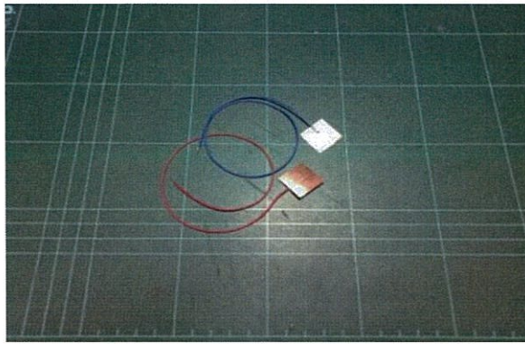
รูปที่ 3.14 แผ่นทองแดงที่บัดกรีสายไฟลงบนแผ่นทองแดงบางสองหน้าด้านใดด้านหนึ่ง
