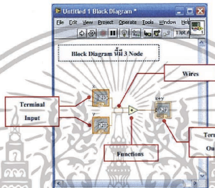
รูปที่ 2.27 ตัวอย่าง Terminal ใน LabVIEW
