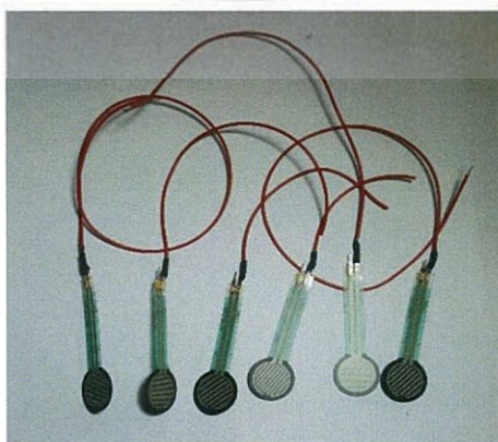
รูปที่ 3.33 การบัดกรีสายไฟเลี้ยงกับเซนเซอร์
