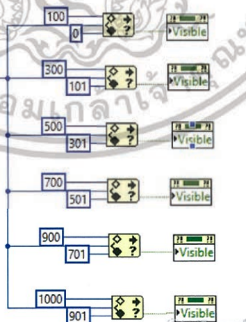
รูปที่ 3.66 การเลือกช่วงการทำงานให้กับบูลีน
