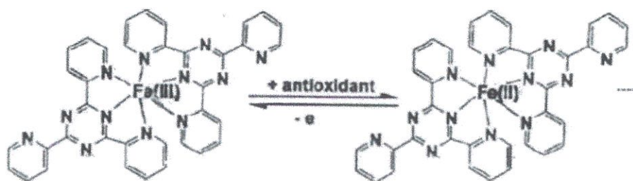
รูปที่ 2.4 ปฏิกริยาของ FRAP assay
