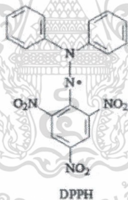
รูปที่ 2.5 สูตรโครงสร้างของ 2,2-diphenyl-1-picrylhydrazyl radical (DPPH radical)
