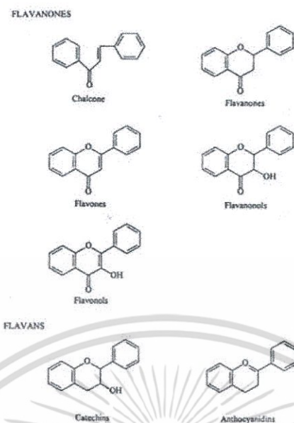
รูปที่ 2.10 โครงสร้างของสารประกอบกลุ่มฟลาโวนอยด์
