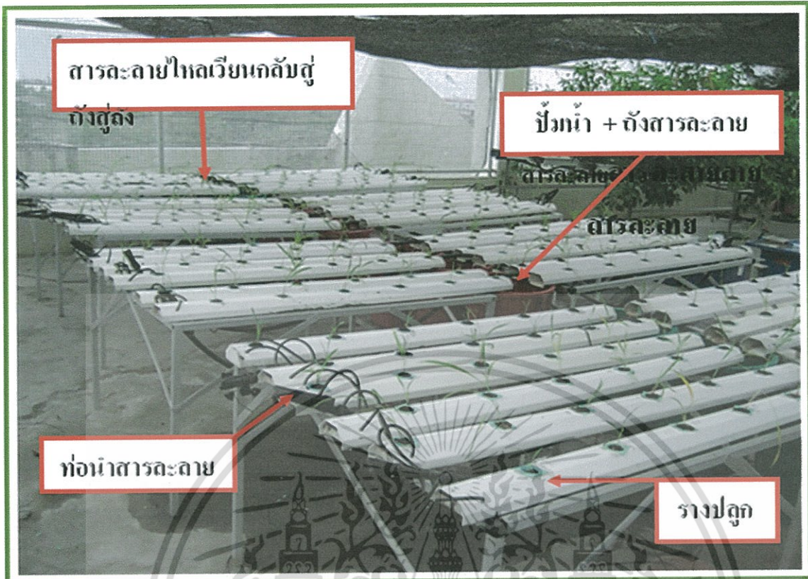
ภาพที่ 5 การหมุนเวียนของสารละลายธาตุอาหารพืชในระบบ NFT
