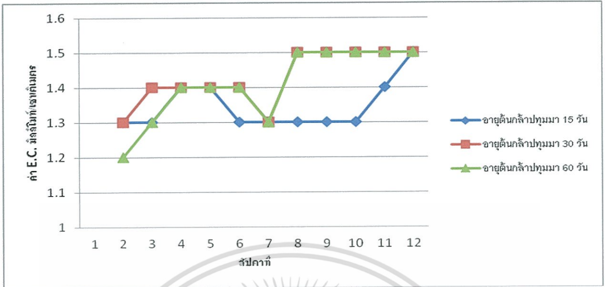
ภาพที่ 14 ค่า E.C. ที่ลดลงใน 12 สัปดาห์ (โดยปรับค่า E.C. ในน้ำเท่ากับ 1.5 มิลลิเมตร/เซนติเมตร ทุกๆ สัปดาห์)
