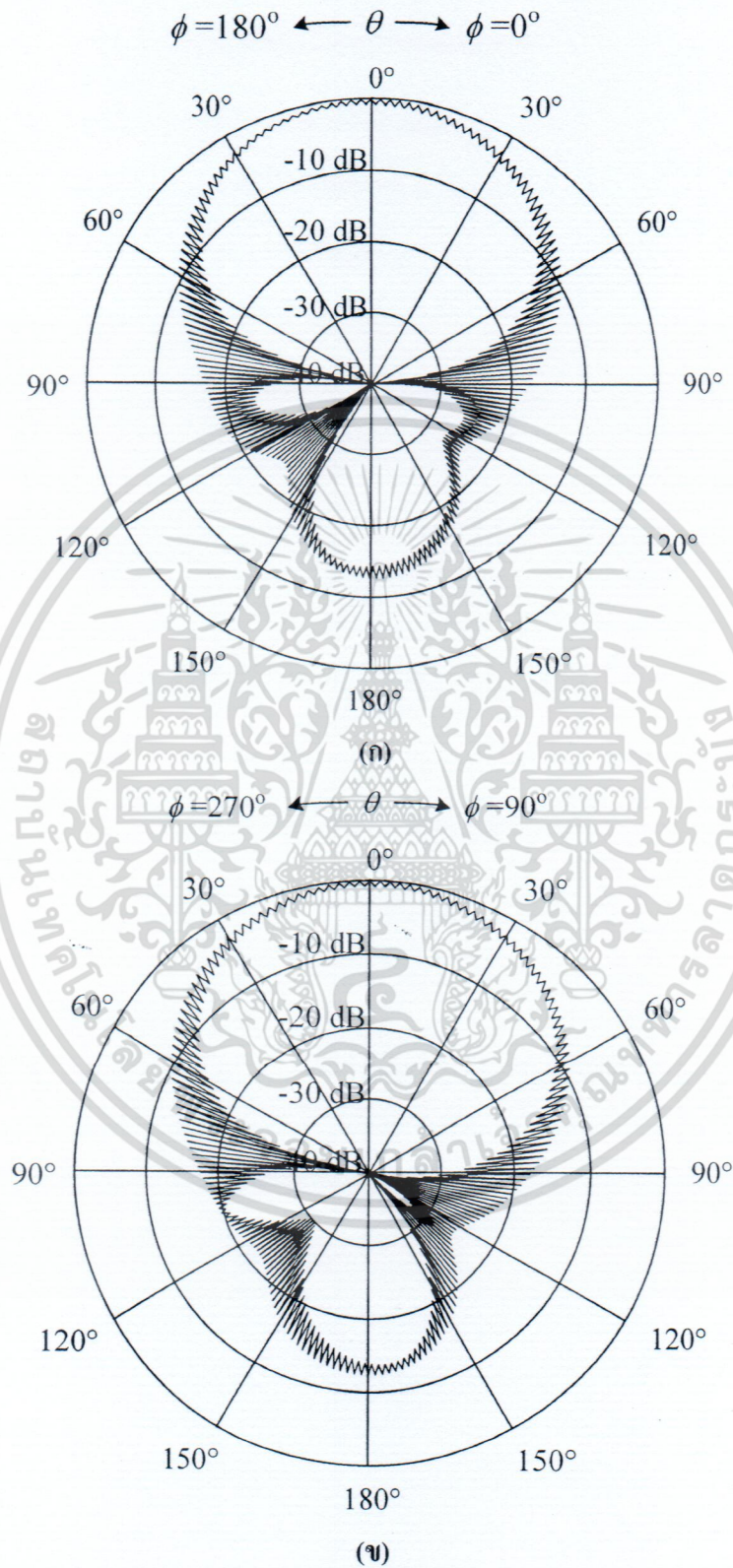
รูปที่ 3.21 แบบรูปการแพร่กระจายคลื่นอัตราส่วนแกนของสายอากาศ (ก)ระนาบ xz (ข)ระนาบ yz
