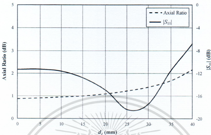
รูปที่ 3.12 อัตราส่วนแกนและ |S_{11}| เมื่อทำการเปลี่ยนแปลงความยาวของร่อง ( d_1 ) ของสายอากาศแผ่นระนาบสี่เหลี่ยมจัตุรัสตัดมุมแบบขึ้นร่วมกับร่องเฉียงคู่
