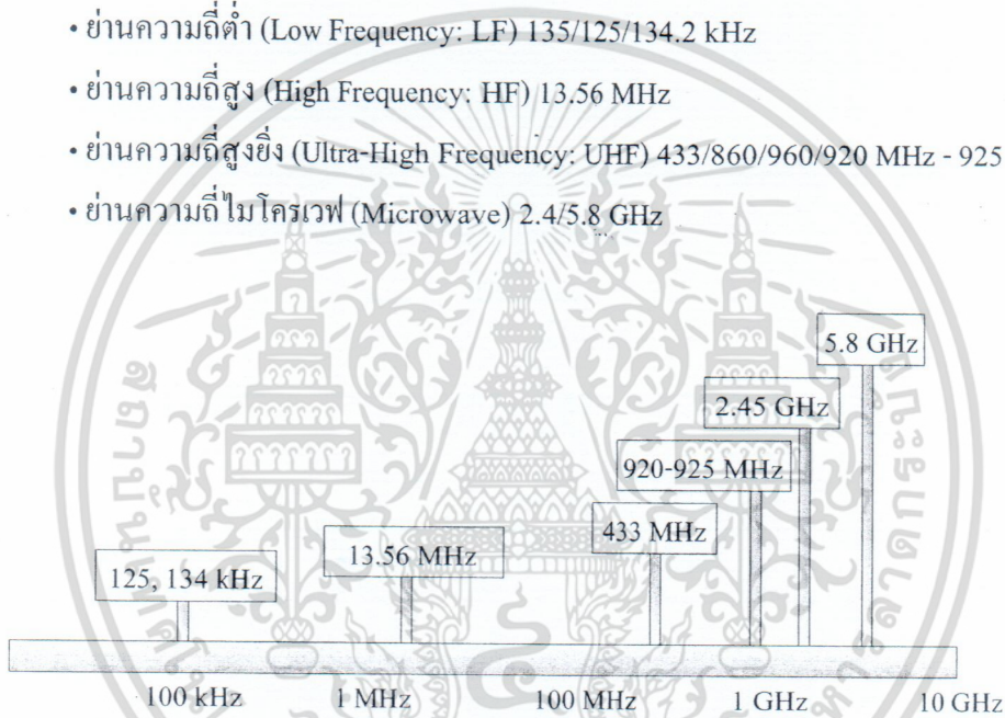
รูปที่ 2.15 ย่านความถี่ที่ใช้งานของระบบระบุลักษณะทางคลื่นความถี่วิทยุ [4]
