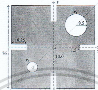
รูปที่ 2.21 สายอากาศไมโครสตริปวงกลมเจาะร่องวงกลมร่วมกับสลิต [25]
