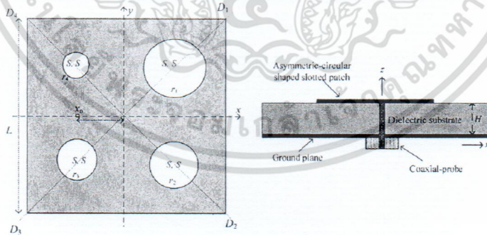
รูปที่ 2.20 สายอากาศไมโครสตริปเจาะร่องวงกลม [24]
