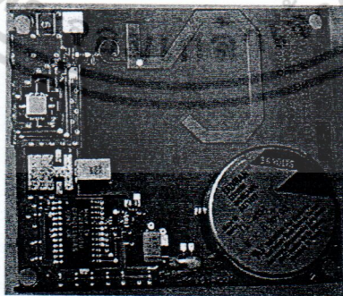
รูปที่ 2.4 แท้กของระบบระบุลักษณะทางคลื่นวิทยุแบบกึ่งแอดทีฟ [11]
