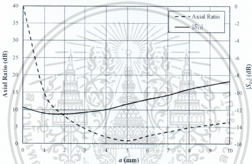
รูปที่ 3.10 อัตราส่วนแกนและค่า |S_{11}| เมื่อทำการเปลี่ยนแปลงความกว้าง ( a ) ของการตัดมุมแบบขั้น
