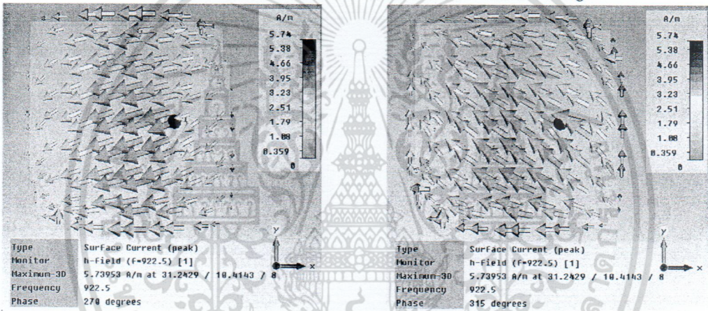
รูปที่ 3.10 กระแสที่ไหลบนแผ่นตัวแพร่กระจายคลื่นของสายอากาศแผ่นระนาบสี่เหลี่ยมจัตุรัสคดมุม
