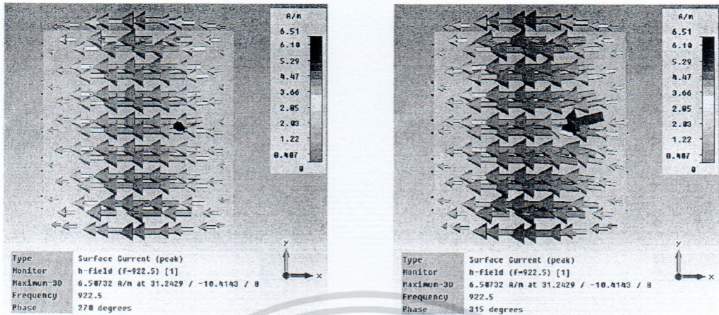
รูปที่ 3.7 กระแสที่ไหลบนผิวแผ่นตัวแพร่กระจายคลื่นของสายอากาศแผ่นระนาบสี่เหลี่ยมจัตุรัสที่เวลา ( t )
