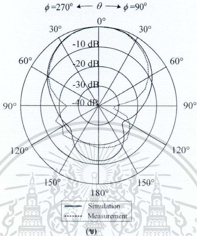
รูปที่ 4.15 เปรียบเทียบผลของแบบรูปการแพร่กระจายคลื่นที่ได้จากการทดสอบและการจำลอง
