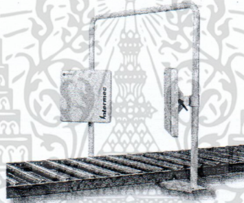
รูปที่ 2.16 สายอากาศเครื่องอ่านระบบระบุลักษณะทางคลื่นวิทยุที่ประยุกต์ใช้กับระบบสายพานลำเลียง [20]
