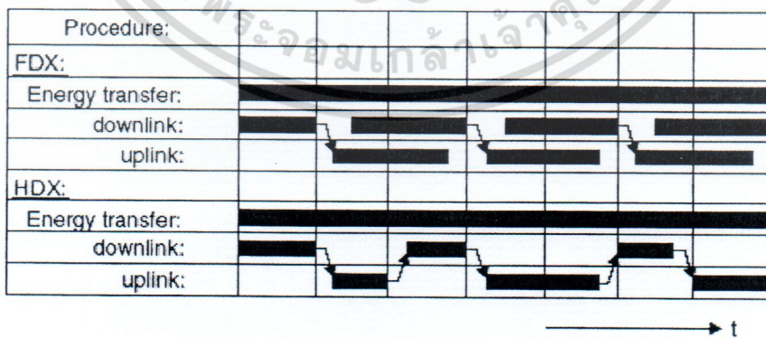
รูปที่ 2.14 ความแตกต่างของการสื่อสารแบบ Full duplex และ Half duplex [2]
