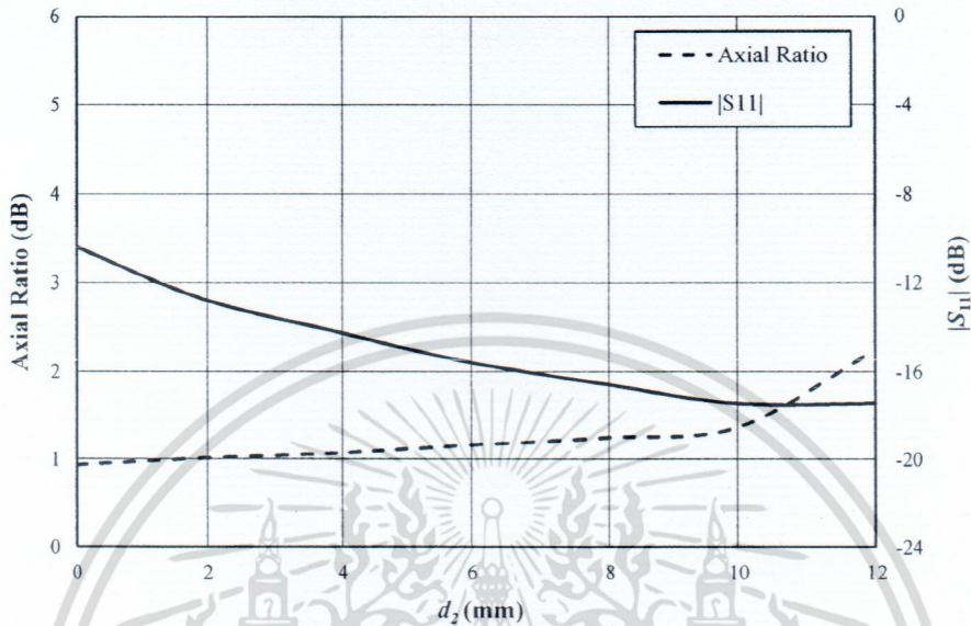
รูปที่ 3.13 อัตราส่วนแกนและ |S_{11}| เมื่อทำการเปลี่ยนแปลงความกว้างร่อง ( d_2 ) ของสายอากาศแผ่นระนาบสี่เหลี่ยมจัตุรัสคดมุมแบบขั้นร่วมกับร่องเอียงคู่
