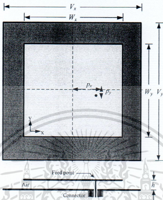
รูปที่ 3.3 โครงสร้างของสายอากาศแผ่นระนาบสี่เหลี่ยมจัตุรัส
