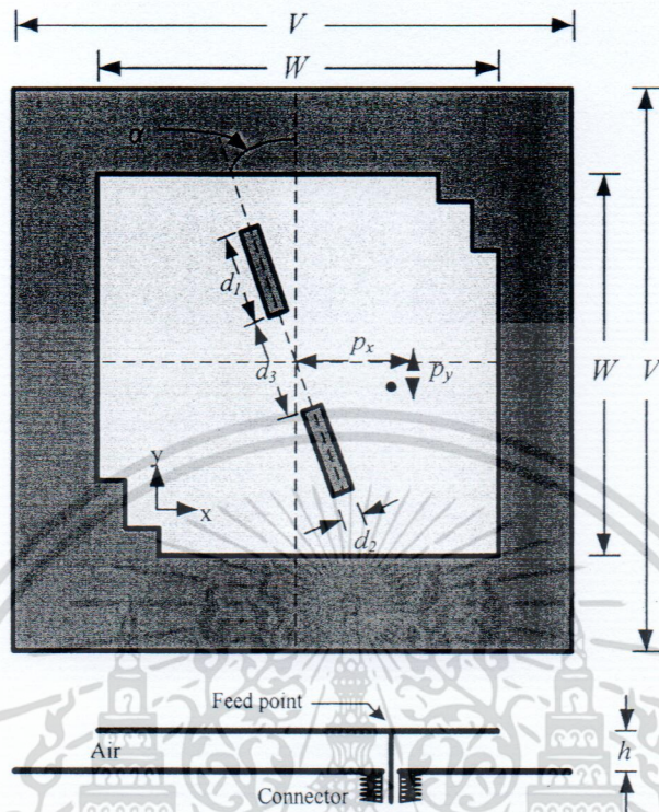
รูปที่ 3.11 โครงสร้างของสายอากาศแผ่นระนาบสี่เหลี่ยมจัตุรัสตัดมุมแบบขั้นร่วมกับร่องเอียงคู่
