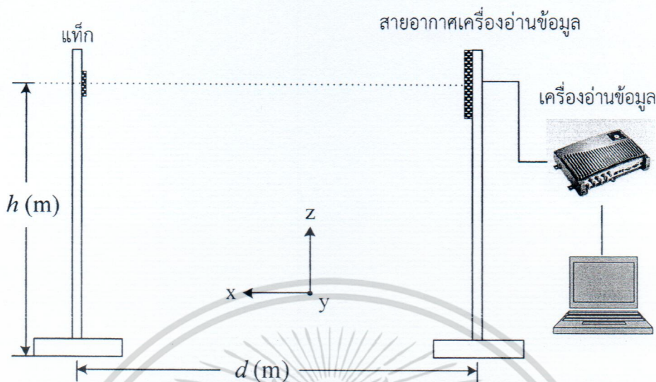
รูปที่ 5.4 การติดตั้งการทดสอบสายอากาศสำหรับเครื่องอ่านข้อมูลใช้งานร่วมกับแท่ง
