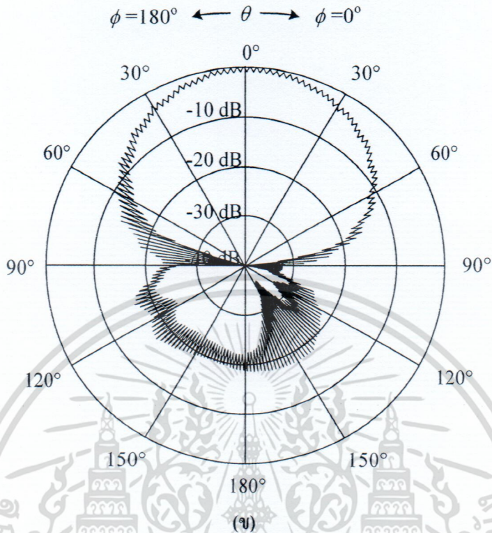
รูปที่ 4.6 แบบรูปการแพร่กระจายคลื่นอัตราส่วนแกนที่ได้จากการทดสอบ (ก)ระนาบ xz (ข)ระนาบ yz
