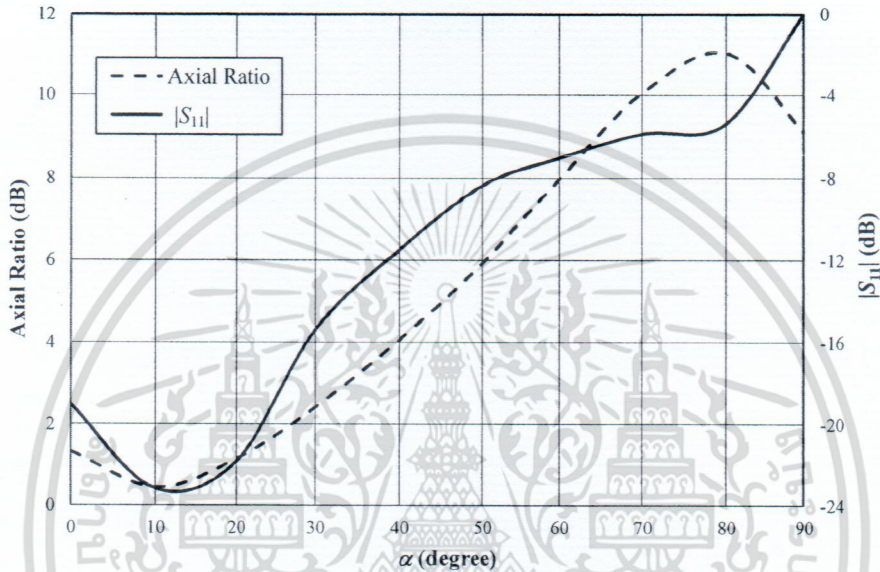
รูปที่ 3.15 อัตราส่วนแกนและ |S_{11}| เมื่อทำการเปลี่ยนแปลงมุมที่ร่องคู่ทำกับแนวแกน y ( \alpha ) ของสายอากาศแผ่นระนาบสี่เหลี่ยมจัตุรัสค้ำมุมแบบขั้นร่วมกับร่องเอียงคู่
