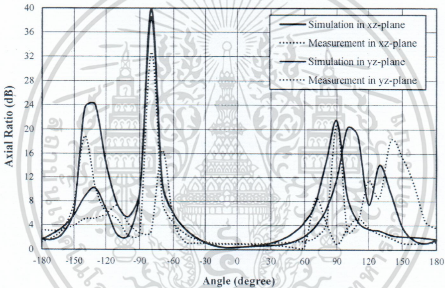
รูปที่ 4.14 เปรียบเทียบผลของอัตราส่วนแกนที่ความถี่กลาง (922.5 MHz) ของย่านความถี่ใช้งานที่ได้จากการทดสอบและการจำลอง
