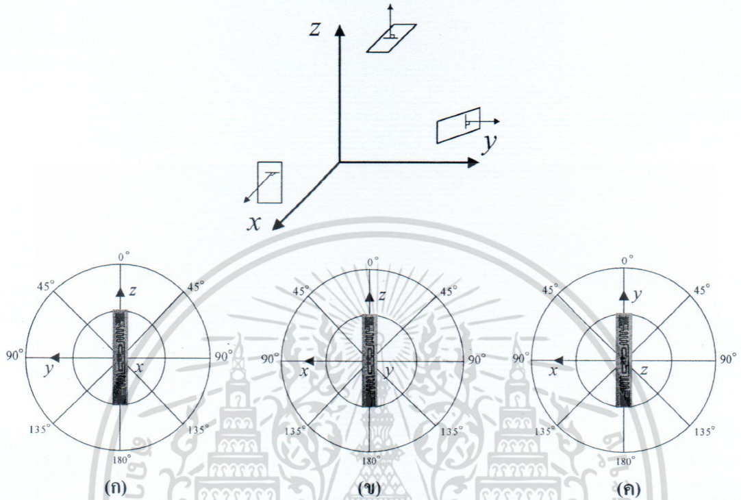
รูปที่ 5.5 การวางตัวของแท่งแต่ละแนวแกน (ก) แนวแกน x (ข) แนวแกน y (ค) แนวแกน z
