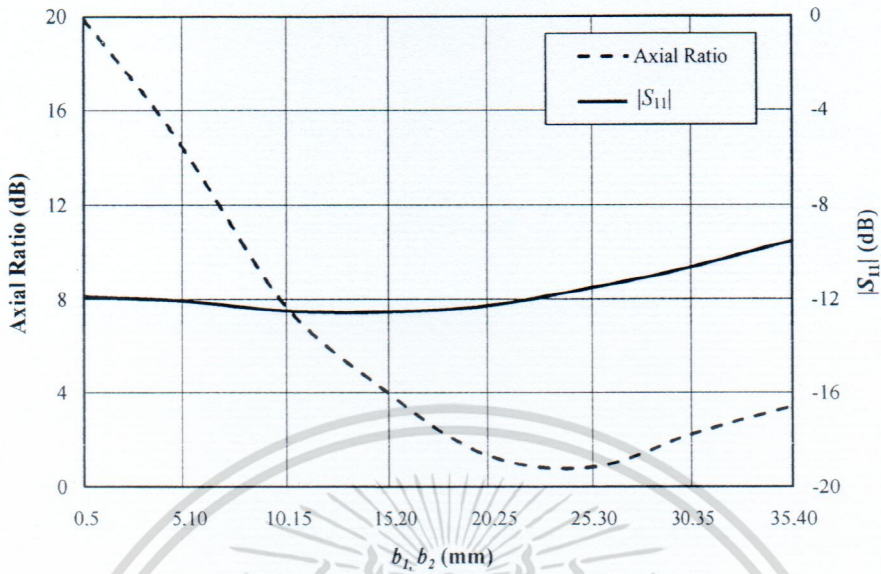
รูปที่ 3.9 อัตราส่วนแกนและ |S_{11}| เมื่อทำการเปลี่ยนแปลงความยาวของการตัดมุมแบบขั้นในแนวแกน x ( b_1 ) และ y ( b_2 )
