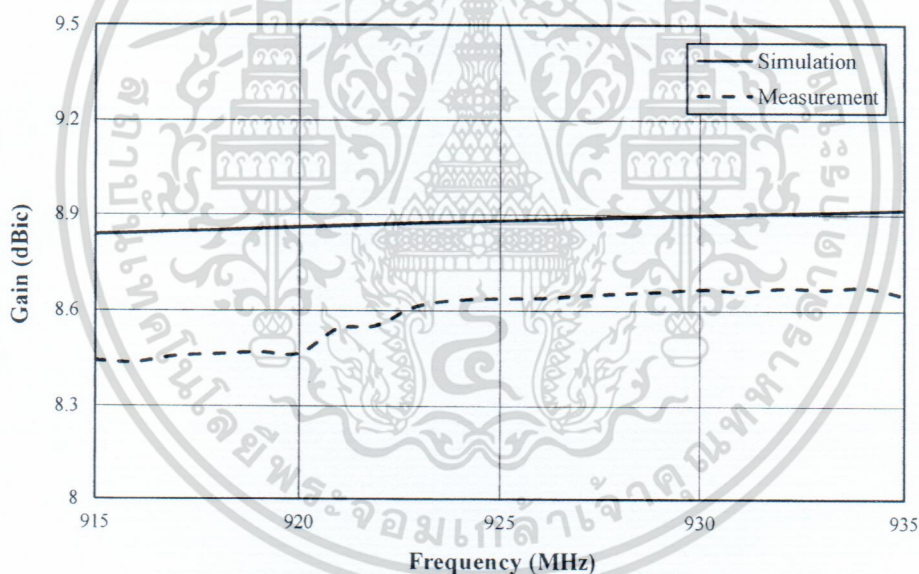
รูปที่ 4.13 เปรียบเทียบผลของอัตรายายที่ได้จากการทดสอบและการจำลอง
