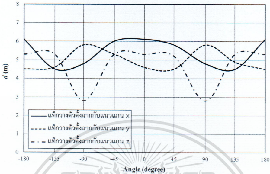
รูปที่ 5.6 ระยะในการติดต่อสื่อสารระหว่างเครื่องอ่านข้อมูลกับแท็กที่มุมต่างๆ เมื่อสายอากาศแผ่นระนาบสี่เหลี่ยมจัตุรัสตั้งมุมแบบขึ้นร่วมกับร่องเอียงคู่มือการ โพลาริซ์แบบวงกลมและแท็กวางตัวตั้งฉากกับแนวแกน x y และ z
