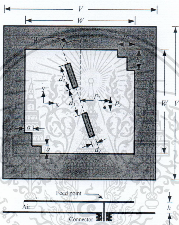
รูปที่ 3.2 โครงสร้างของสายอากาศแผ่นระนาบสี่เหลี่ยมจัตุรัสตัดมุมแบบขั้นร่วมกับร่องเฉียงคู่
