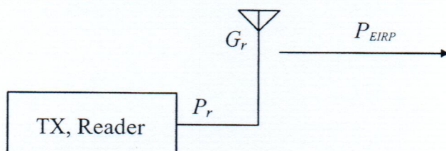
รูปที่ 2.25 กำลังงานการแพร่กระจายคลื่นประสิทธิภาพไอโซทรอปิก
