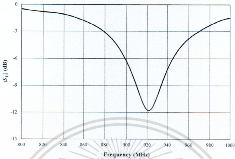
รูปที่ 3.5 |S_{11}| ของสายอากาศแผ่นระนาบสี่เหลี่ยมจัตุรัส
