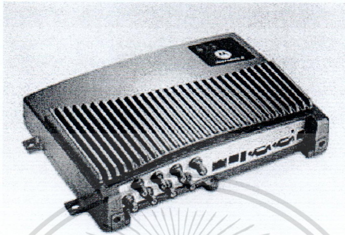
รูปที่ 5.16 เครื่องอ่านข้อมูลของระบบระบุลักษณะทางคลื่นวิทยุย่านความถี่สูงยิ่ง [29]
