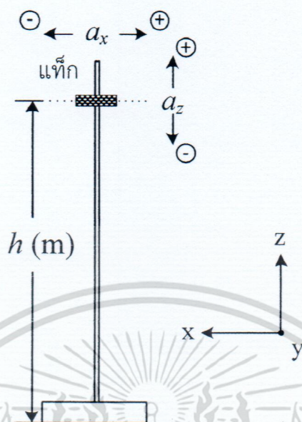
รูปที่ 5.7 การเปลี่ยนแปลงตำแหน่งความสูงในแนวแกน z ( a_z ) และ ตำแหน่งในแนวแกน x ( a_x ) ของสายอากาศแท่ง
