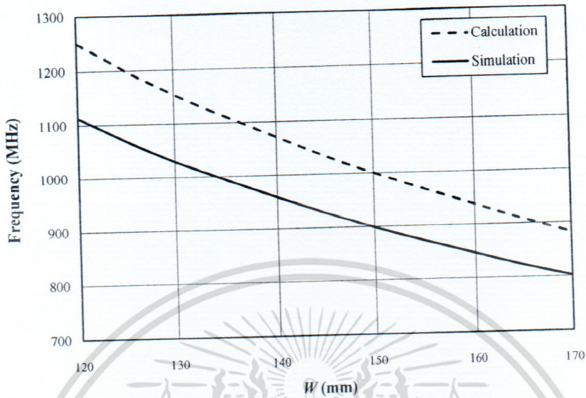
รูปที่ 3.4 ความสัมพันธ์ระหว่างขนาด ( W ) ของสายอากาศกับความถี่เรโซแนนซ์
