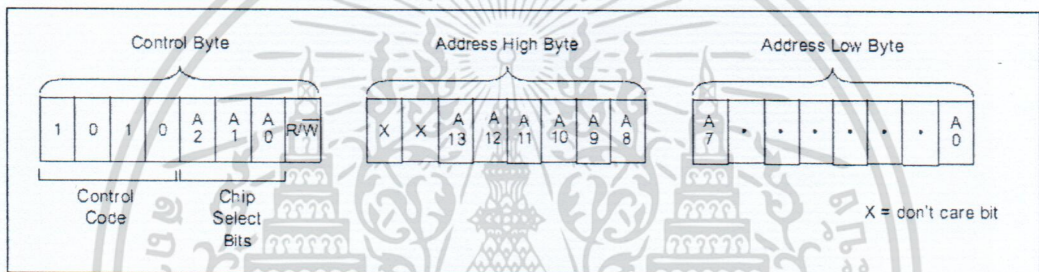
รูป 2.23 แอดเดรสของ Control Byte และ Address High Byte/Low Byte
