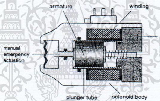
รูป 2.7 ขดลวดโซลินอยด์ชนิดเปียก (Wet solenoid)
