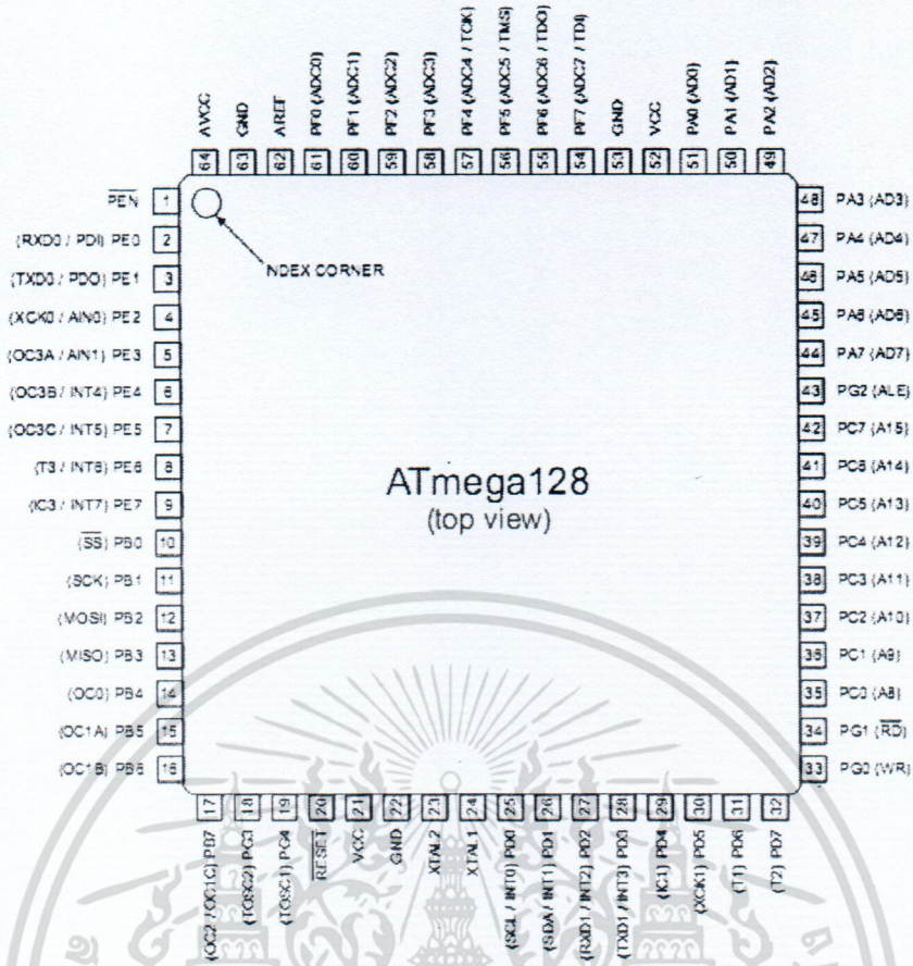
รูป 2.3 ขาพอร์ต AVR(ATmega128)
