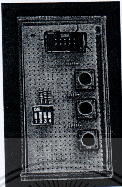
รูป 4.24 บอร์ดสำหรับการทำงานแบบไม่เชื่อมต่อกับคอมพิวเตอร์
