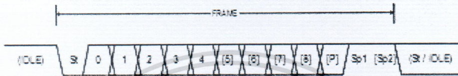
รูป 2.21 รูปแบบเฟรมข้อมูลในการส่งข้อมูลแบบ USART
