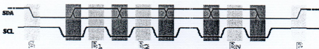
รูป 2.20 ไตอะแกรมเวลาแสดงสถานะต่างๆ ในบัส I 2 C
