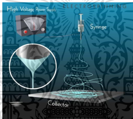
รูปที่ 4. วิธีการสังเคราะห์เส้นใยนาโนด้วยเทคนิคอิเล็กโตรสปินนิง [12]
