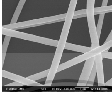
รูปที่ 5. แสดงโครงสร้างจุลภาคของเส้นใย (PZ/PPEO) ที่ได้จากระบวนการอิเล็กโตรสปินนิง
