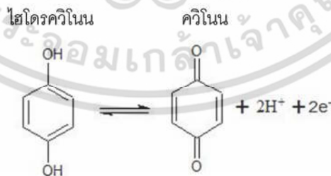
รูปที่ 5. ปฏิกิริยารีดอกซ์ของไฮโดรควิโนนบนขั้วไฟฟ้า
