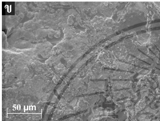
รูปที่ 6 ลักษณะทางกายภาพ (SEM) ของขี้เถ้าอะลูมิเนียม หลังจากการทดสอบวิธีกัลวานอสแตติกและปล่อยให้สารละลายแห้งอยู่บนพื้นผิว (ก) ใน NaOH และ (ข) สารละลายผสม (1:1)
