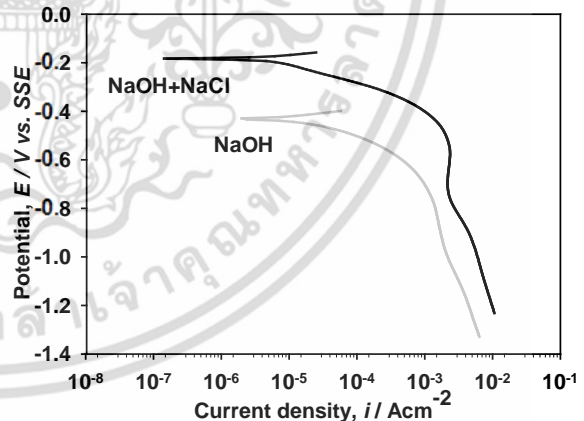
รูปที่ 3 แคโทดิกโพลาไรเซชันของขั้วอากาศในสารละลายผสม 1:1 (สีดำ) และ NaOH (สีเทา)
