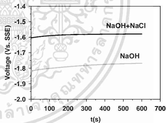
รูปที่ 1 ศักย์ไฟฟ้าวงจรถัดของขั้วอะลูมิเนียมในสารละลายผสม 1:1 (สีดำ) และ NaOH (สีเทา)
